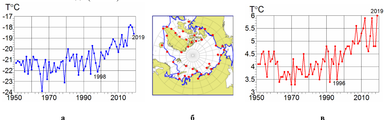
Рисунок 5.6 – Средняя за декабрь-февраль (а) и за июнь-август (в) приповерхностная температура воздуха на 41 станции в морской Арктике (б) в 1951–2019 гг.
