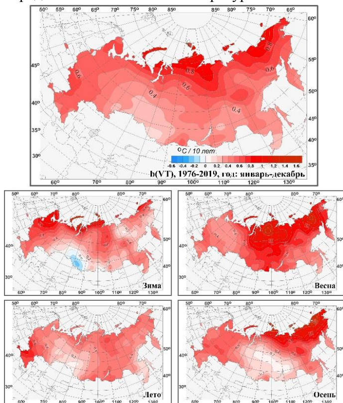
Рисунок 1.6 – Коэффициент линейного тренда среднегодовой и средних сезонных значений температуры приземного воздуха на территории России за период 1976-2019 гг. ( ^{\circ}\text{C}/10 \text{ лет} )
