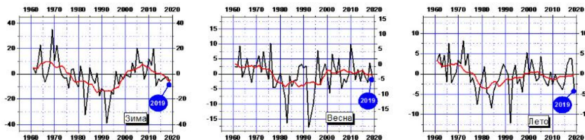
Рисунок 9.6 - Аномалии (в процентах от среднего за 1961-1990 гг.) сезонных сумм прямой радиации, поступающей на горизонтальную поверхность, осредненные по территории РФ. 1961-2019гг.
