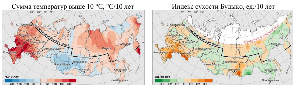
Рисунок 7.2 – Скорость изменения (линейный тренд) суммы активных температур выше 10 °C и индекса сухости Будыко (ИС) на территории России за 2000–2019 гг.
