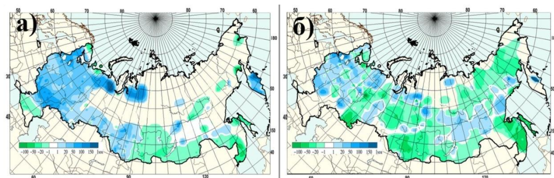
Рисунок 3.3 - Аномалии максимального запаса воды в снеге (мм) зимой 2018-2019 гг. (от среднееголетних значений за период 1971-2000 гг.) в поле (а) и в лесу (б).
