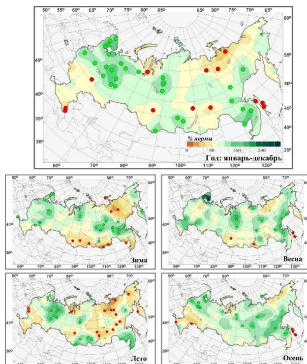
Рисунок 2.2 – Аномалии осадков на территории России в 2019 г. с указанием локализации 5%-х экстремумов (красные кружки) и 95%-х (зеленые кружки)
