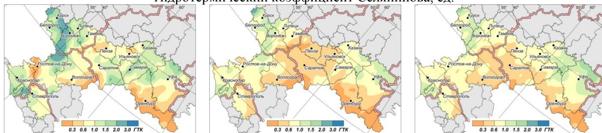
Рисунок 7.1 – Мониторинг условий увлажнённости вегетационного периода 2019 г.: сумма осадков в % относительно средних значений за 2009–2018 гг. и гидротермический коэффициент Селянинова (ГТК) на 20 мая, 20 июня и 20 июля 2019 г.
