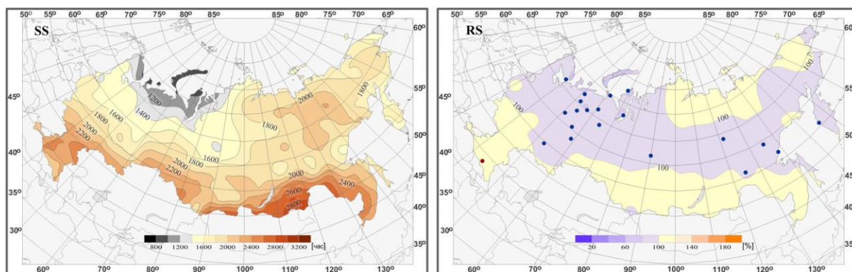
Рисунок 10.1 – Пространственное распределение суммарной за год продолжительности солнечного сияния (SS, часы) и ее относительных аномалий (RS, %) на территории РФ в 2019 г. (январь – декабрь). Кружками синего цвета показано местоположение станций с экстремумами ниже 5-го перцентиля, коричневого цвета – выше 95-го перцентиля
