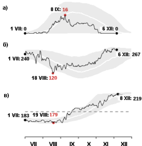
Рисунок 14.3 - Основные характеристики весенней Антарктической озоновой аномалии 2019 г.: площадь, с ОСО меньше 220 ед. Д. (млн. км 2 , а), минимальное ОСО (ед. Д., б) и минимальная температура в стратосфере (К, в). Серым цветом отмечены области между минимальными и максимальными величинами, наблюдаемыми в 1979-2018 гг.; светлые линии внутри этих областей – средние за этот период.
