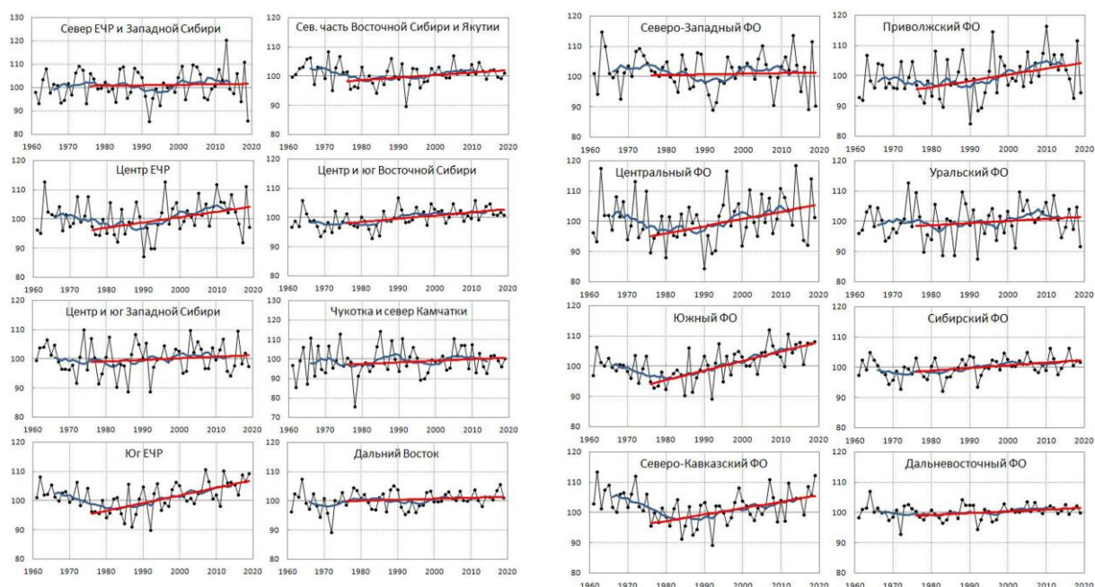
Рисунок 10.8 – Относительные аномалии (%) суммарной за год продолжительности солнечного сияния, осредненные по физико-географическим регионам и по федеральным округам РФ
