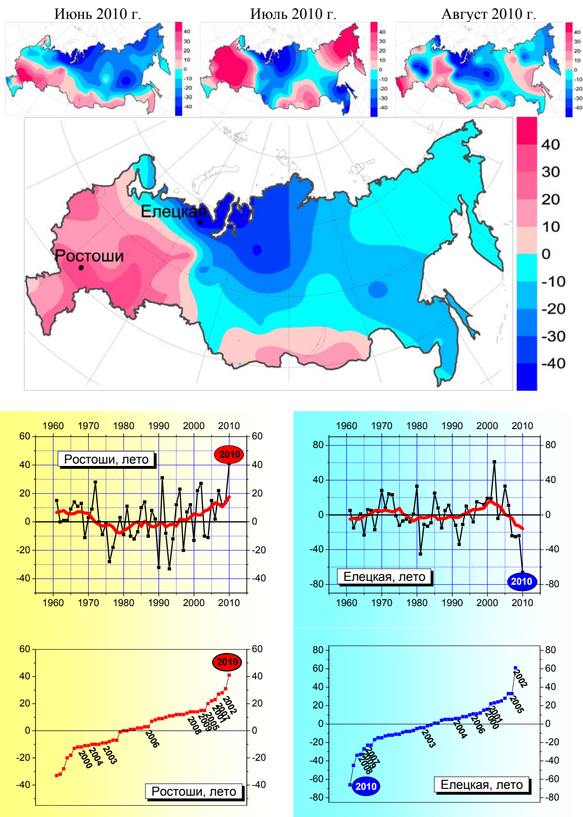
Рисунок 9.5 – Аномалии (в процентах от среднего за 1961-90 гг.) месячных и сезонных сумм прямой солнечной радиации. Лето 2010 г.
