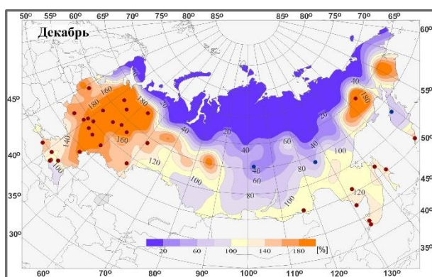
Рисунок 10.3 – Пространственное распределение относительных аномалий продолжительности солнечного сияния ( RS , %) на территории РФ в декабре 2020 г. Кругами синего цвета показано местоположение станций с экстремумами ниже 5-го процентиля, коричневого цвета – выше 95-го процентиля.
