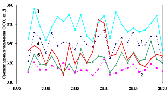
Рисунок 16.3 - Межгодовая изменчивость среднегодовых значений ОСО в интервалах широт 60°-90° с.ш. (1), 30°-60° с.ш. (2) и на станциях Якутск (3, 62° с.ш., 130° в.д.), Екатеринбург (4, 57° с.ш., 61° в.д.) и С.-Петербург (5, 60° с.ш., 30° в.д.)
