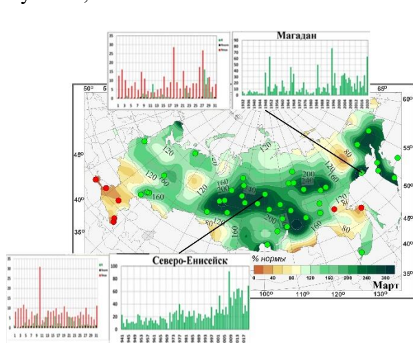
Рисунок 2.3 – Аномалии осадков в марте.
