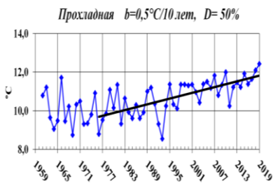
Рисунок 1.7 - Среднегодовой ход температуры на мс с линейным трендом за период 1976-2019 гг.; b - значение углового коэффициента линейного тренда, ^{\circ}\text{C}/10 лет; D (%) - вклад тренда в суммарную дисперсию.
