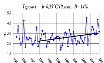
Рисунок 1.7 - Среднегодовой ход температуры на мс с линейным трендом за период 1976-2019 гг.; b - значение углового коэффициента линейного тренда, ^{\circ}\text{C}/10 лет; D (%) - вклад тренда в суммарную дисперсию.
