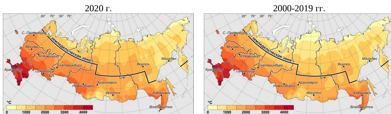
Рисунок 7.1 – Сумма температур выше 10^{\circ}\text{C} ( ^{\circ}\text{C} ) за 2020 г. и средние значения за 2000–2019 гг.
