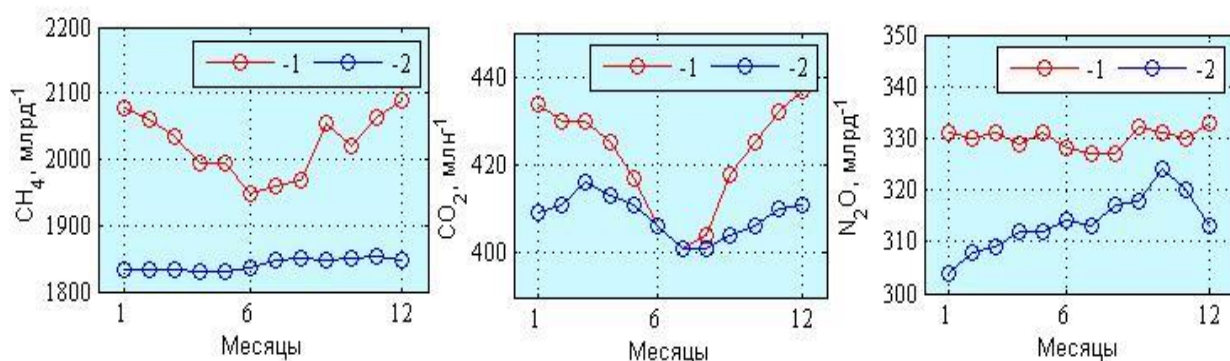
Рисунок 14.5 – Приземные (1) и средние по высоте (2) концентрации \text{CH}_4 , \text{CO}_2 , \text{N}_2\text{O} за 2015-2020 гг.
