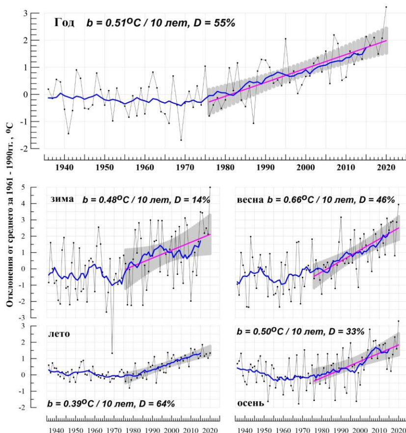
Рисунок 1.1 – Средние годовые (вверху) и сезонные аномалии температуры приземного воздуха (°C), осредненные по территории России, 1936-2020 гг.
