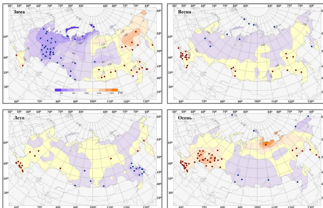
Рисунок 10.2 – Пространственное распределение относительных аномалий сезонной продолжительности солнечного сияния (RS, %) на территории РФ в 2020 г. Кругжками синего цвета показано местоположение станций с экстремумами ниже 5-го перцентиля, коричневого цвета – выше 95-го перцентиля.
