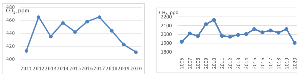
Рисунок 14.6 - Изменения среднегодовых концентраций \text{CO}_2 и \text{CH}_4 в приземном слое атмосферы на станции ПТБЗ.
