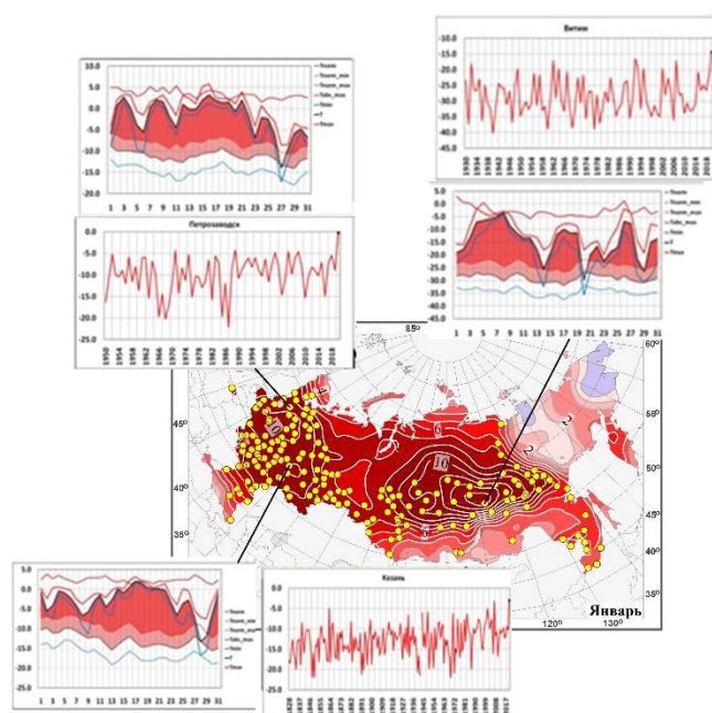
Рисунок 1.3 – Аномалии температуры приземного воздуха на территории России в январе
