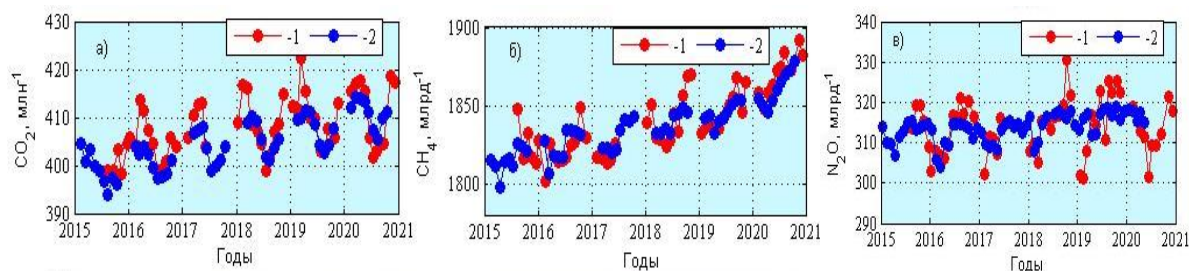
Рисунок 14.4 – Средняя по высоте объемная концентрация \text{CO}_2 (а), \text{CH}_4 (б), \text{N}_2\text{O} (в). 1 – ст. «Обнинск», 2 – спутниковые данные GOSAT ( \text{CO}_2 и \text{CH}_4 ) и данные ст. Карлсруэ ( \text{N}_2\text{O} ).
