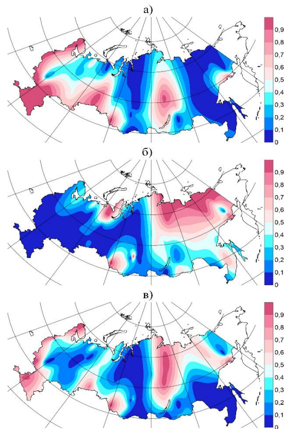
Рисунок 9.7 – Вероятности превышения сезонных сумм прямой солнечной (а), рассеянной (б) и суммарной (в) радиации. Лето 2020 г.
