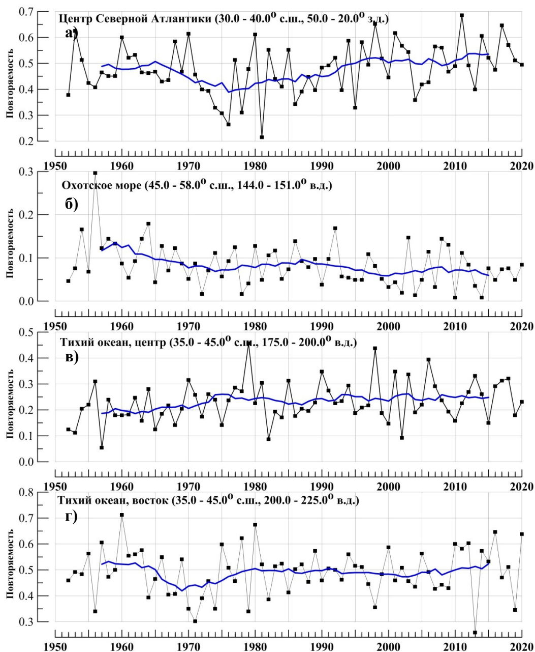
Рисунок 10 - Повторяемость антициклонов летом 2020 года для регионов Северной Атлантики и северной части Тихого океана
