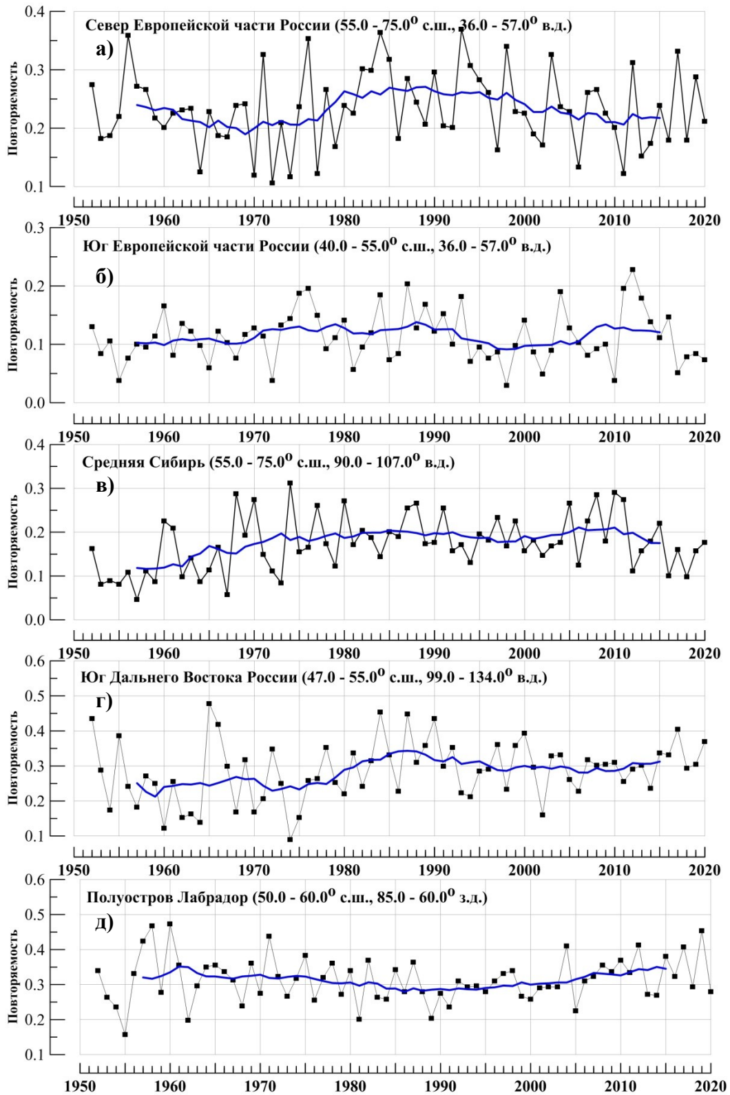
Рисунок 9 - Повторяемость циклонов в континентальных регионах северной Евразии и Северной Америки для летнего сезона 2020 года
