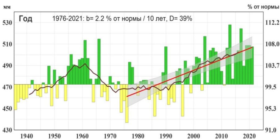
Рис. 1.2. Средние годовые суммы осадков (мм) осредненные по территории РФ, 1936-2021 гг.
