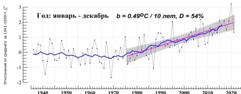
Рис. 1.1. Средние годовые аномалии температуры приземного воздуха ( ^{\circ}\text{C} ), осредненные по территории РФ, 1936-2021 гг.
