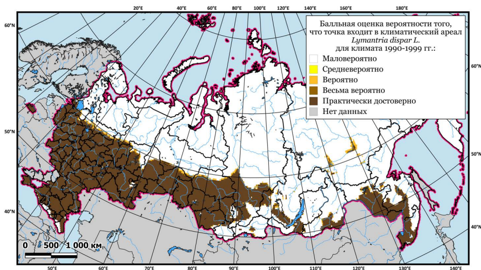
Рисунок 3. Балльная оценка вероятности того, что точка входит в климатический ареал L. dispar на территории России, соответствующий климату КЦР а для 1990-1999 гг.
