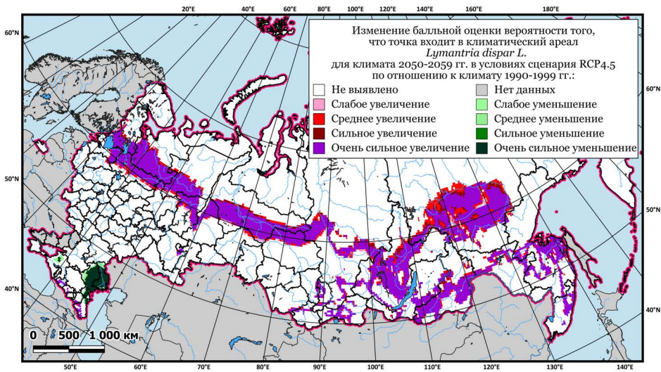
Рисунок 5. Изменение балльной оценки вероятности того, что точка географического пространства входит в климатический ареал L. dispar , соответствующий климату КЦР a для 2050-2059 гг. по сравнению с климатом 1990-1999 гг. в условиях сценария RCP4.5
