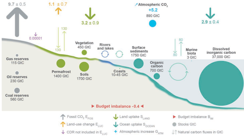
Рисунок 1. Диаграмма распределения запасов углерода в атмосфере, гидросфере, биосфере и литосфере, а также средних (за период с 2014 по 2023 годы) изменений поглощения \text{CO}_2 сушей и океаном (зеленые и голубые стрелки, соответственно) и накопление \text{CO}_2 в атмосфере вследствие выбросов \text{CO}_2 в атмосферу от антропогенных источников (серая стрелка). Потоки \text{CO}_2 обозначены стрелками. Компоненты бюджета \text{CO}_2 включают независимые оценки антропогенных выбросов \text{CO}_2 в результате (1) сжигания и окисления ископаемого топлива в процессе энергетических и промышленных процессов, включая производство цемента и карбонизацию ( E_{\text{FOS}} ; \text{GtC}/\text{год} ), и (2) антропогенной деятельности, приводящей к изменению структуры землепользования ( E_{\text{LUC}} ; \text{GtC}/\text{год} ), а также их распределение между накоплением \text{CO}_2 в атмосфере ( G_{\text{ATM}} ; \text{GtC}/\text{год} ) и поглощением \text{CO}_2 в (4) океане ( S_{\text{OCEAN}} ; \text{GtC}/\text{год} ) и (5) на суше ( S_{\text{LAND}} ; \text{GtC}/\text{год} ). Поглотители \text{CO}_2 , представленные на рисунке, концептуально включают реакцию суши (с учётом внутренних вод и эстуариев) и океана (включая окраинные моря) на повышенный уровень \text{CO}_2 , изменения климата и других условий окружающей среды. Потоки выражены в \text{GtC}/\text{год} , а резервуары углерода – в \text{GtC} (Friedlingstein et al., 2025)
