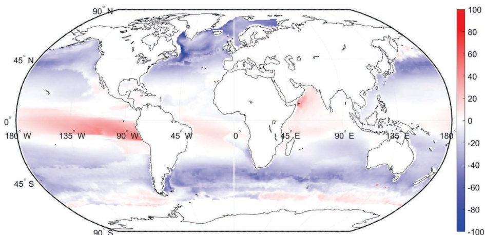
Рисунок 3. Оценка суммарного годового потока \text{CO}_2 ( \text{гC/м}^2\text{год} ) для поверхности мирового океана в 2023 году, полученная с использованием данных по концентрации растворенного \text{CO}_2 в воде ( \text{pCO}_2 ), концентрации \text{CO}_2 в воздухе и скорости ветра у поверхности океана, для регулярной сетки 1^\circ \times 1^\circ (Iida, et al., 2021) и доступная на платформе Japan Meteorological Agency, JMA [ https://www.data.jma.go.jp/kaiyou/english/co2_flux/co2_flux_data_en.html ]. Карта построена А.О. Масляшовой
