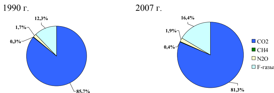
Рис. III. 5 Доля отдельных парниковых газов в их общем выбросе (CO 2 -экв.), связанном с промышленными процессами, использованием растворителей и другой продукции в 1990 и 2007 гг.
