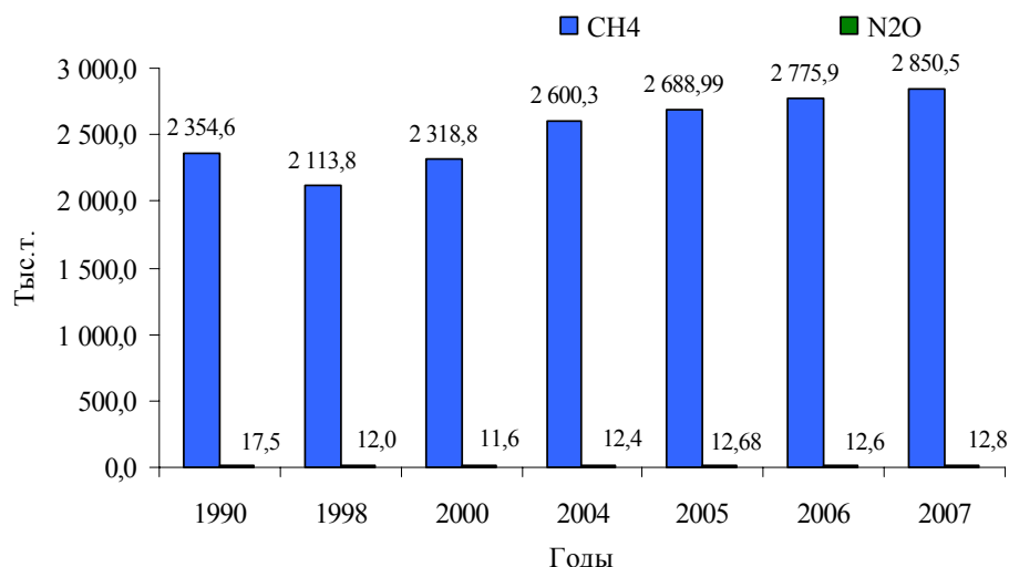
Рис. III.11 Динамика выбросов метана и закиси азота в секторе обращения с отходами
