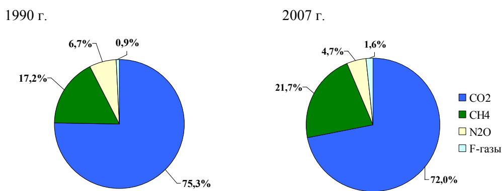
Рис. 1. 3. Доля отдельных парниковых газов в их общем выбросе (CO 2 -экв.) в 1990 и 2007 гг. (без учета сектора «Землепользование, изменение землепользования и лесное хозяйство»)
