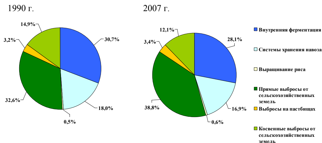
Рис. III.7 Доля отдельных источников в общем выбросе парниковых газов (CO 2 -экв.) в сельскохозяйственном секторе в 1990 и 2007 гг.
