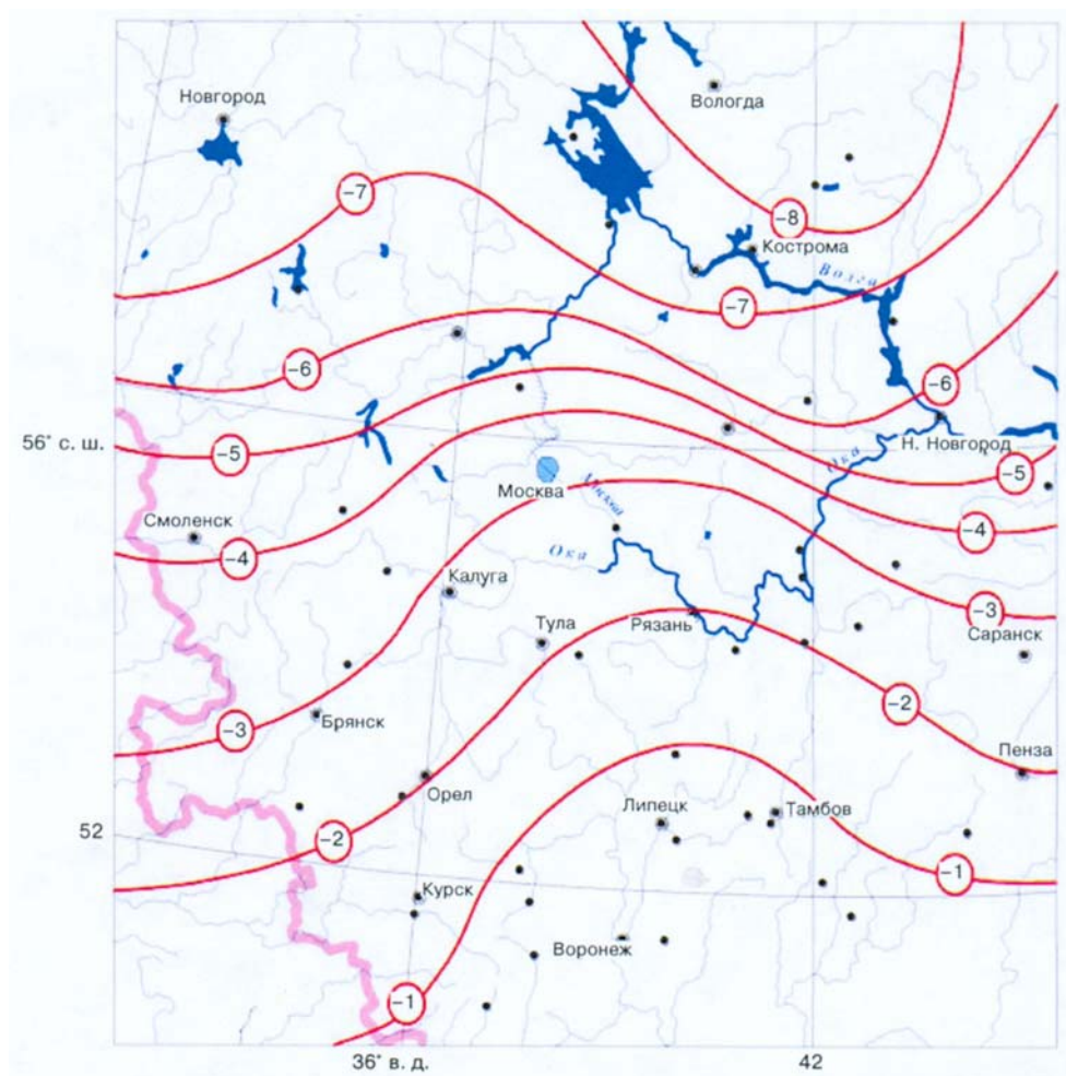
Рис. VI. 1. Изолинии сдвига сроков разворачивания первых листьев у березы бородавчатой на ЕТР за период 1970-2000 гг., сутки; точками показаны пункты фенологических наблюдений
