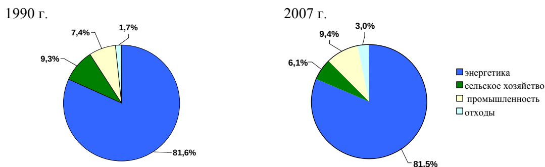
Рис. 1. 2. Распределение общего выброса парниковых газов (CO 2 -экв.) по секторам в 1990 и 2007 гг.
