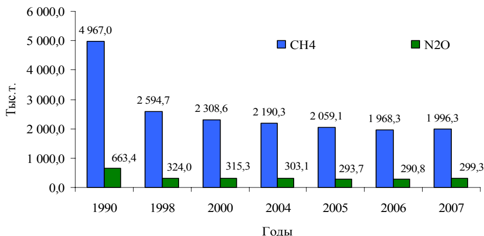
Рис. III.6 Выбросы метана и закиси азота в сельскохозяйственном секторе в 1990-2007гг.
