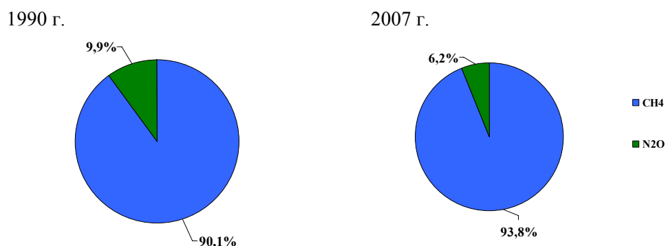
Рис. III.13 Доля отдельных парниковых газов в их общем выбросе ( CO_2 -экв.) в секторе обращения с отходами в 1990 и 2007 годах
