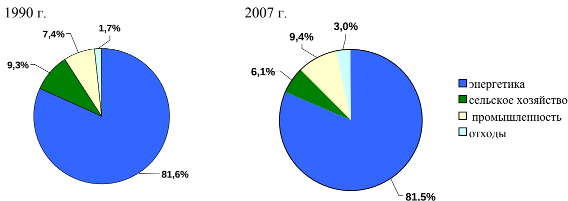
Рис. III. 2. Распределение общего выброса парниковых газов (CO 2 -экв.) по секторам в 1990 и 2007 гг.
