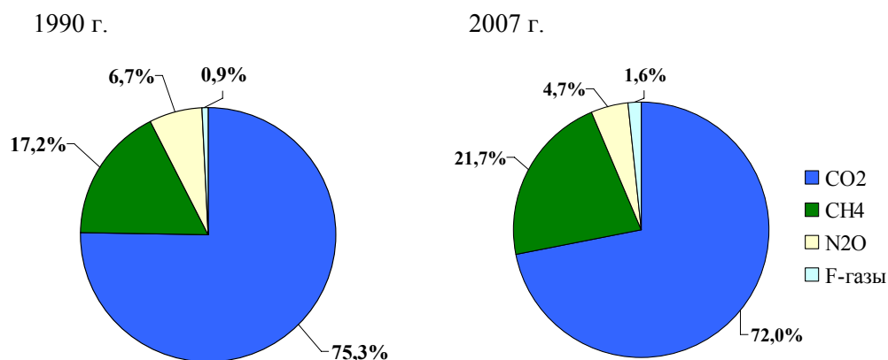
Рис. III. 3. Доля отдельных парниковых газов в их общем выбросе (CO 2 -экв.) в 1990 и 2007 гг. (без учета сектора «Землепользование, изменение землепользования и лесное хозяйство»)
