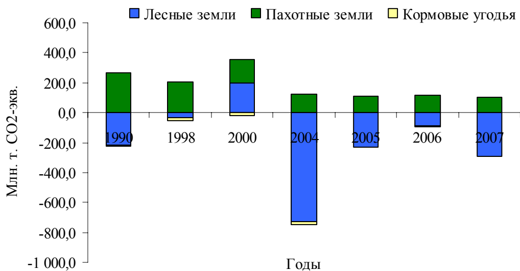
Рис. III.10 Выбросы (+) и поглощение (-) парниковых газов при землепользовании и в лесном хозяйстве в 1990, 1998, 2000 и 2004-2007 гг.
