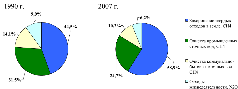
Рис. III.12 Доля отдельных источников в общем выбросе парниковых газов ( CO_2 -экв.) в секторе обращения с отходами в 1990 и 2007 годах
