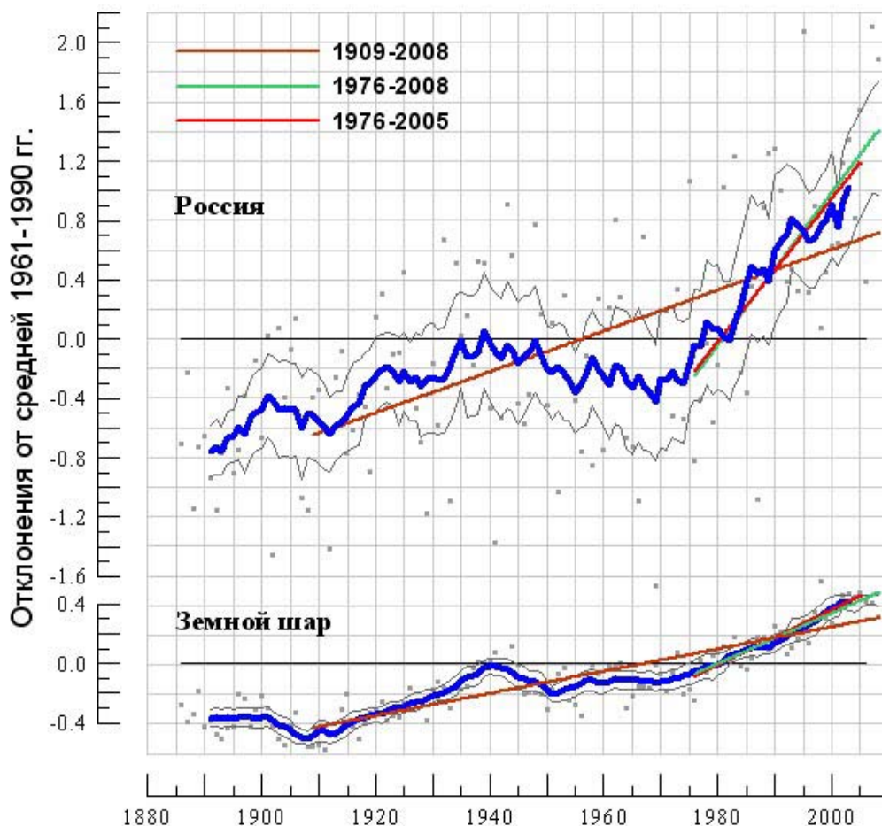
Рис. I.5. Изменения среднегодовой температуры приземного воздуха, осредненной по территории России (вверху), и средней приповерхностной температуры Земного шара (внизу) в отклонениях от средних за 1961-1990 гг. Точками показаны результаты наблюдений, кривыми – 11-летняя сглаженная и 95% доверительный интервал сглаженных значений. Линейные тренды проведены за периоды: 1909-2008, 1976-2005 и 1976-2008 гг.
