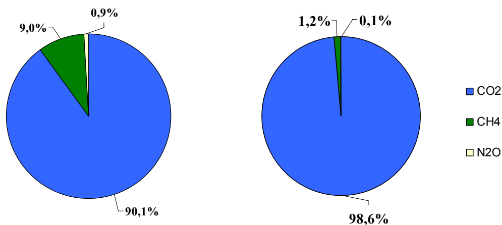
Рис. III.9 Доля отдельных парниковых газов в общем выбросе ( \text{CO}_2 -экв.) от землепользования, изменений в землепользовании и лесном хозяйстве в 1990 и 2007 годах.
