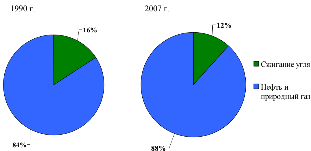
Рис. III.4 Доля отдельных источников в общем выбросе парниковых газов (CO 2 -экв.), связанном с технологическими выбросами и утечками в 1990 и 2007 гг.
