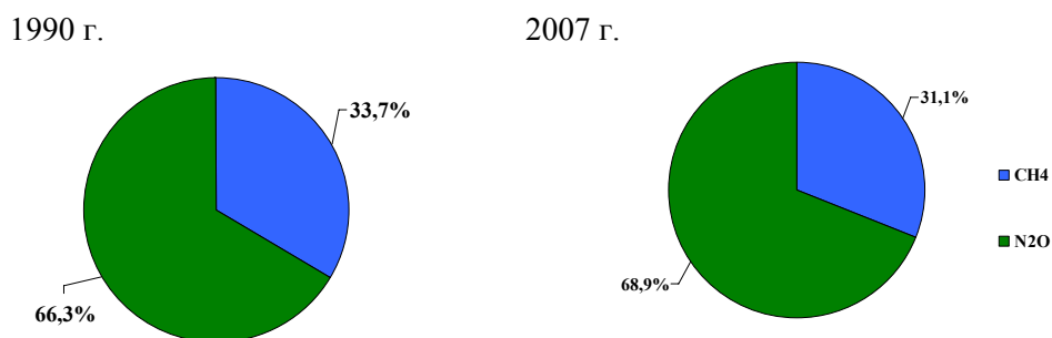
Рис. III.8 Доля отдельных парниковых газов в их общем выбросе (CO 2 -экв.) в сельскохозяйственном секторе в 1990 и 2007 гг.
