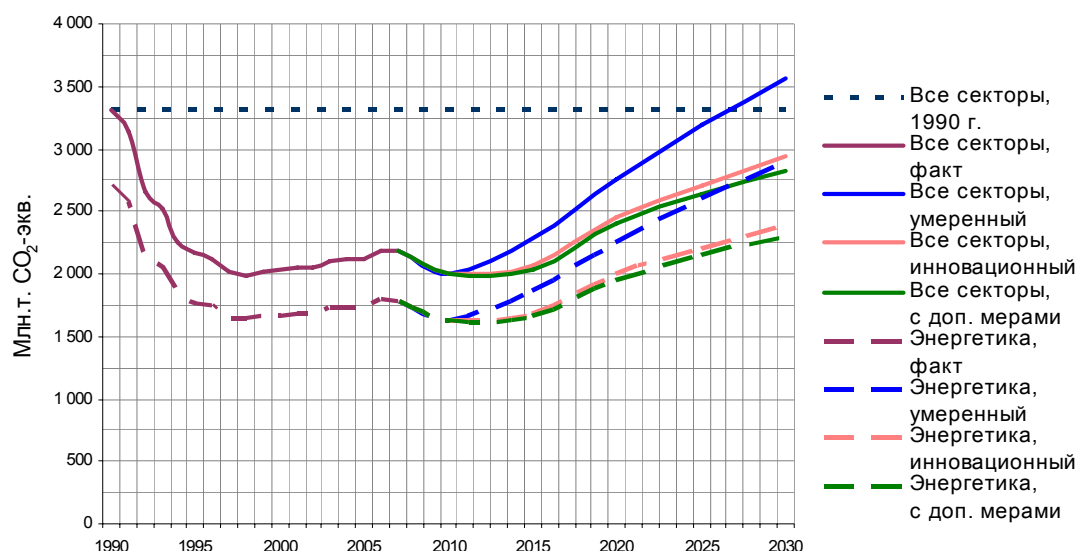
Рис. 1.4. Сценарии совокупного выброса парниковых газов и выброса парниковых газов в энергетическом секторе Российской Федерации до 2030 г.
