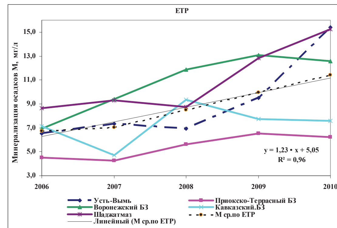
Рис. 4.4. Ход изменения со временем минерализации осадков по отдельным станциям и средней суммы ионов ( M_{\text{ср.}} ) на ЕТР за период 2006–2010 гг.
