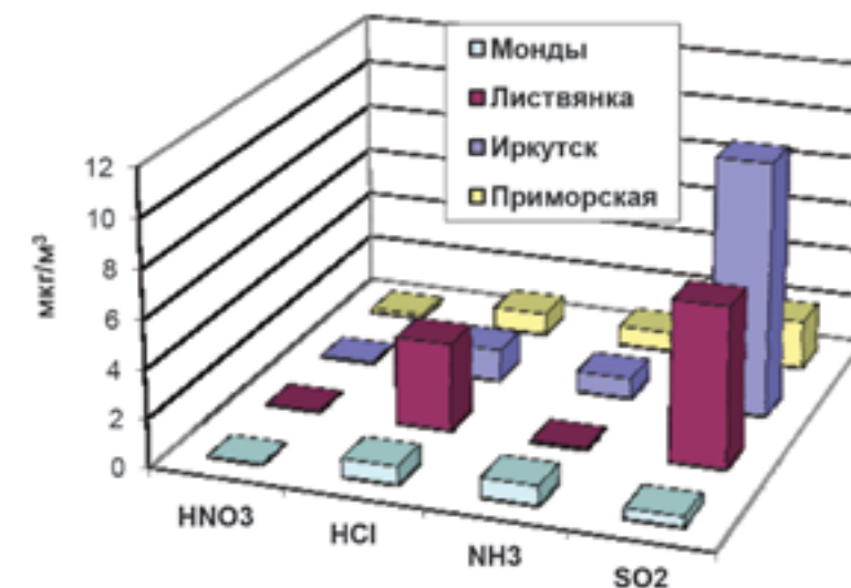
Рис. 1.4.1. Среднегодовое содержание газовых примесей в воздухе по данным измерений на станциях ЕАНЕТ в 2012 г. (мкг/м³)
