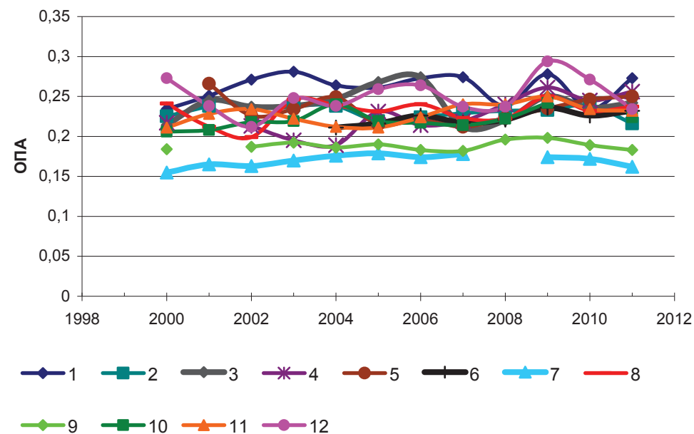
Рис. 1.2.3.5. Изменение среднегодовых значений ОПА на северных и арктических станциях (1 – Бутрино, 2 – о. Врангеля, 3 – Елецкая, 4 – Оленек, 5 – Сеяха, 6 – Уэлен), на антарктической станции 7 – obs. Мирный и на фоновых станциях (8 – Памятная, 9 – Шаджатмаз, 10 – Туруханск, 11 – Хужир, 12 – Усть-Вымь)
