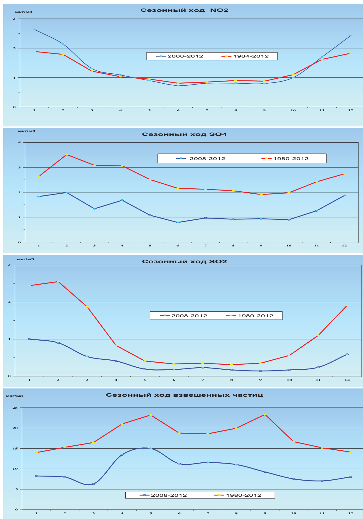
Рис. 5.2. Сезонный ход фоновых концентраций загрязняющих веществ в атмосферном воздухе Бerezинского БЗ
