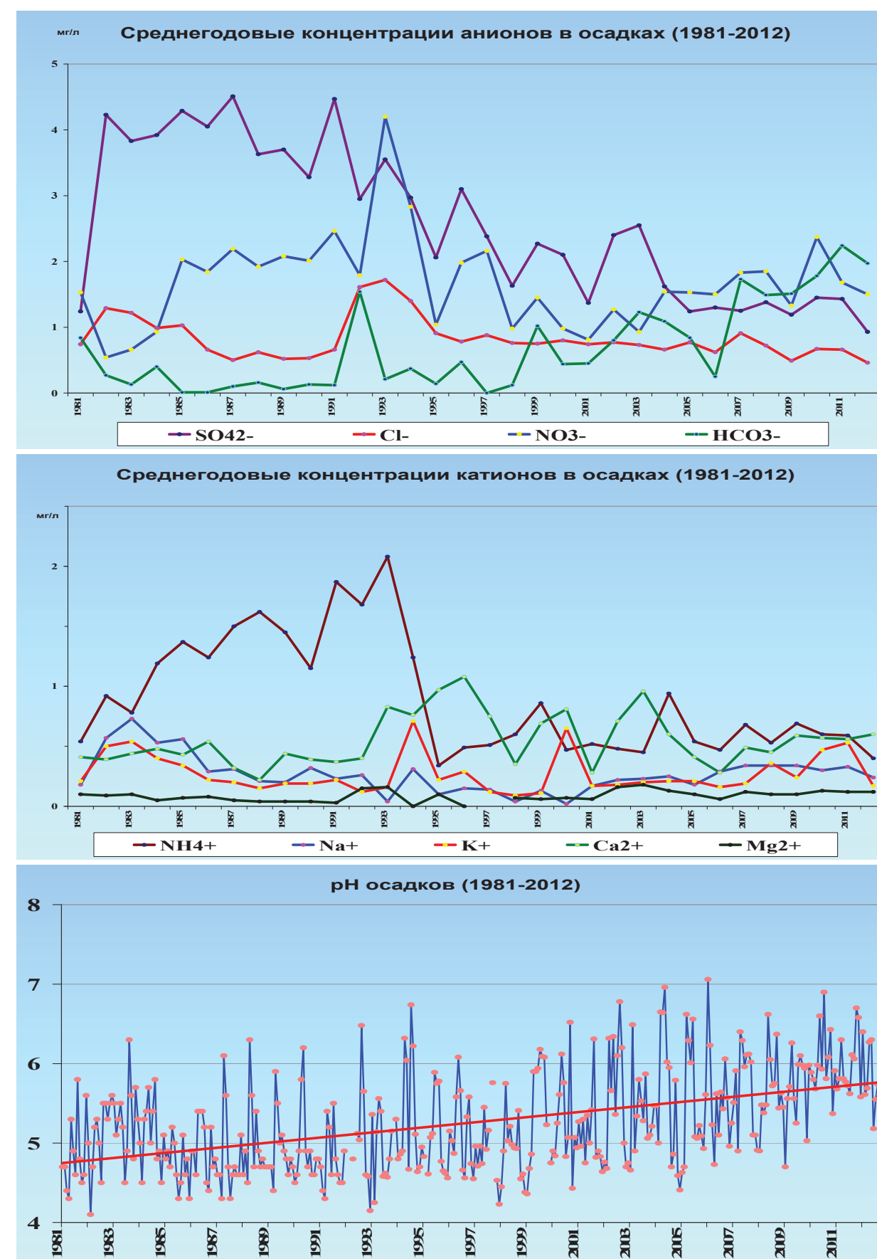
Рис. 5.3. Среднегодовые концентрации основных ионов и динамика pH в атмосферных осадках Бerezинского БЗ
