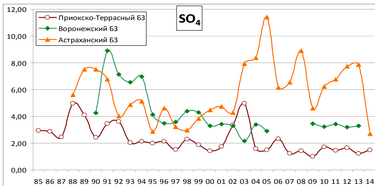
Рис. 1.1.3. Изменение фоновое содержание диоксида серы, диоксида азота и сульфатов в атмосферном воздухе фоновых районов (мкг/м³).
