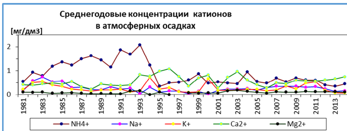
Рис. 5.3. Среднегодовые концентрации основных ионов и динамика pH в атмосферных осадках Березинского БЗ.
