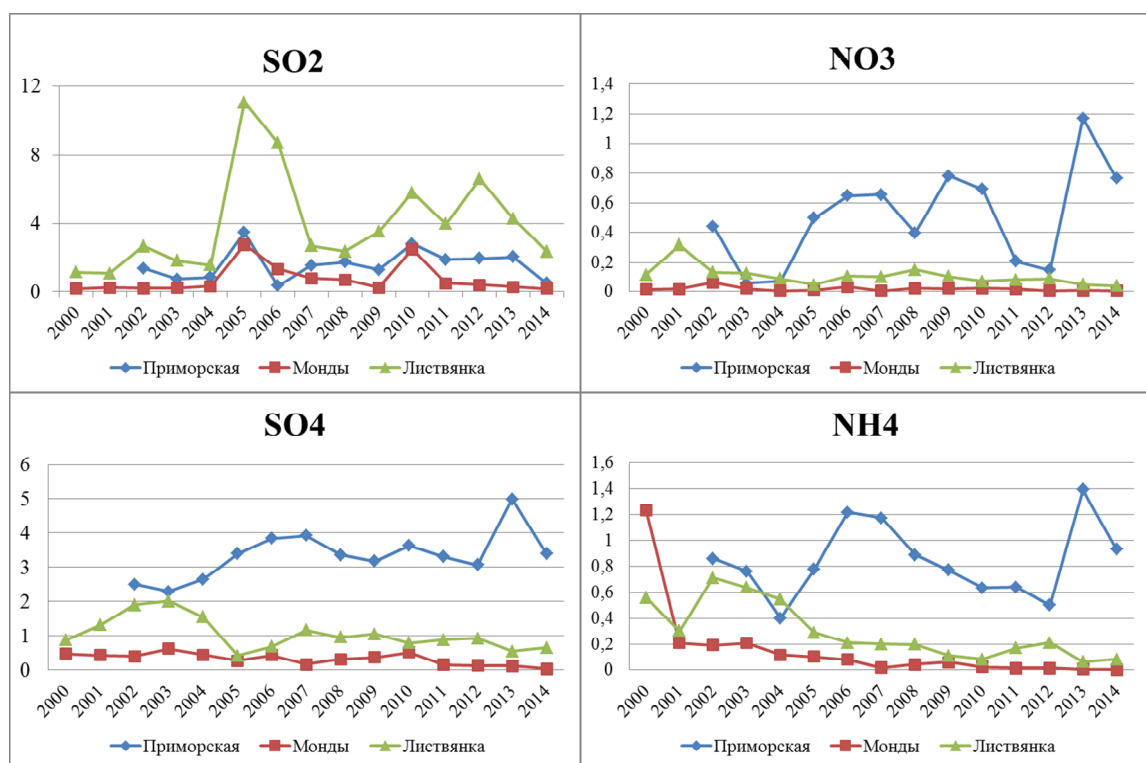
Рис. 1.4.3. Изменения средних годовых концентрации соединений серы (слева) и азота (справа) в воздухе на станциях ЕАНЕТ ( \mu\text{кг}/\text{м}^3 ).
