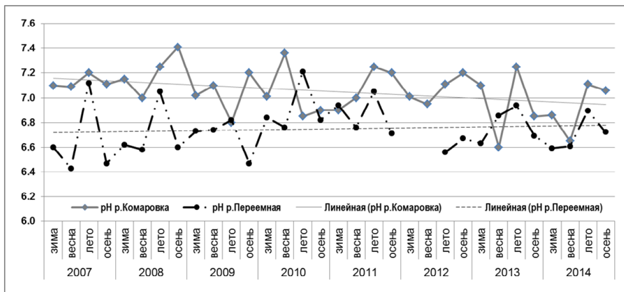
Рис.3.3.2. Тенденции изменения рН в поверхностных водах на станциях ЕАНЕТ в Приморье и в районе оз. Байкал.
