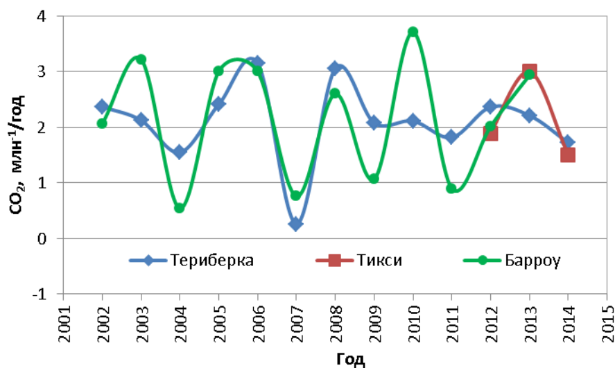
Рис. 1.2.1.1. Межгодовые изменения концентрации CO 2
