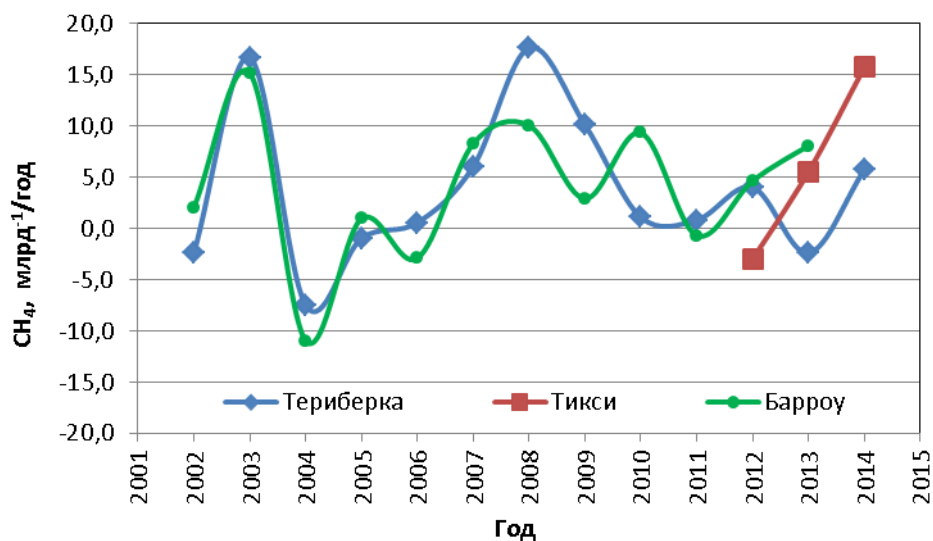
Рис. 1.2.1.2. Межгодовые изменения концентрации CH 4
