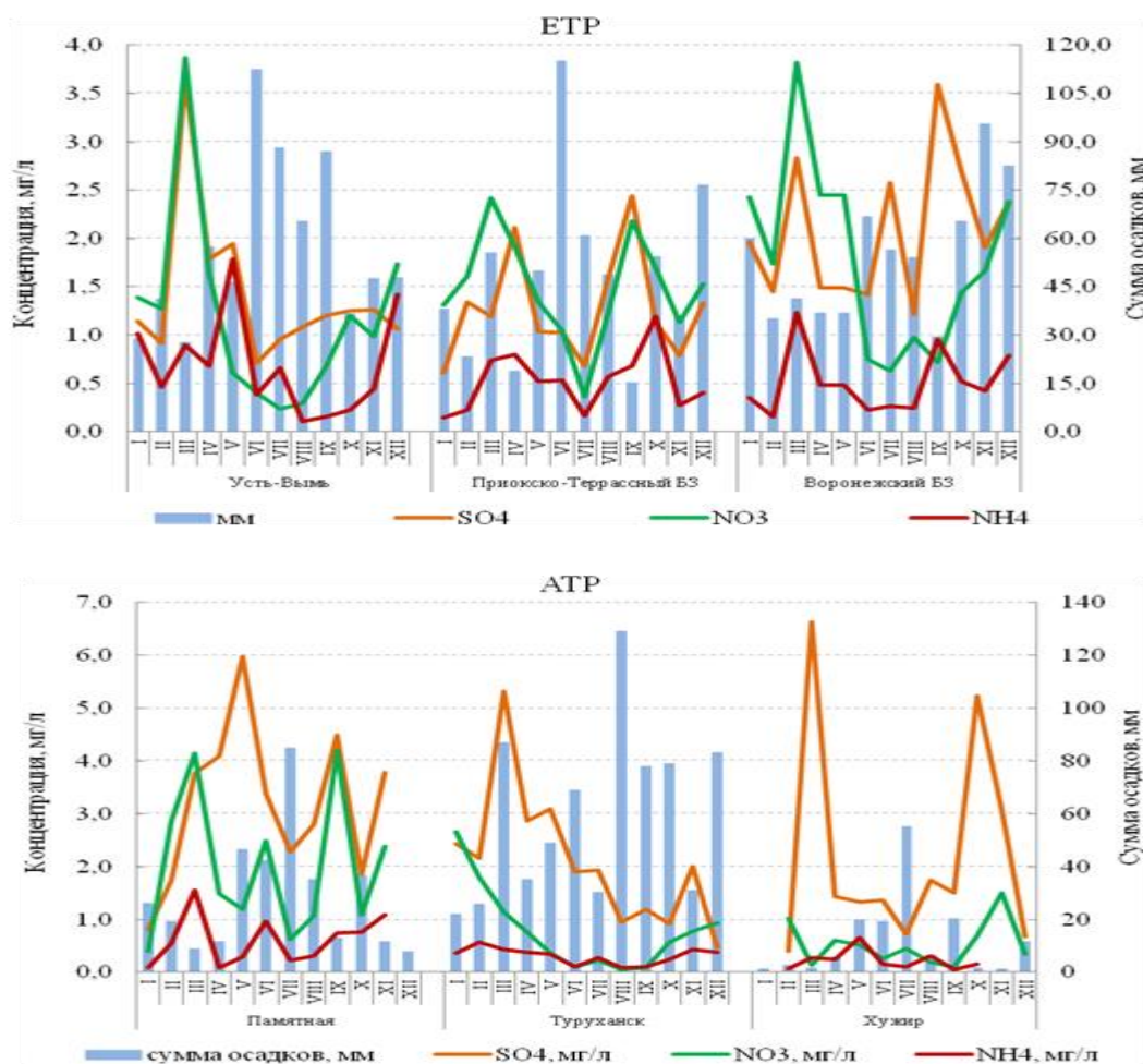
Рис. 1.3.6 (начало). Годовой ход содержания в атмосферных осадках сульфатов, нитратов и аммония, 2017 г.
