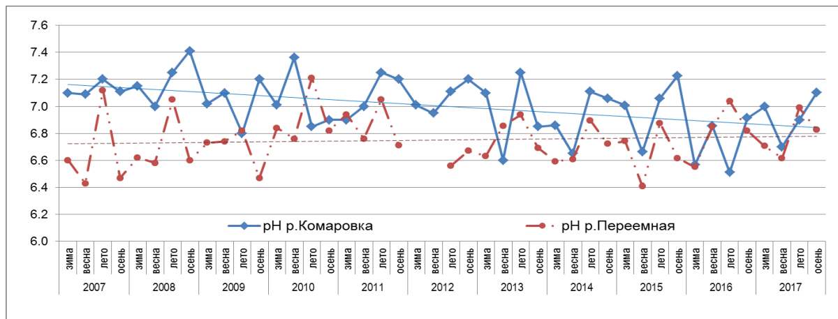
Рис.3.3.1 Тенденции изменения pH в поверхностных водах на станциях ЕАНЕТ в Приморье и в районе оз. Байкал.
