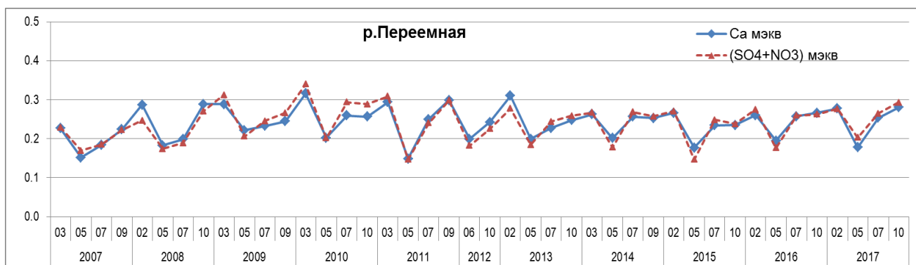
Рис.3.3.9 Тренды согласованного изменения сульфатов, нитратов и кальция (верхний, мг/л) и их эквивалентов (нижний, мэкв/л) в поверхностных водах р. Переемная в 2007-2017 гг.
