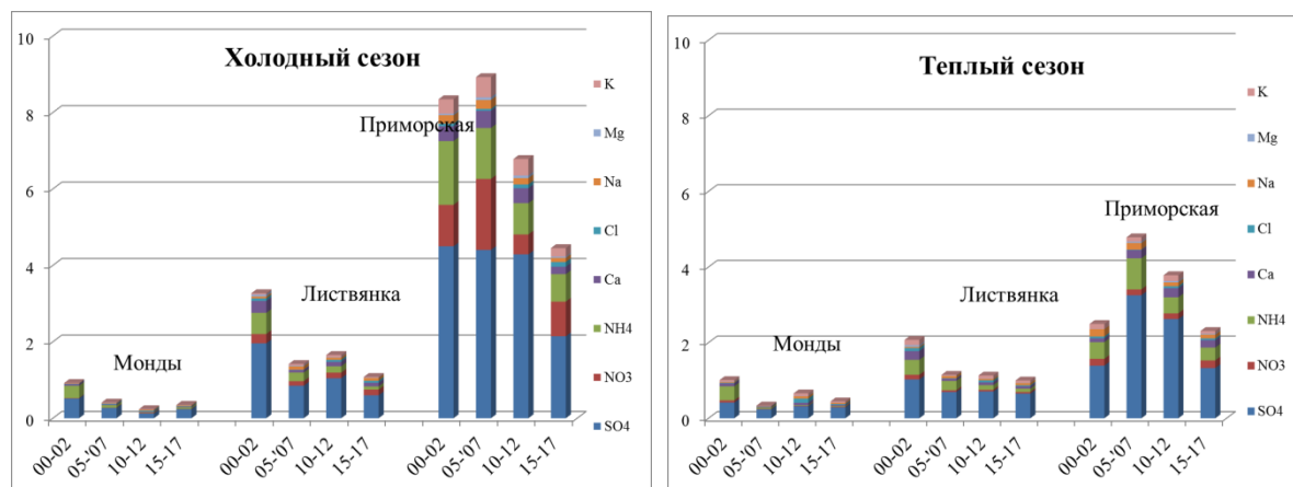
Рис. 1.4.1 Изменение среднего химического состава аэрозолей ( \text{мкг/м}^3 ) на станциях ЕАНЕТ в холодный (слева) и теплый (справа) периоды по наблюдениям в 2000-2017 г.
