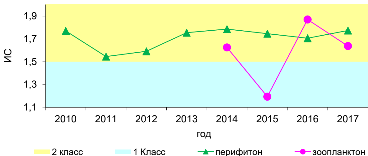
Рис. 3.4.5 Значения ИС в 2010-2017 гг., р. Базаиха
