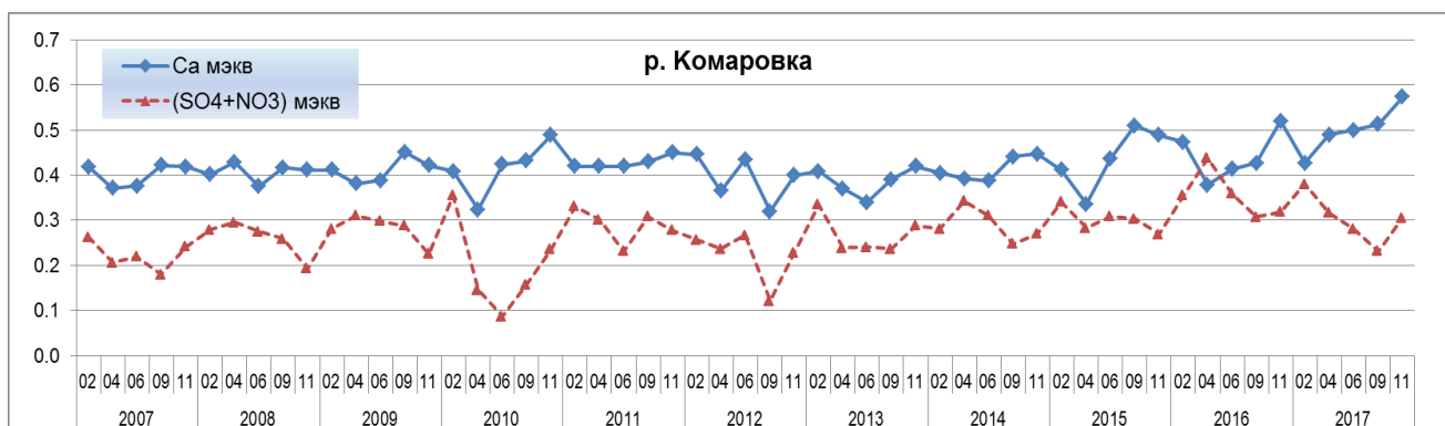
Рис.3.3.8 Тренды согласованного изменения сульфатов, нитратов и кальция (верхний, мг/л) и их эквивалентов (нижний, мэкв/л) в поверхностных водах на станции ЕАНЕТ Приморская в 2007-2017 гг.
