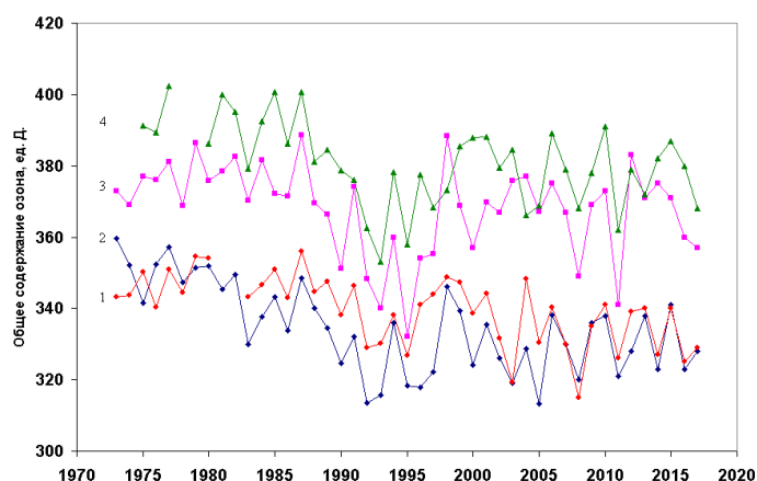
Рис. 1.2.8 Межгодовой ход среднегодовых значений ОСО в пунктах наблюдений: 1 - Екатеринбург (57° N, 61° E), 2 - Санкт-Петербурга (60° N, 30° E), 3 - Якутск (62° N, 130° E), 4 - Нагаево (60° N, 151° E).
