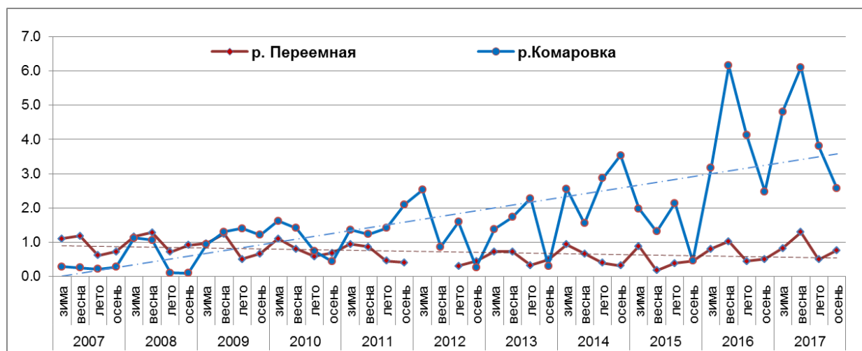
Рис.3.3.4 Тенденции изменения концентраций нитратов (мг/л) в поверхностных водах на станциях ЕАНЕТ в Приморье (р. Комаровка) и в районе оз. Байкал (р. Переемная).
