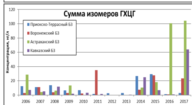
Рис. 1.3.2 Изменение среднего содержания органических загрязняющих веществ в атмосферных осадках фоновых районов в 2006-2017 гг.
