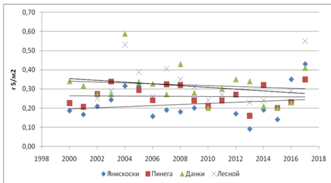
Рис. 1.5.1 Многолетние выпадения сульфатной серы из атмосферы с осадками на станциях ЕМЕП ( gS/m^2/год )
