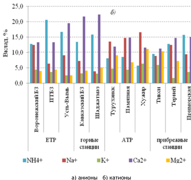
Рис. 1.3.3 (окончание). Вклад (%) ионов в химический состав атмосферных осадков фоновых станций, 2017 г.
