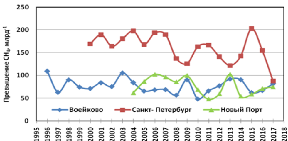
Рис. 1.2.3 Среднегодовые превышения концентраций \text{CH}_4 над фоновым уровнем
