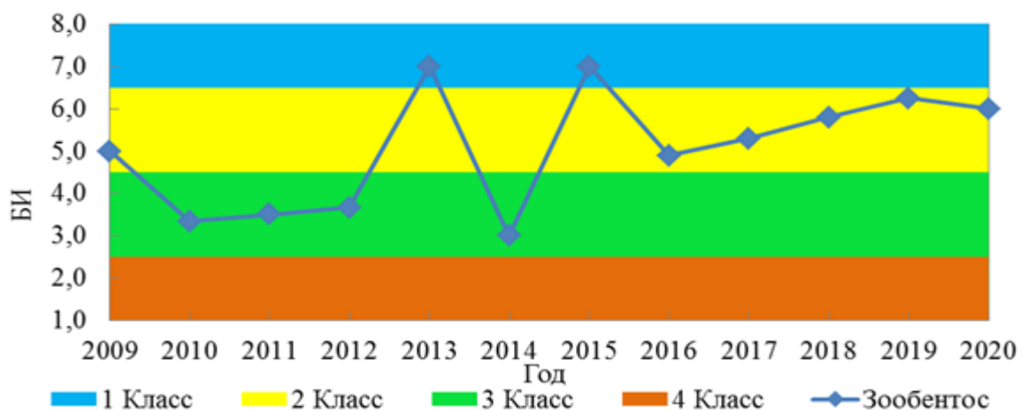
Рис. 3.4.6. Значение БИ в 2009–2020 гг., р. Вите.
