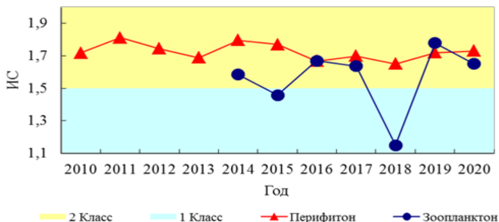
Рис. 3.4.14. Значения ИС в 2010–2020 гг., р. Базаиха
