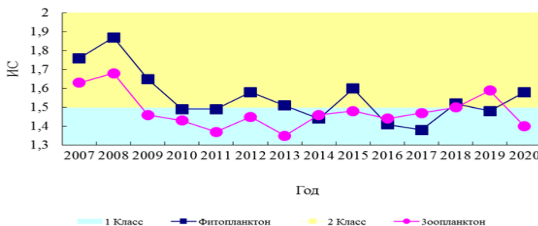
Рис. 3.4.16. Значения ИС в 2007–2020 гг. р. Джиде
