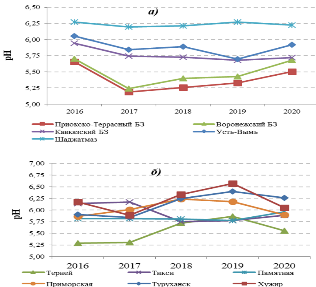
Рис. 1.3.2.2. Изменение среднегодовых значений рН атмосферных осадков фоновых станций на ЕЧР (а) и АЧР (б) в период с 2016 по 2020 гг.
