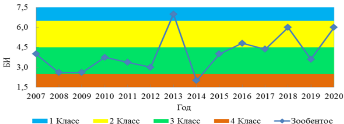
Рис. 3.4.11. Значения БИ в 2007–2020 гг., р.Лена ст.Хабарова
