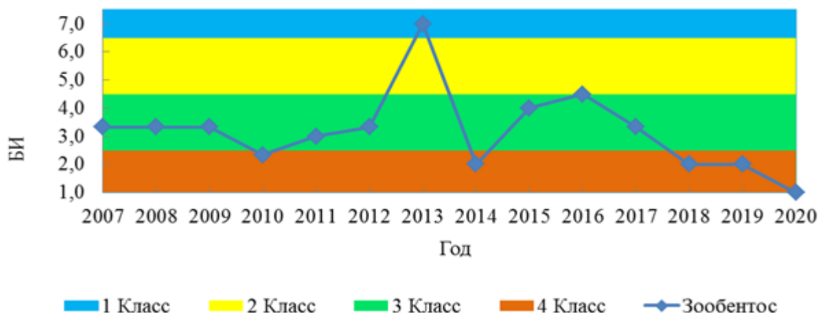
Рис. 3.4.8. Значение БИ в 2009–2020 гг., оз. Чунозеро
