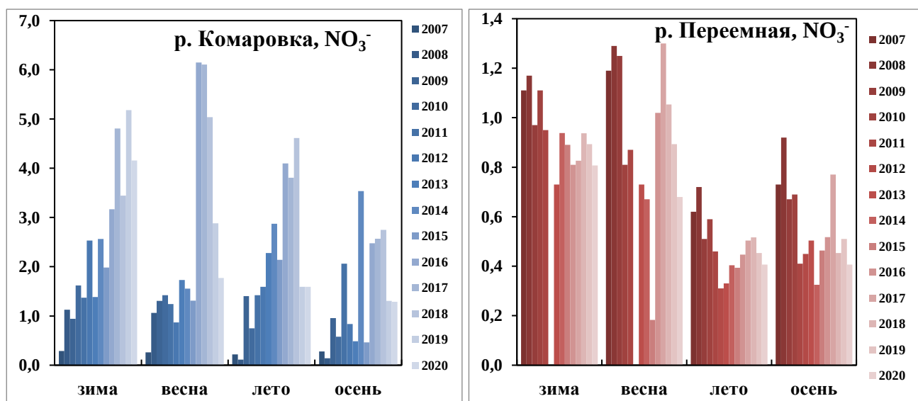
Рис.3.3.3 Внутригодовые изменения концентраций нитратов (мг/л) в р. Комаровка (слева) и р. Переемная (справа) в 2007-2020 гг.
