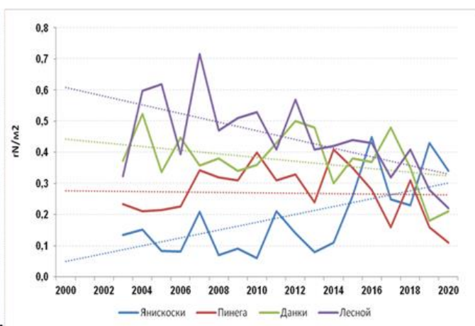
Рис. 1.5.2 . Многолетние выпадения суммарного азота (нитратного и аммонийного) из атмосферы с осадками на станциях ЕМЕП (г N/м²/год)
