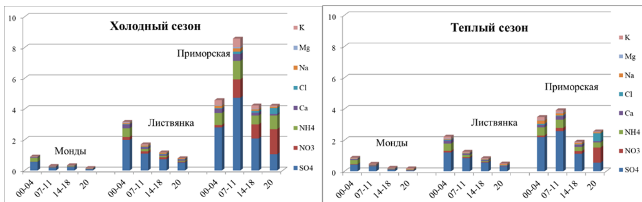
Рис. 1.4.1. Изменение среднего химического состава аэрозолей ( \text{мкг}/\text{м}^3 ) на станциях ЕАНЕТ в холодный (слева) и теплый (справа) периоды по наблюдениям в 2000-2020 гг.
