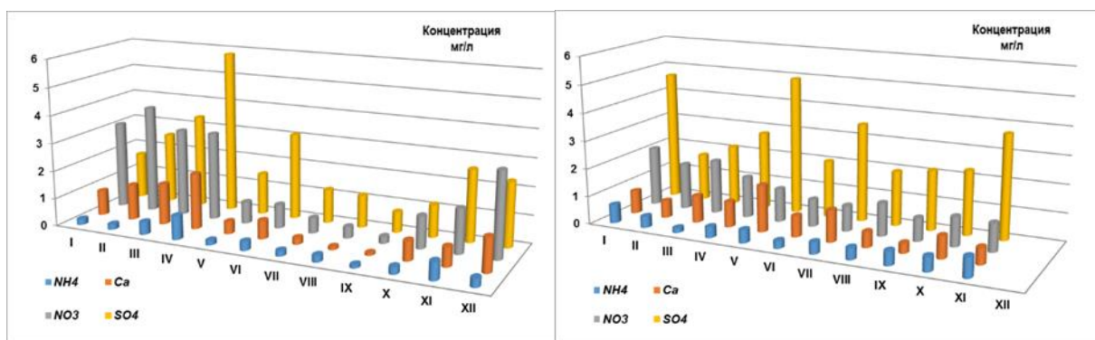
Рис. 1.4.3 (начало). Годовой ход концентраций (верхний) и выпадений (нижний) основных кислотообразующих ионов с осадками в районе оз. Байкал (ст. Листвянка, слева) и на Дальнем Востоке (ст. Приморская, справа) в 2020 г.
