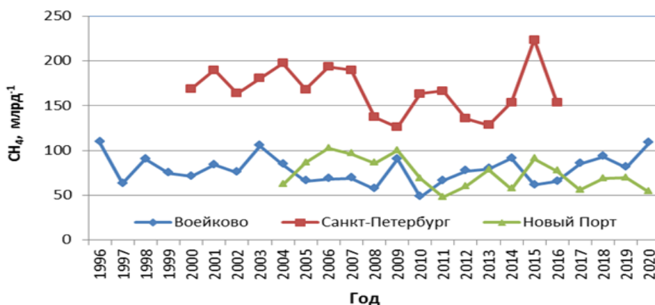
Рис. 1.2.1.3. Среднегодовое превышение концентрации \text{CH}_4 над фоновым уровнем
