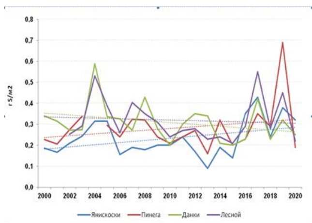
Рис. 1.5.1 . Многолетние выпадения сульфатной серы из атмосферы с осадками на станциях ЕМЕП (г S/м²/год)
