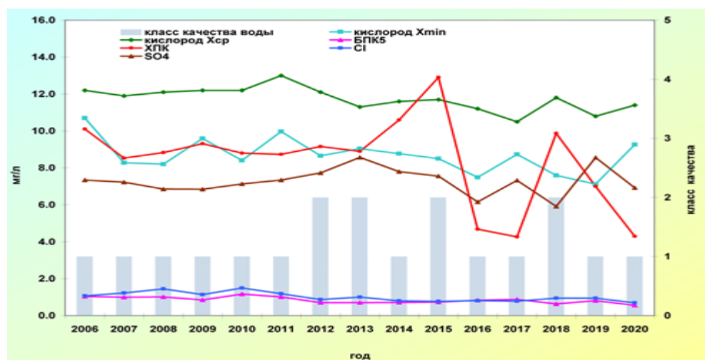
Рис. 3.2.4. Изменение среднегодовых концентраций отдельных ингредиентов и качества воды Иркутского водохранилища, ОГП-1 Исток Ангара в многолетнем плане
