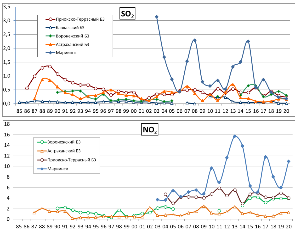
Рис. 1.1.2. Изменение фоновое содержание диоксида серы и диоксида азота в атмосферном воздухе фоновых районов (мкг/м 3 ) за многолетний период (геофизические года)
