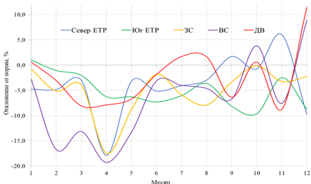
Рис. 1.2.2.3. Отклонения среднемесячных значений ОСО от норм по регионам РФ в 2020 г. (Север ЕЧР – Север Европейской части России, Юг ЕЧР – Юг Европейской части России, ЗС – Западная Сибирь, ВС – Восточная Сибирь, ДВ – Дальний восток)
