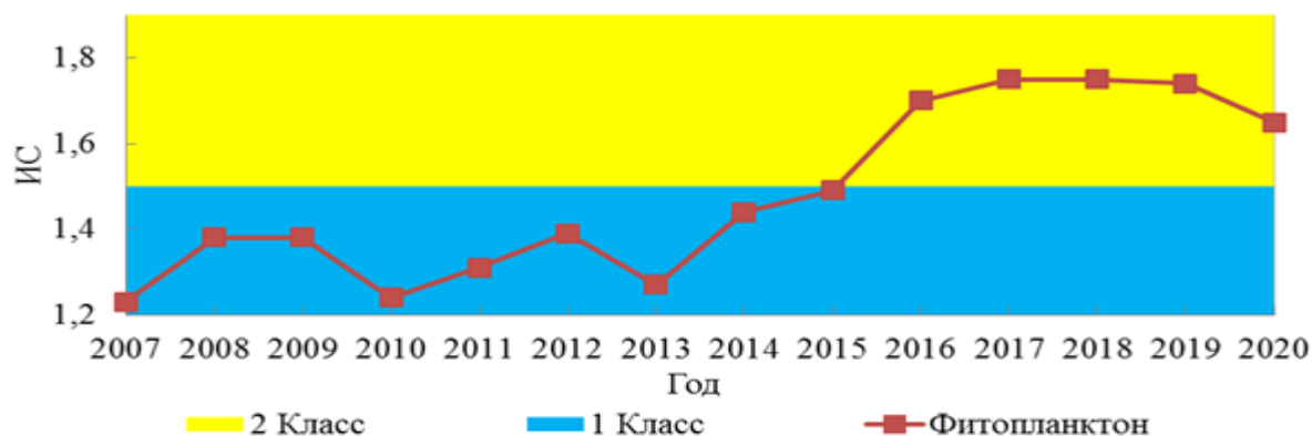
Рис. 3.4.10. Значения ИС в 2007–2020 гг., р. Лена ст. Хабарова
