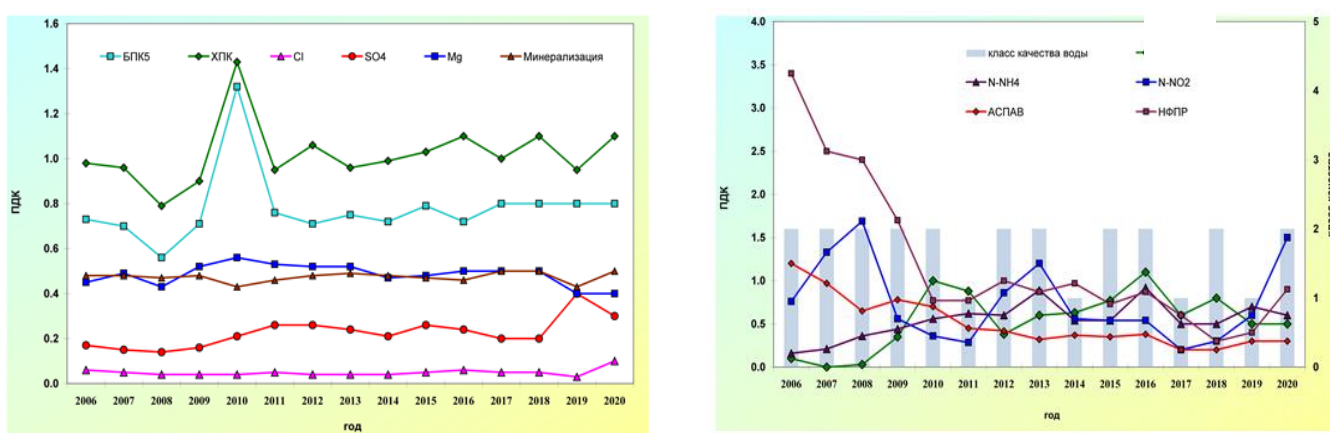
Рис. 3.2.2. Изменение среднегодовых концентраций отдельных ингредиентов и качества воды р. Лесной Воронеж выше г. Мичуринск в многолетнем плане
