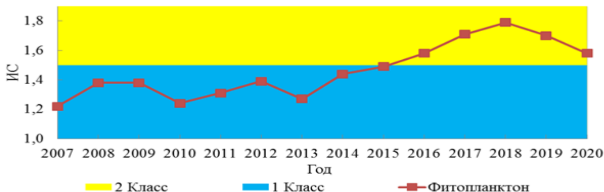
Рис. 3.4.12. Значения ИС в 2007–2020 гг., р. Копчик-Юреге
