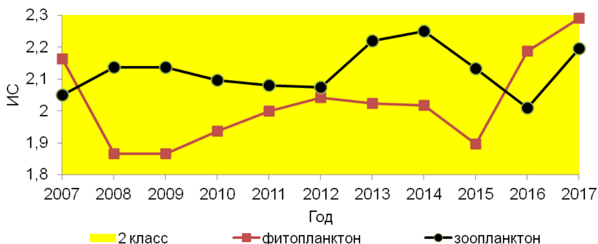
Рисунок 25. Значения ИС в 2009-2017 гг., оз. Ледовое
