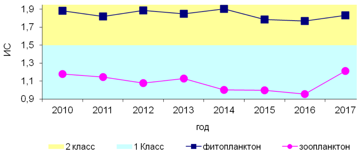
Рисунок 82. Значения ИС в 2010-2017 гг., п. Ангара.
