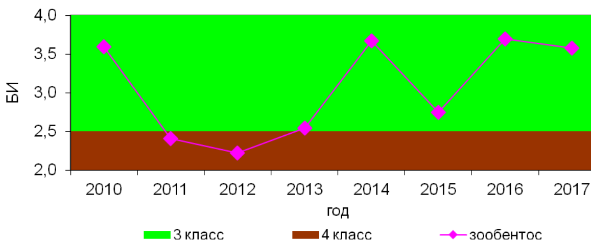
Рисунок 48. Значения БИ в 2010-2017 гг., р.Волга, г.Астрахань
