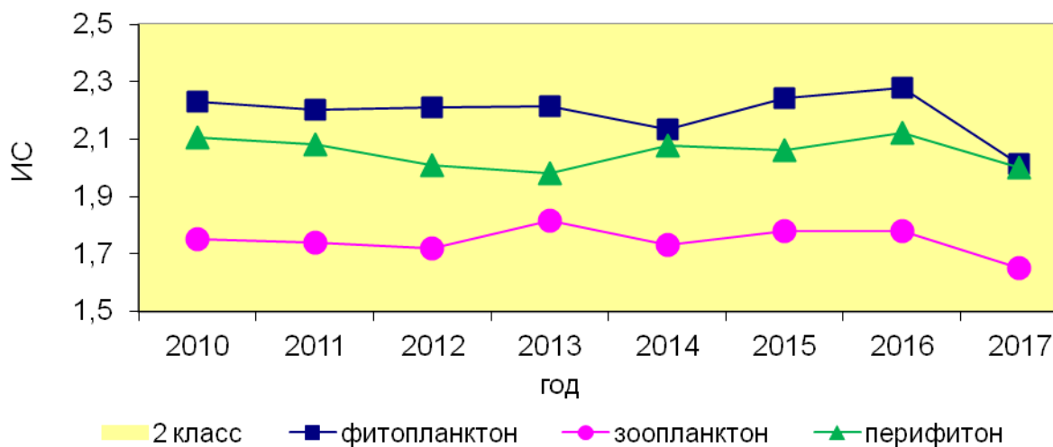
Рисунок 43. Значения ИС в 2010-2017 гг., Саратовское вдхр., г. Самара
