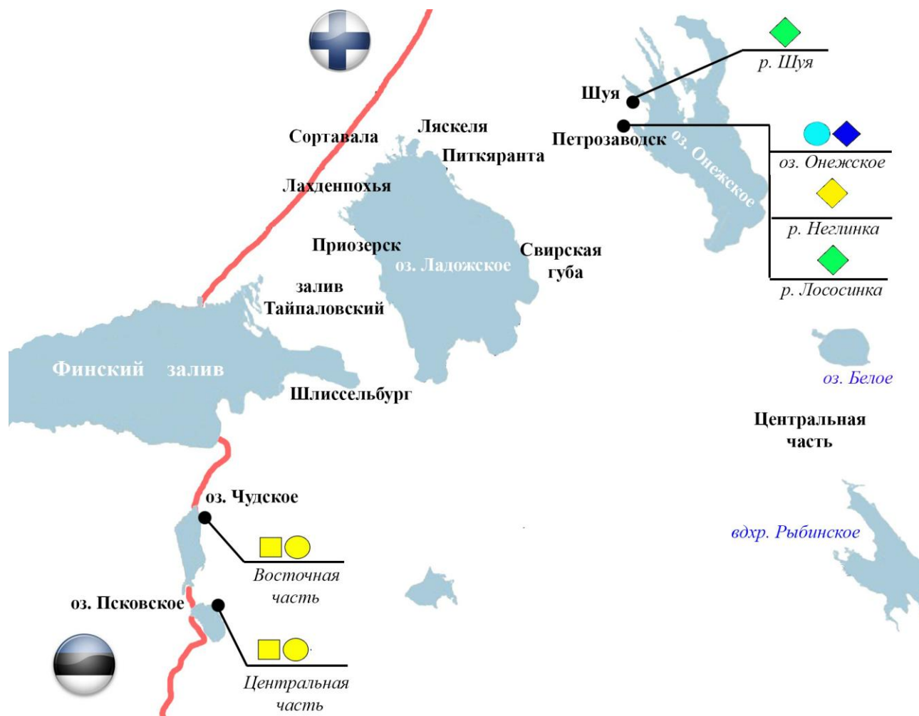
Рисунок 28. Качество вод водоёмов и водотоков Балтийского гидрографического района по гидробиологическим показателям в 2017 году (условные обозначения приведены на стр.12).
