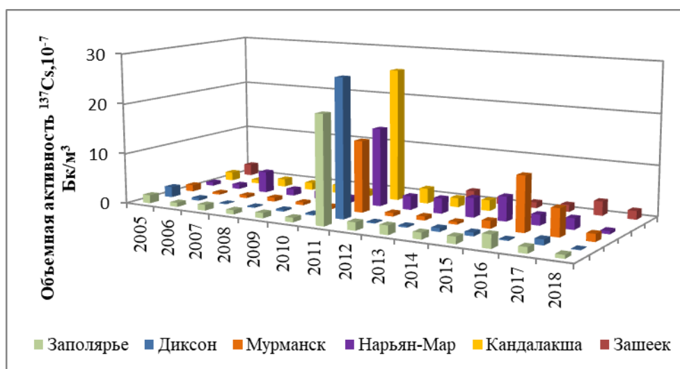
Рис. 4.59. Объемная активность ^{137}\text{Cs} в приземной атмосфере в пунктах наблюдения Сухопутных территорий Арктики и в среднем по Заполярью в 2005-2018 гг., 10^{-7} \text{ Бк/м}^3
