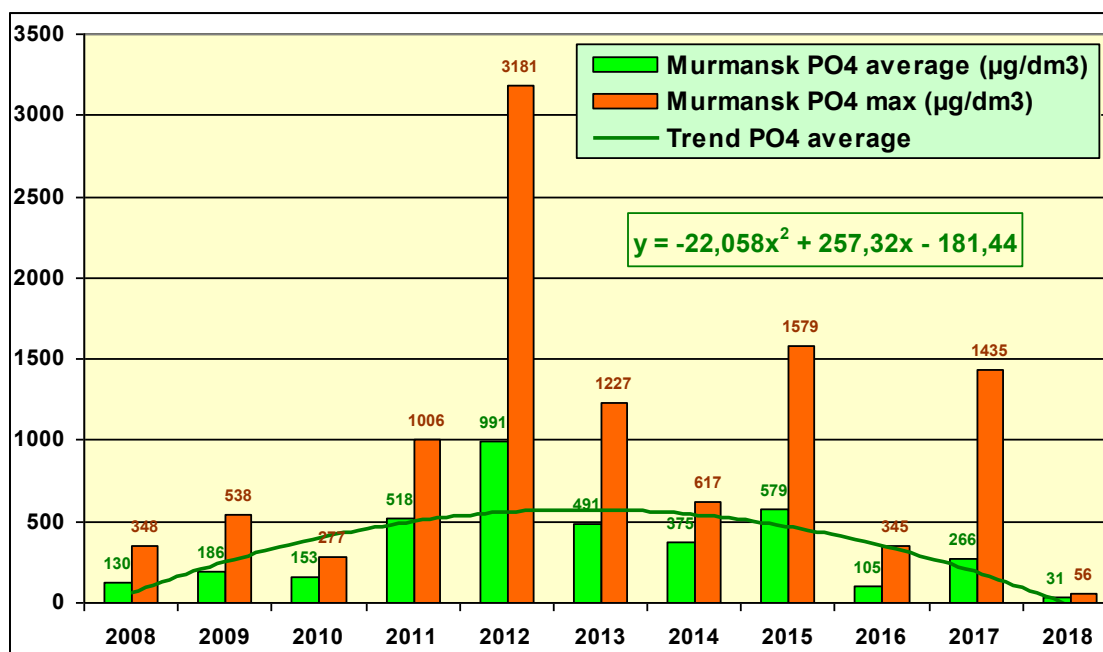
Рис. 3.65. Динамика среднегодовой и максимальной концентраций неорганического фосфора Р-Р 04 (мкг/дм³) в водах водпоста торгового порта г. Мурманска в 2008-2018 гг.
