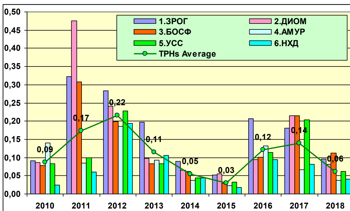
Рис. 3.68. Динамика среднегодовой концентрации нефтяных углеводородов (мг/дм³) в водах различных районов залива Петра Великого Японского моря. 1 - бухта Золотой Рог, 2 - бухта Диомид, 3 - пролив Босфор Восточный, 4 - Амурский залив, 5 - Уссурийский залив, 6 - залив Находка.
