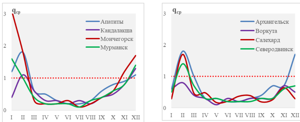
Рис. 4.49. Годовой ход бенз(а)пирена в городах АЗРФ в 2018 г., q_{ср} , нг/м³
