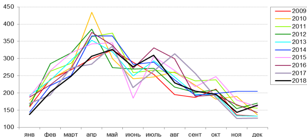
Рис. 3.49. Динамика внутригодового распределения количества случаев ВЗ и ЭВЗ поверхностных вод суши на территории Российской Федерации за период 2009-2018 гг.
