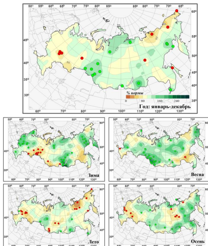
Рис. 1.11. Аномалии годовых и сезонных сумм осадков на территории России в 2018 г. (% от нормы 1961-1990 гг.). Кругами красного и зеленого цвета показаны станции, на которых осадки оказались соответственно ниже 5-го или выше 95-го процентиля.
