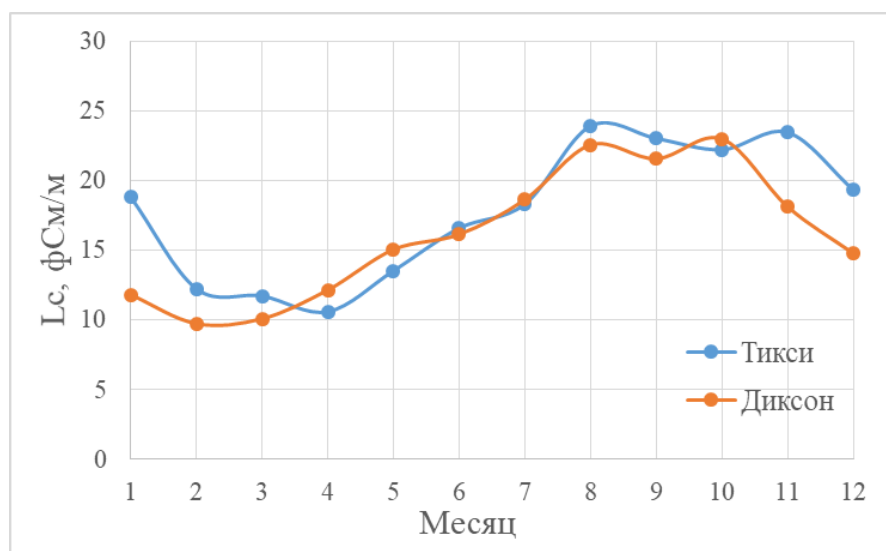
Рис. 4.36. Годовой ход L_5 на станциях Тикси и Диксон за период измерений
