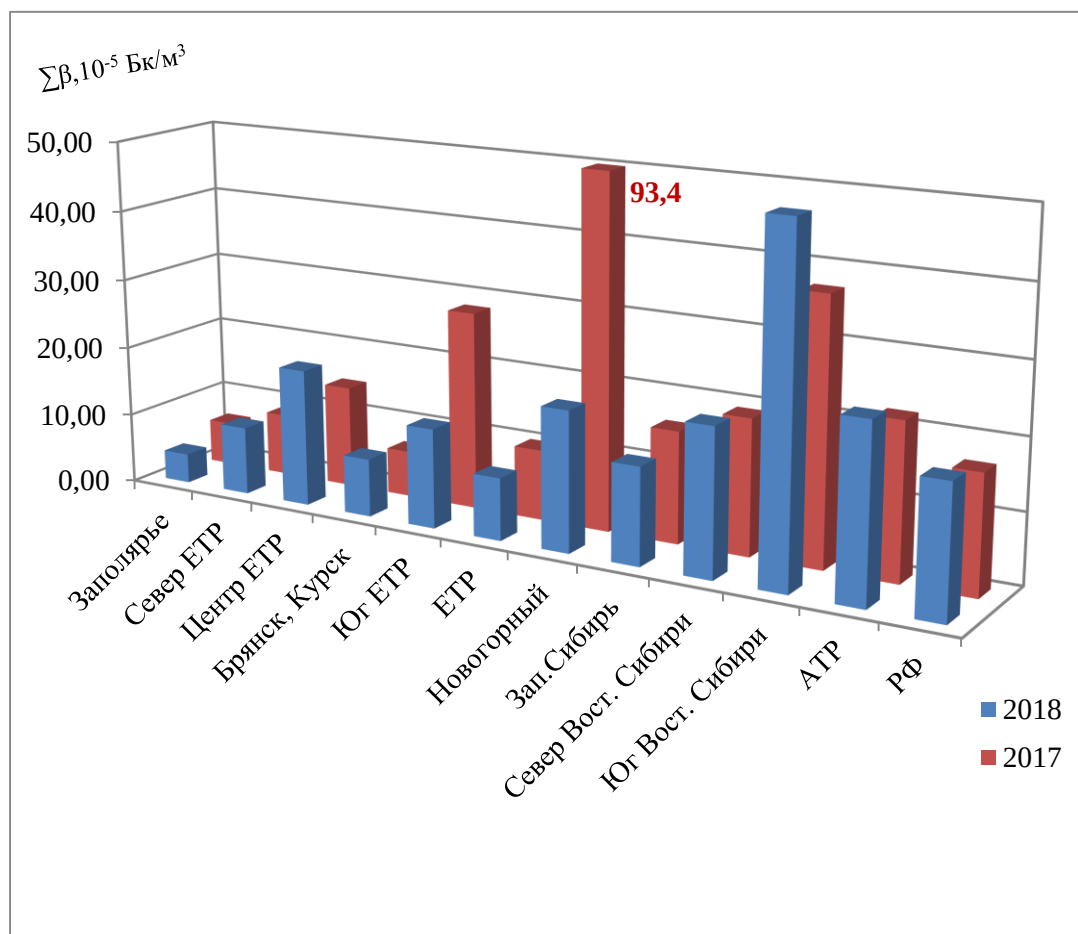
Рис. 2.43. Средние значения объемной \Sigma\beta в приземном слое атмосферы на территории РФ в 2017-2018 гг., 10^{-5} Бк/м 3
