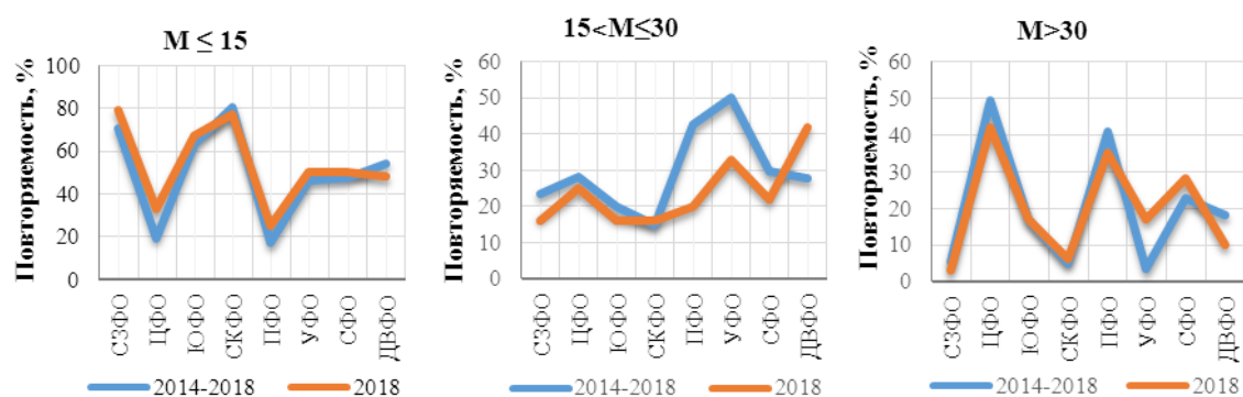
Рис. 2.21. Повторяемость (%) минерализации осадков ( M , мг/л) по диапазонам в период с 2014 по 2018 гг.
