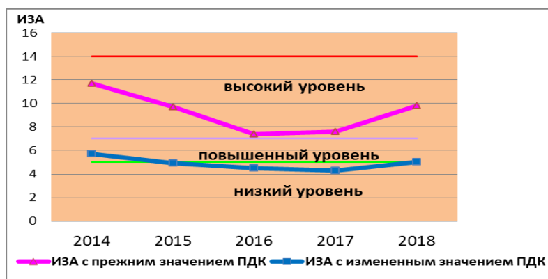
Рис. 4.5. Изменения значений комплексного ИЗА, рассчитанных с прежним и измененным значениями ПДКс.с. формальдегида, соотношенные с уровнями загрязнения атмосферного воздуха
