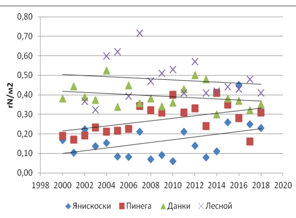
Рис. 2.29. Многолетние выпадения суммарного азота (нитратного и аммонийного) из атмосферы с осадками на станциях ЕМЕП (г N/м 2 /год)
