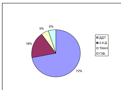
Рис. 3.25. Доля площади, загрязненной различными пестицидами
