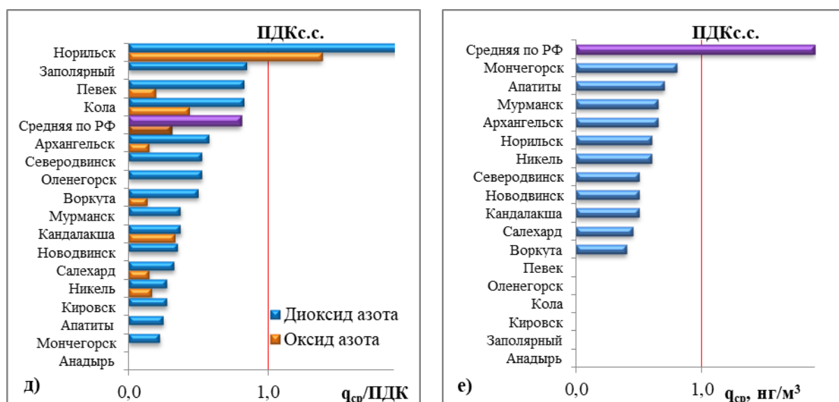
Рис. 4.48. Средние за год концентрации: взвешенных веществ (а), диоксида серы (б), оксида углерода (в), формальдегида (г), q_{ср} , мг/м³, диоксида и оксида азота (д), q_{ср} , ПДК, бенз(а)пирена (е), q_{ср} , нг/м³, в городах АЗРФ и в целом по России в 2018 г.
