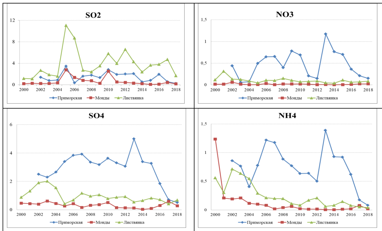
Рис. 2.31. Изменения средних годовых концентрации соединений серы (слева) и азота (справа) в воздухе на станциях ЕАНЕТ (мкг/м 3 )
