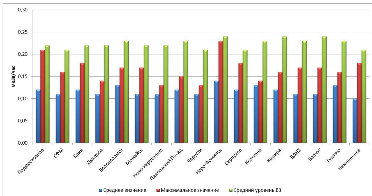
Рис. 4.15. Мощность AMBIENT EQUIVALENT DOSE OF GAMMA RADIATION (МАЭД) на станциях Московского региона в 2018 г.
