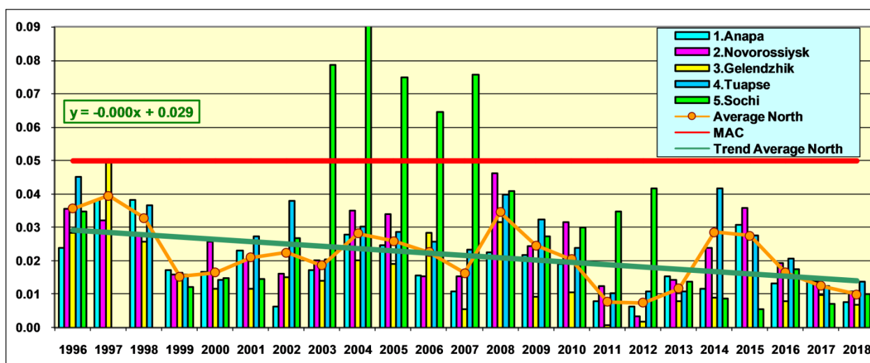
Рис. 3.59. Динамика среднегодовой концентрации нефтяных углеводородов (мг/дм³) в прибрежных водах Кавказа в 1996-2018 гг. Сокращения: Average North - средняя величина в северной части Кавказского побережья; MAC - предельно допустимая концентрация; Trend Average North - тренд концентрации НУ в северной части побережья.
