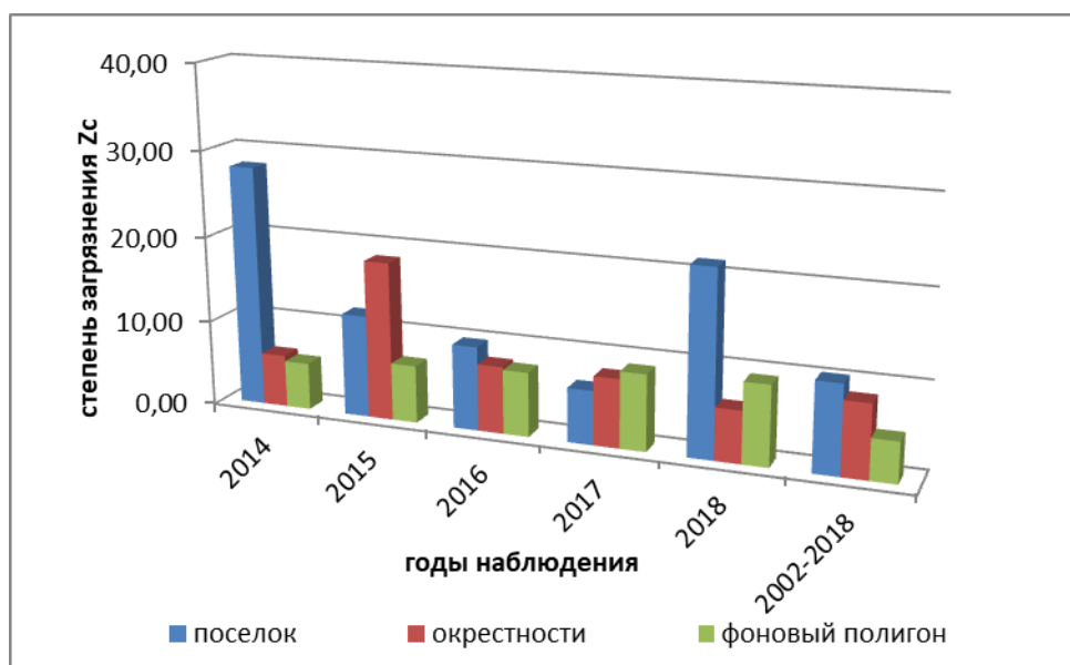
Рис. 4.65. Межгодовая изменчивость суммарного показателя химического загрязнения Z_c в районе поселка Баренцбург, его окрестностях и фоновых территориях в период 2014-2018 гг. и осредненные значения за 2002-2018 гг
