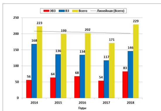
Рис. 4.50. Динамика количества случаев ВЗ и ЭВЗ поверхностных вод Арктической зоны РФ
