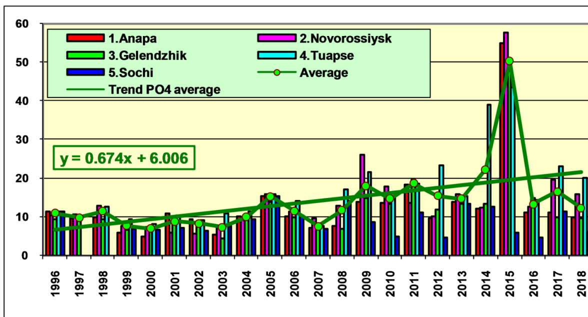
Рис. 3.60. Динамика среднегодовой концентрации фосфатов P-PO 4 (мг/дм³) в прибрежных водах Кавказа в 1996-2018 гг. Примечание: Average - средняя концентрация фосфатов; Trend PO 4 average - тренд средней концентрации фосфатов.
