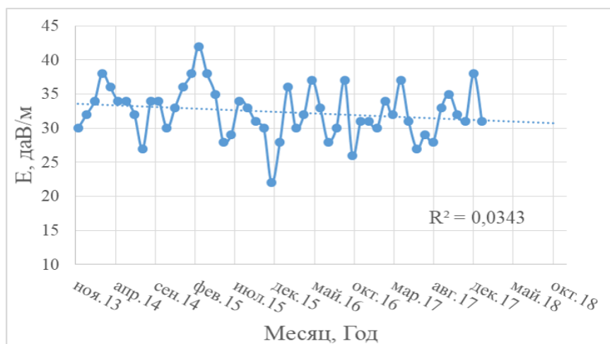
Рис. 4.34. Среднемесячные значения V' по данным наблюдения на станции Тикси в период 2014-2018 гг.
