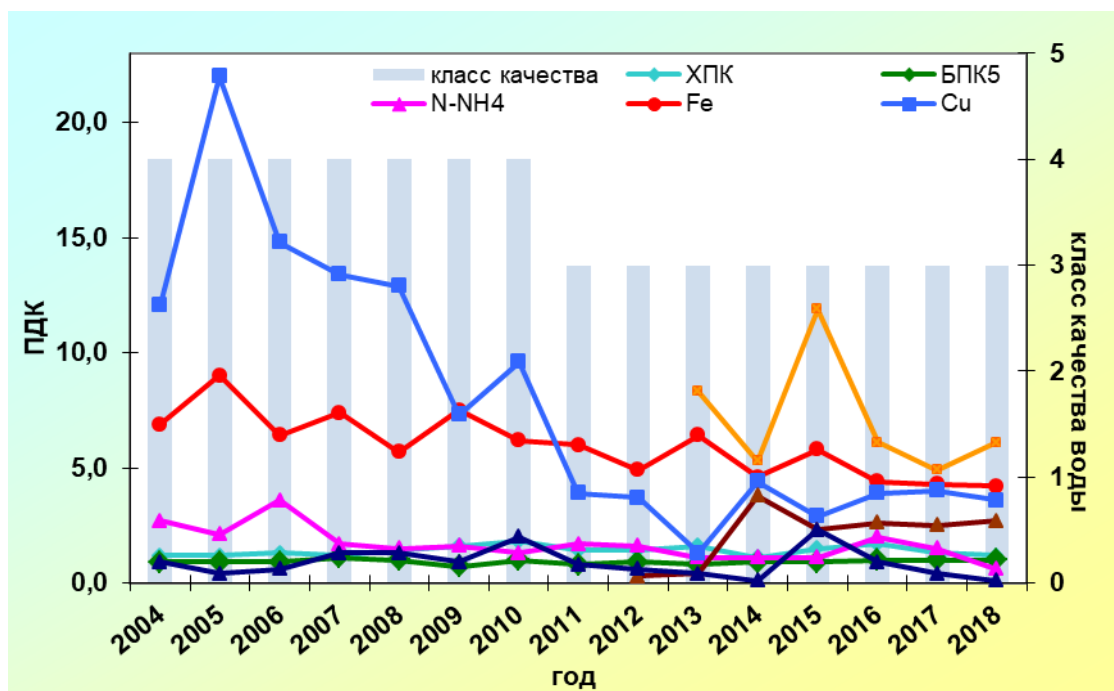
Рис. 3.46. Динамика среднегодового содержания основных загрязняющих веществ в воде р. Амур, в пункте г. Амурск
