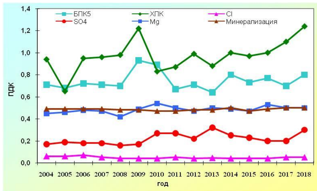
Рис. 2.34 (начало). Изменение среднегодовых концентраций отдельных ингредиентов и качества воды р. Ворона в черте г. Уварово в многолетнем плане
