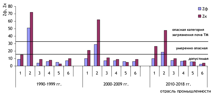
Рис. 3.21. Динамика усреднённых за несколько лет приоритетных показателей загрязнения почв комплексом ТМ ( Z_f , Z_k ) вокруг предприятий черной металлургии (1), цветной металлургии (2), машиностроения и металлообработки (3), топливной и энергетической промышленности (4), химической и нефтехимической промышленности (5), строительной промышленности и производства стройматериалов (6)
