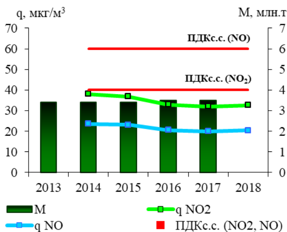
Рис. 3.12. Среднегодовые концентрации диоксида ( q\text{NO}_2 , мкг/м³) и оксида азота ( q\text{NO} , мкг/м³) и суммарные выбросы ( M , млн. т) \text{NO}_x (в пересчете на \text{NO}_2 )
