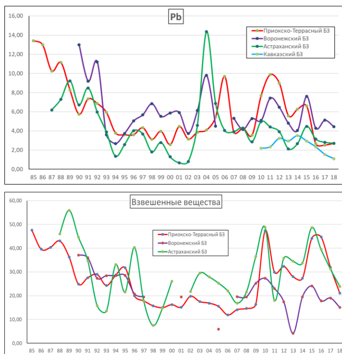
Рис. 2.15. Изменение среднегодового содержания свинца ( \text{нг/м}^3 ) и взвешенных частиц ( \text{мкг/м}^3 ) в атмосферном воздухе фоновых районов
