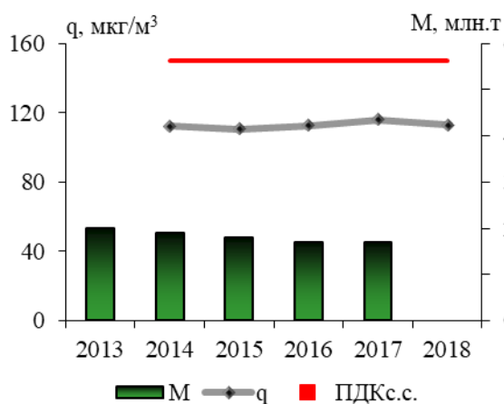
Рис. 3.9. Среднегодовые концентрации ( q , мкг/м 3 ) взвешенных веществ и выбросы от стационарных источников ( M , млн. т) твердых веществ
