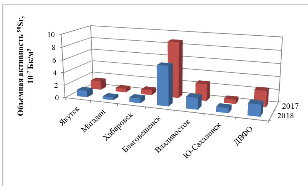
Рис. 2.46. Среднегодовая объемная активность 90 Sr в населенных пунктах ДВФО в 2017-2018 гг., 10 -7 Бк/м 3
