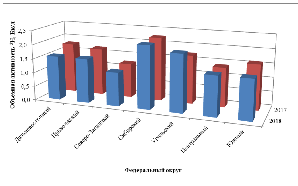
Рис. 2.47. Среднегодовая объемная активность 3 H в атмосферных осадках на территории федеральных округов РФ в 2017-2018 гг., Бк/л
