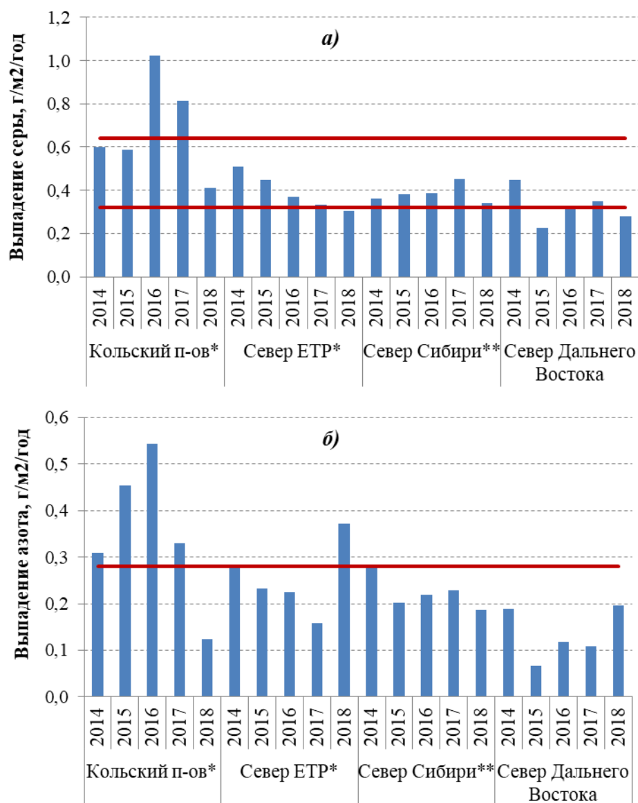
Рис. 4.44. Межгодовой ход влажных выпадений: (а) - серы; (б) - суммарного азота
