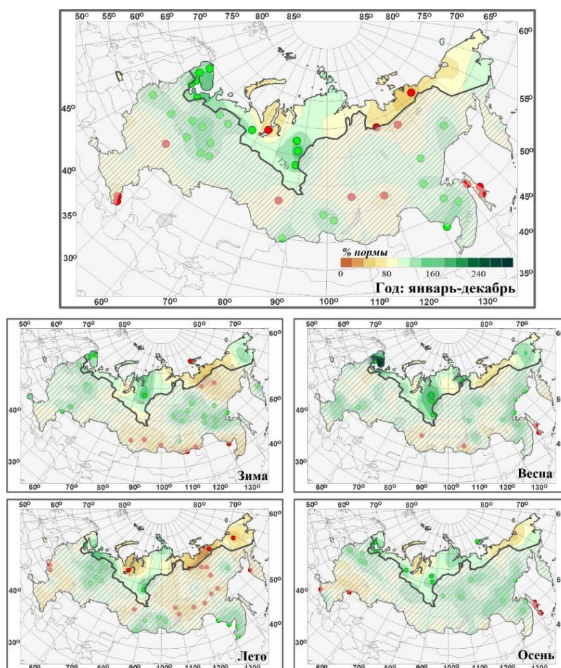
Рис. 4.29. Годовые (январь-декабрь) и сезонные суммы осадков (% от нормы периода 1961-90 гг.) в Российской Арктике. Зелеными кружками показаны станционные аномалии выше 95-го перцентиля, красными - ниже 5-го.
