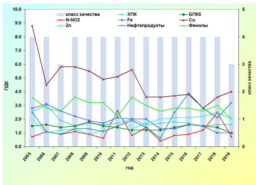
Рис. 3.38. Изменение среднегодовых концентраций отдельных ингредиентов и качества воды р. Волга, 5,5 км ниже г. Астрахань за многолетний период
