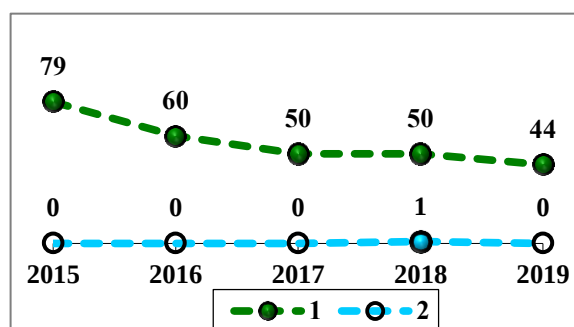
Рис. 3.6. Количество городов, в которых среднегодовые концентрации диоксида азота превысили 1 ПДК (1), СИ диоксида азота больше 10 (2)
