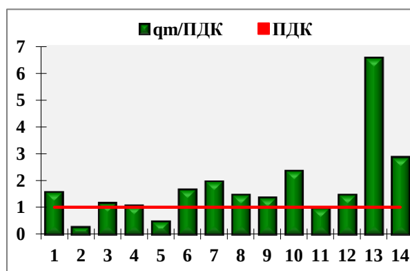
Рис. 3.18. Средние из максимальных концентрации примесей в городах России 1 - взвешенные вещества, 2 - диоксид серы, 3 - оксид углерода, 4 - диоксид азота, 5 - оксид азота, 6 - сероводород, 7 - сероуглерод, 8 - фенол, 9 - фторид водорода, 10 - хлорид водорода, 11 - аммиак, 12 - формальдегид, 13 - бенз(а)пирен, 14 - этилбензол
