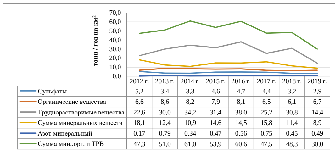
Рис. 4.18. Динамика поступления химических веществ из атмосферы на ст. Большое Голоустное
