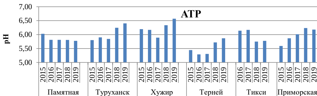
Рис. 2.18 (окончание). Изменение среднегодовых значений pH атмосферных осадков фоновых станций в период с 2015 по 2019 гг.
