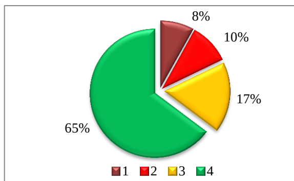
Рис. 3.15. Количество городов (%), где ИЗА \geq 14 (1), 7-13 (2), 5-6 (3), \leq 5 (4)
