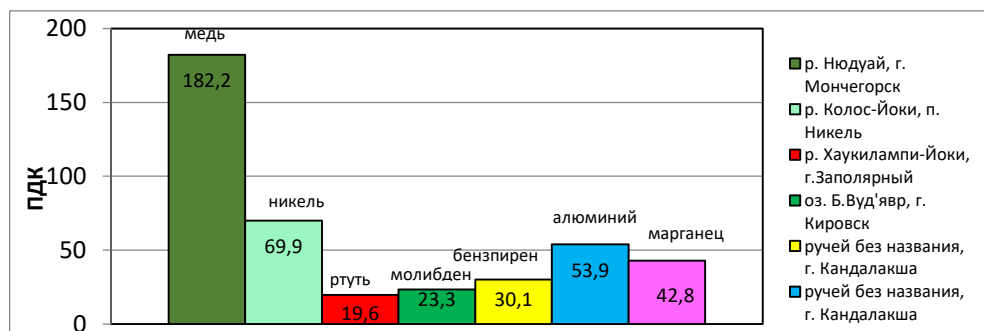
Рис. 4.50. Максимальные значения ПДК основных загрязняющих веществ в водных объектах Мурманской области в 2019 г.
