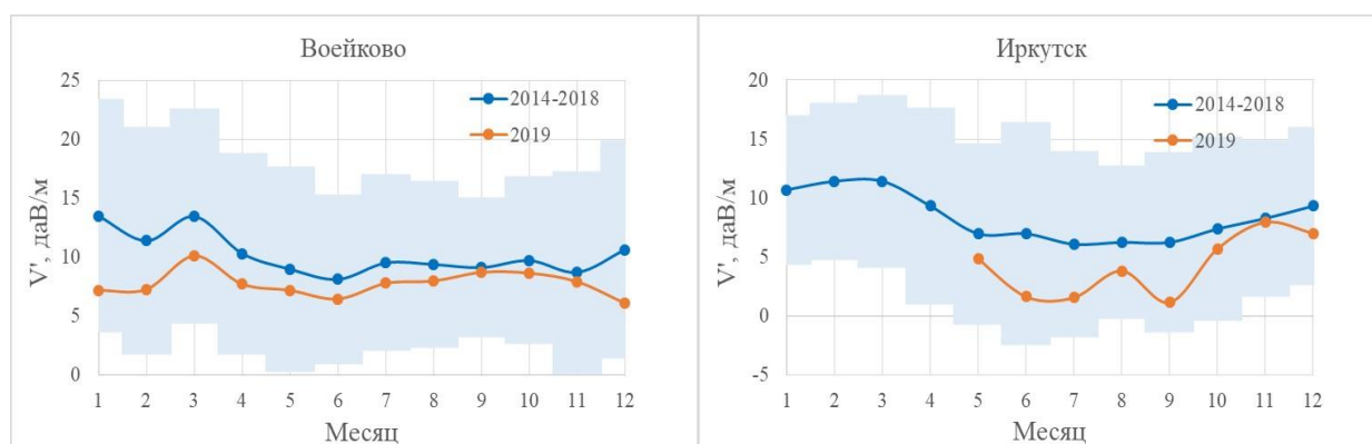
Рис. 2.8. Годовой ход V' по станциям атмосферно-электрической сети Воейково и Иркутск в 2019 г. на фоне осредненного годового хода V' за период 2014-2018 гг.
