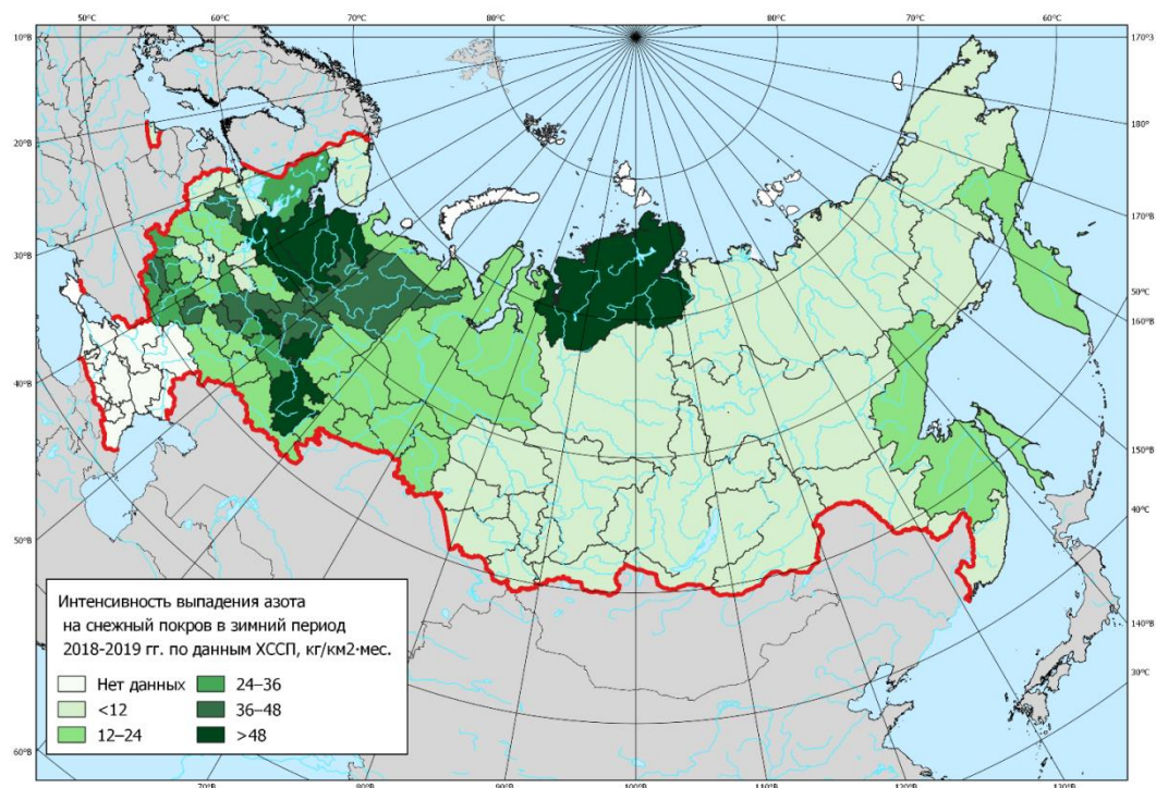
Рис. 2.26. Интенсивность выпадения азота на снежный покров в 2019 г.
