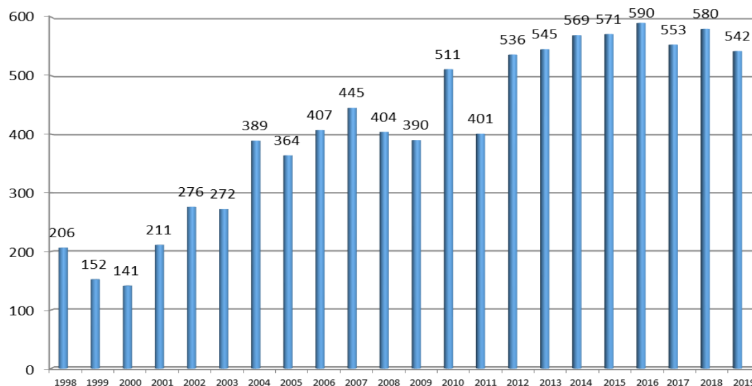
Рис. 1.6. Распределение метеорологических ОЯ по годам
