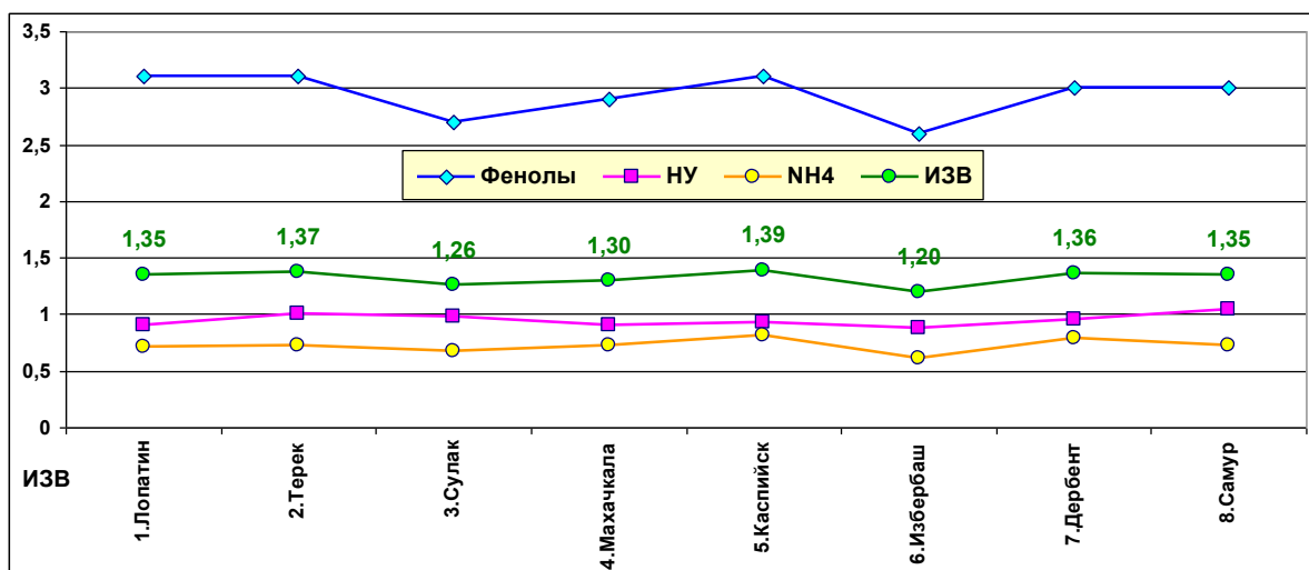
Рис. 3.60. Средняя годовая концентрация (в единицах ПДК) приоритетных загрязнителей и значение ИЗВ вдоль Дагестанского побережья в 2019 г.
