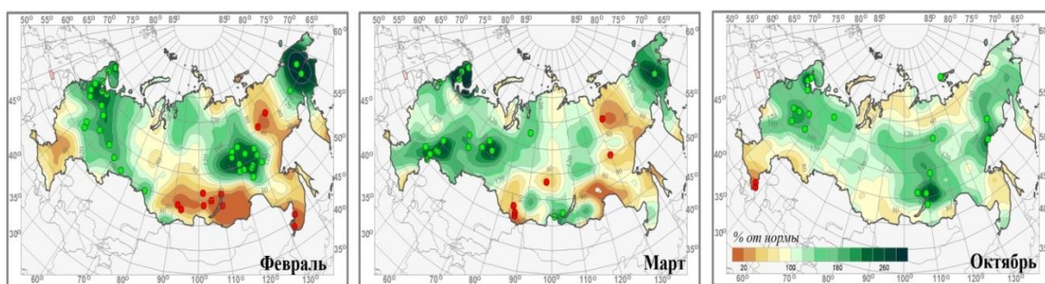
Рис. 1.12. Аномалии сумм осадков в феврале, марте и в октябре 2019 г.
