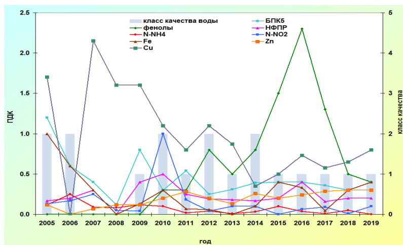
Рис. 2.39 (начало). Изменение среднегодовых концентраций отдельных ингредиентов и качества воды а) р. Голоустная, б) р. Бугульдейка, в) р. Сарма, г) р. Мантуриха, д) р. Мысовка за многолетний период
