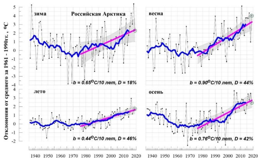
Рис. 4.28. Сезонные аномалии температуры воздуха в Российской Арктике в 1936-2019 гг. Жирная синяя кривая - 11летнее скользящее среднее. Показан линейный тренд за 1976-2019 гг.
