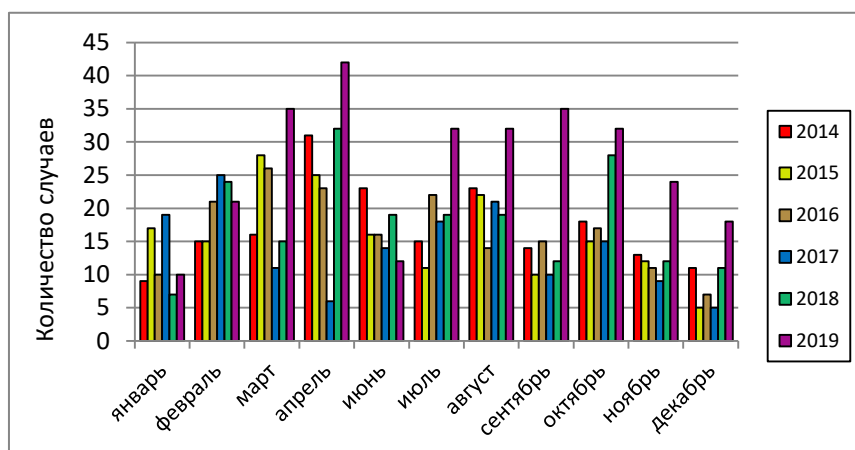
Рис. 4.47. Динамика внутригодового распределения случаев ВЗ и ЭВЗ в поверхностных водах Арктической зоны РФ за период 2014-2019 гг.
