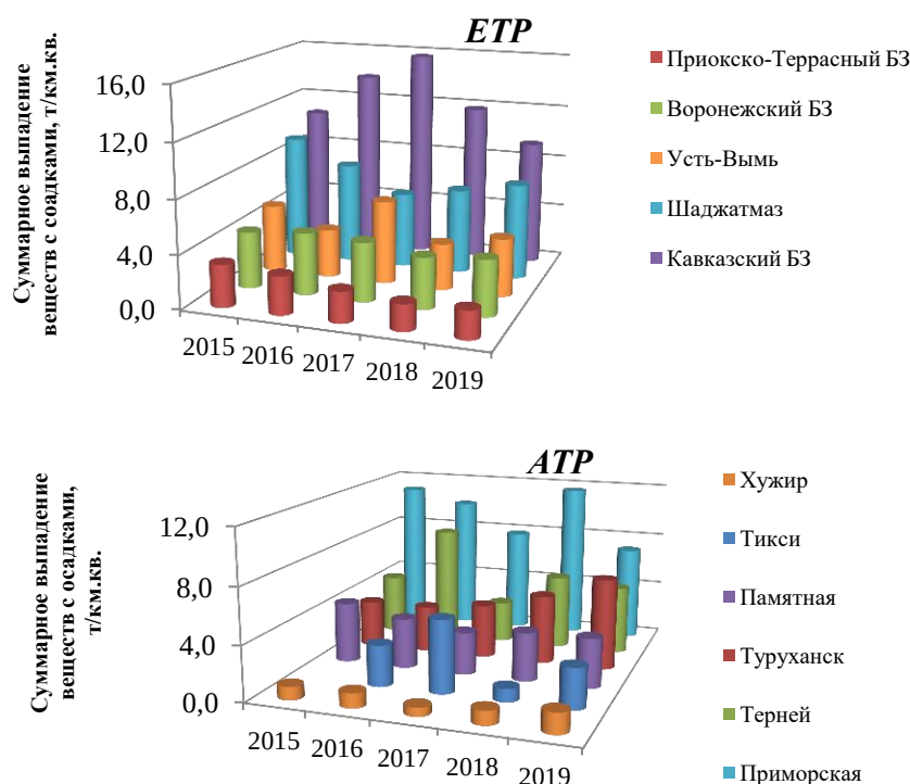
Рис. 2.21. Суммарное поступление веществ с осадками на фоновых станциях в период с 2015 по 2019 гг.
