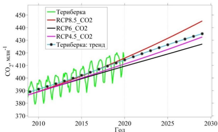
Рис. 4.38. Фактическая концентрация диоксида углерода в Териберке и вероятные концентрации \text{CO}_2 , соответствующие различным сценариям эмиссии \text{CO}_2 (RCP4.5, RCP6 и RCP8.5)
