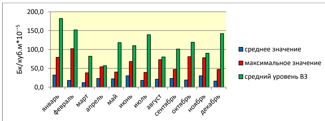
Рис. 4.12. Среднемесячная и максимальная объемная суммарная бета-активность радионуклидов в приземном слое атмосферы в 2019 г.
