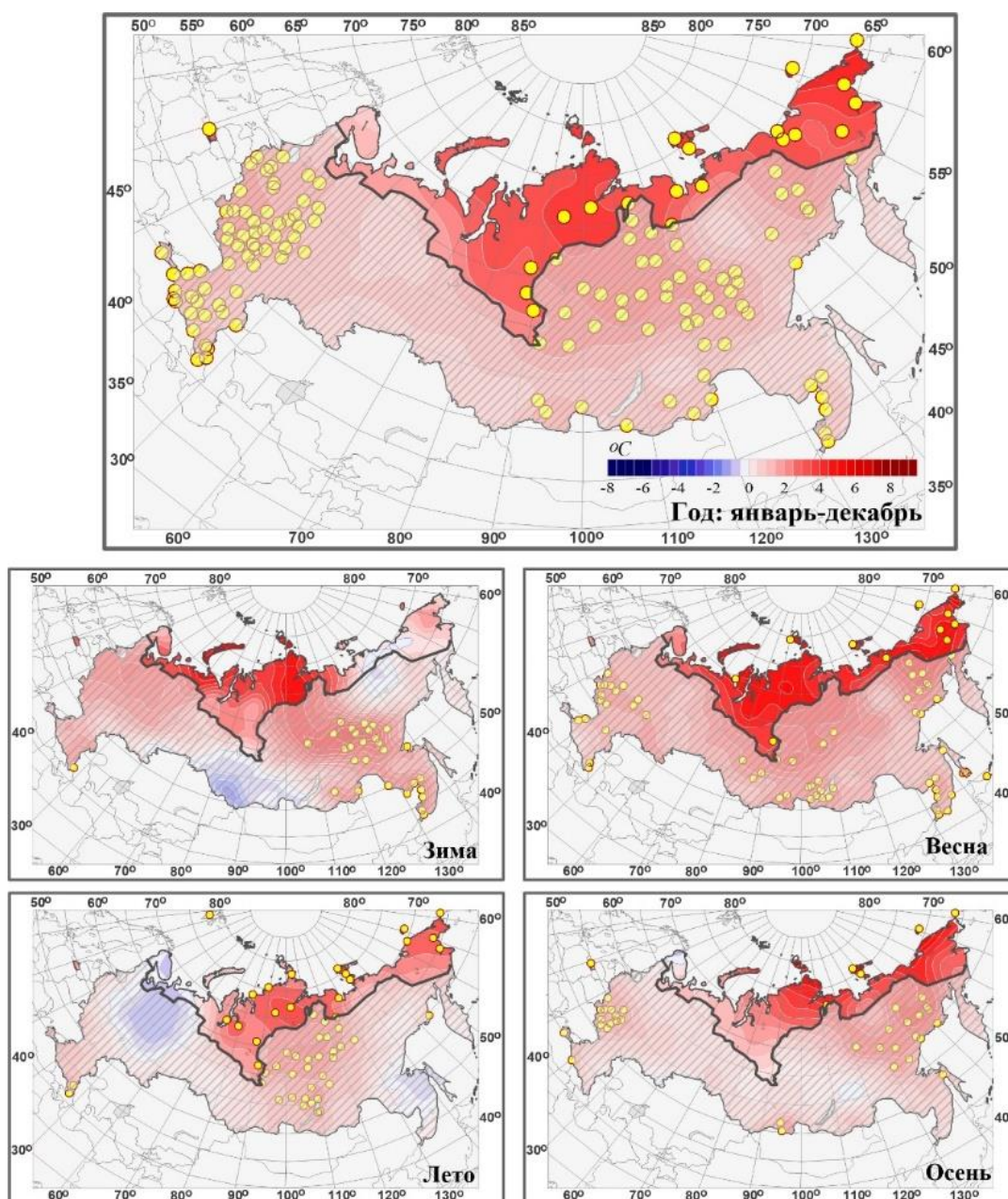
Рис. 4.26. Годовые (январь-декабрь) и сезонные аномалии температуры воздуха в Российской Арктике. Аномалии (°C) рассчитаны относительно норм периода 1961-1990 гг. Желтыми кружками показаны аномалии выше 95-го процента.
