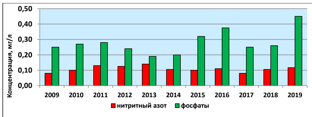
Рис. 4.8. Изменение среднегодовых концентраций нитритного азота и фосфатов в целом по водным объектам Московского региона
