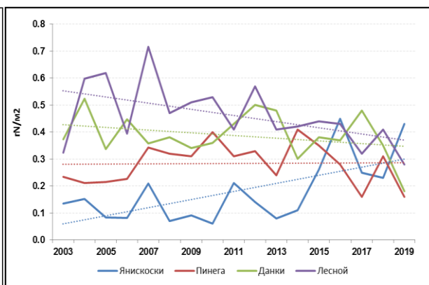
Рис. 2.30. Многолетние выпадения суммарного азота (нитратного и аммонийного) из атмосферы с осадками на станциях ЕМЕП (г N/m²/год)
