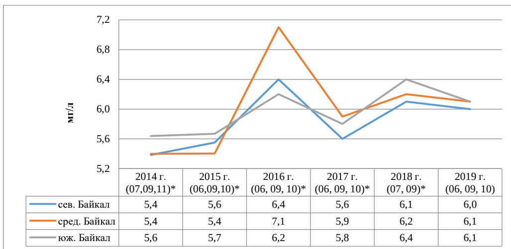
Рис. 4.23. Динамика сульфатных ионов по котловинам продольного разреза (*-месяц отбора проб)
