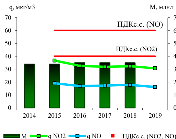
Рис. 3.12. Среднегодовые концентрации диоксида ( q\text{NO}_2 , мкг/м 3 ) и оксида азота ( q\text{NO} , мкг/м 3 ) и суммарные выбросы ( M , млн. т) \text{NO}_x (в пересчете на \text{NO}_2 )
