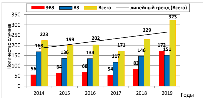
Рис. 4.45. Динамика количества случаев ВЗ и ЭВЗ поверхностных вод Арктической зоны РФ
