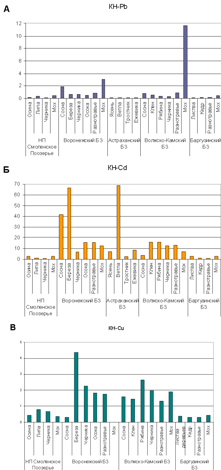
Рис. 2.36. Коэффициенты накопления свинца (А), кадмия (Б) и меди (В) в растениях СКФМ
