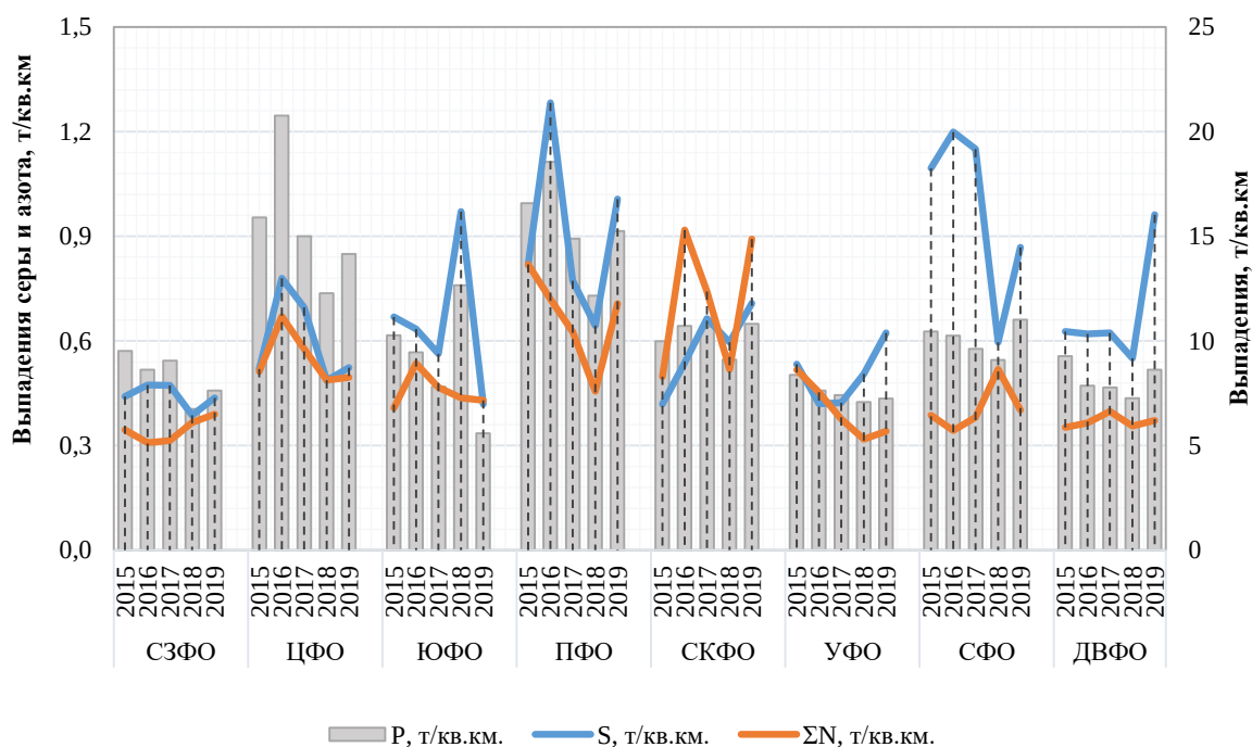
Рис. 2.24. Временной ход средних за год выпадений с осадками серы (S), суммарного азота ( \Sigma N ) и суммы ионов (P) по федеральным округам, 2015-2019 гг.
