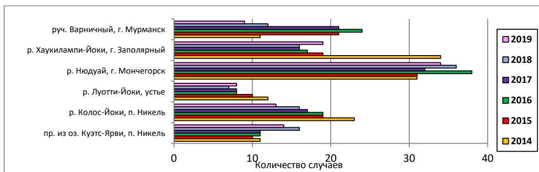
Рис. 4.49. Водные объекты Мурманской обл., на которых регистрировалось максимальное число повторений случаев ВЗ и ЭВЗ за период 2014-2019 гг.
