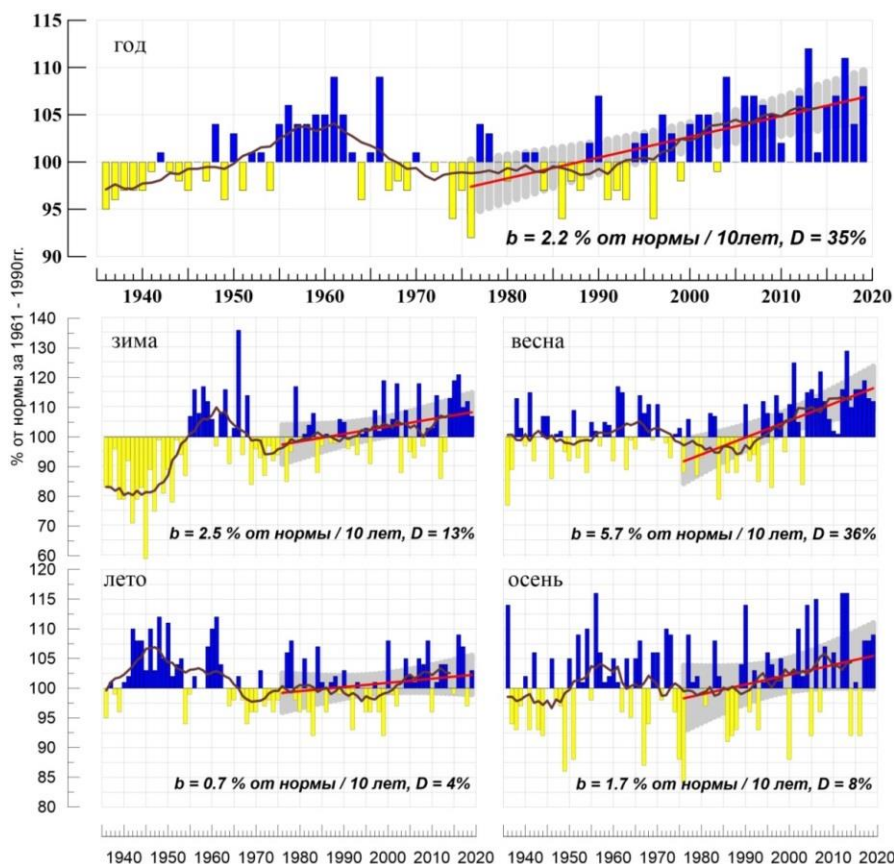
Рис. 1.10. Средние годовые и сезонные осадки (% от нормы), осредненные по территории РФ, 1936-2019гг. Нормы рассчитаны по периоду 1961-1990 гг. Сглаженная кривая получена 11-летним скользящим осреднением. Линейный тренд проведен по данным за 1976-2019 гг.; b - коэффициент тренда (% от нормы / 10 лет), D - вклад в суммарную дисперсию (%).
