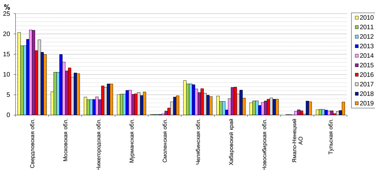
Рис. 3.56. Динамика количества случаев ВЗ и ЭВЗ по субъектам Российской Федерации, в которых регистрировалось наибольшее количество случаев ВЗ и ЭВЗ в 2019 г. (в % от общего количества случаев ВЗ и ЭВЗ на территории Российской Федерации)
