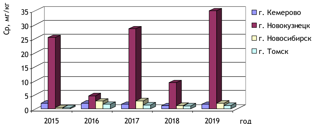
Рис. 3.28. Динамика содержания водорастворимых соединений фтора в почвах городов Западной Сибири
