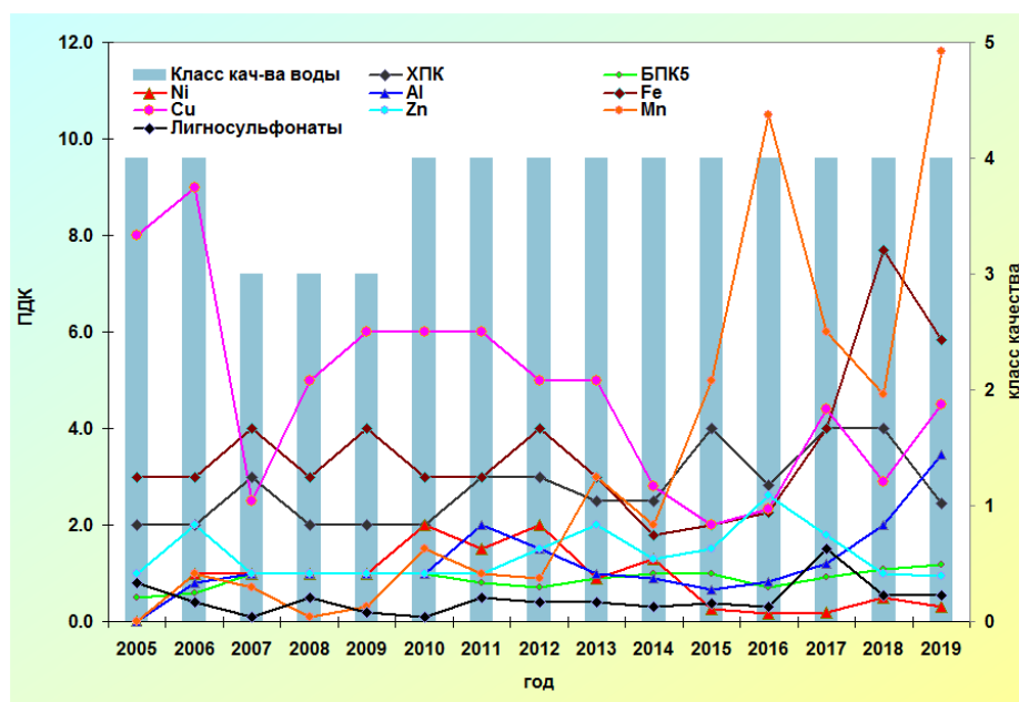
Рис. 3.35. Изменение среднегодовых концентраций отдельных ингредиентов и качества воды р. Северная Двина, г. Красавино, 3,5 км ниже города за многолетний период
