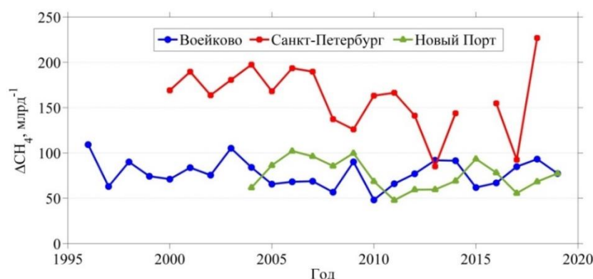
Рис. 2.3. Среднегодовое превышение концентрации CH 4 над фоновым уровнем
