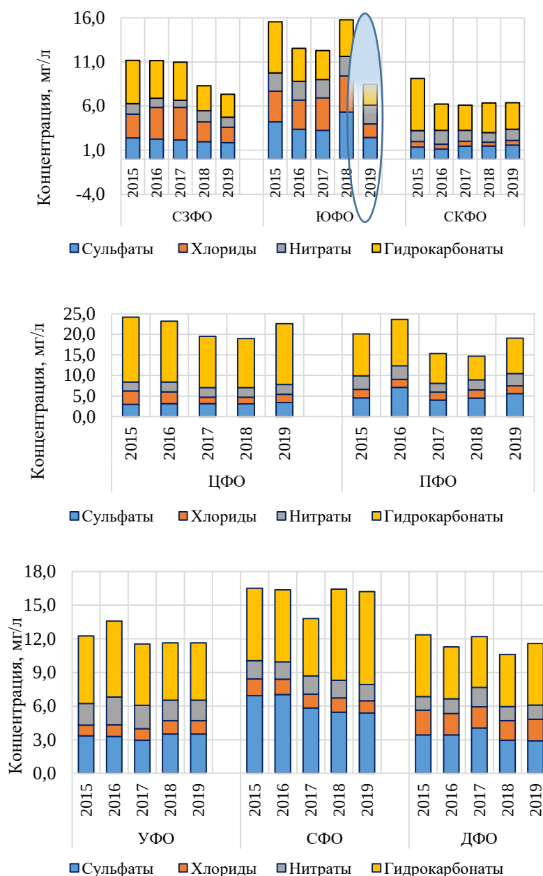
Рис. 2.23. Изменения средневзвешенной концентрации ионов в осадках по федеральным округам, 2015-2019 гг.
