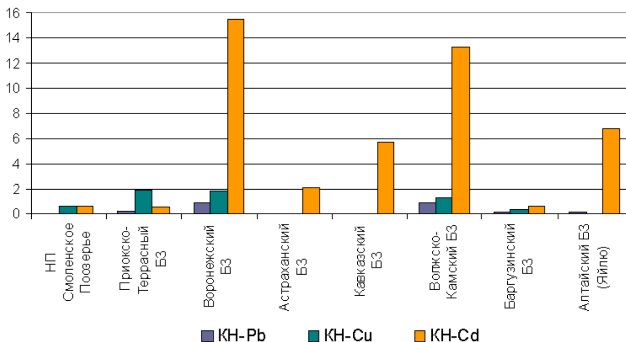
Рис. 2.35. Коэффициенты накопления свинца, кадмия и меди в растительности напочвенного покрова СКФМ
