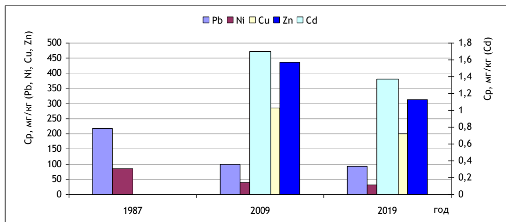
Рис. 3.26. Содержание ТМ в почвах г. Медногорска
