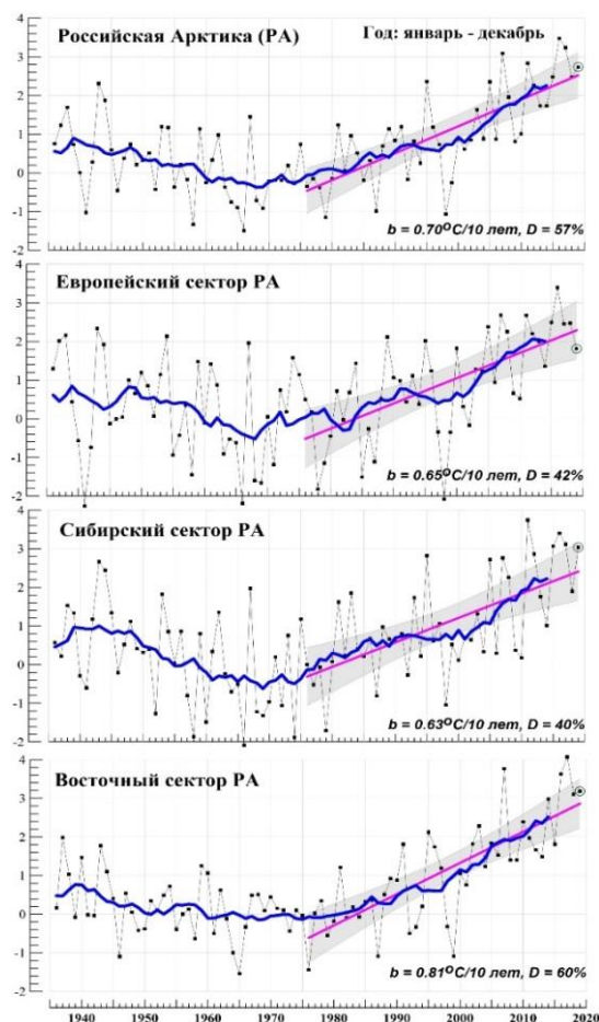
Рис. 4.27. Годовые (январь-декабрь) аномалии температуры воздуха в Российской Арктике и ее секторах в 1936-2019 гг. Жирная синяя кривая - 11летнее скользящее среднее. Показан линейный тренд за 1976-2019 гг.
