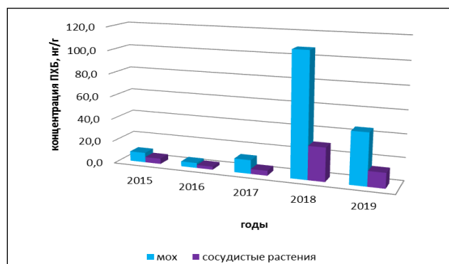
Рис. 4.64. Изменение средних концентраций ПХБ в растительности за период 2015-2019 гг.
