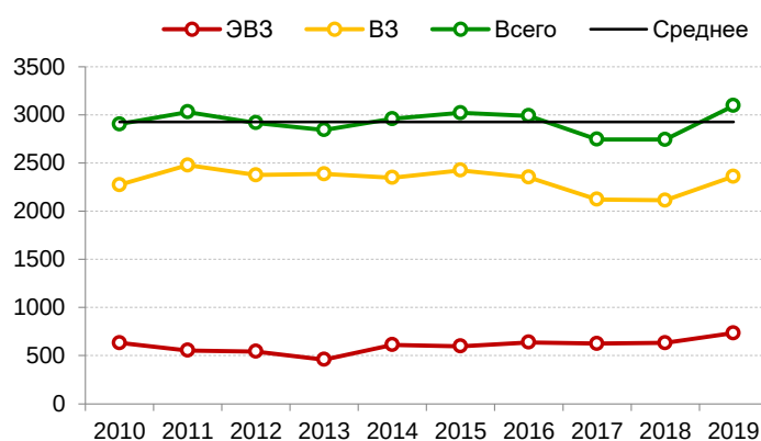
Рис. 3.53. Динамика количества случаев ВЗ и ЭВЗ поверхностных вод суши на территории Российской Федерации
