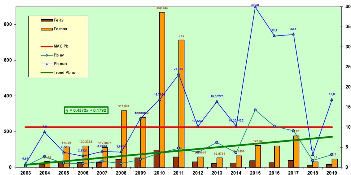
Рис. 3.66. Средняя и максимальная концентрация железа и свинца (мкг/дм 3 ) в прибрежных водах района Адлер-Сочи в 2003-2019 гг. Сокращения: Fe av - средняя концентрация железа; Fe max - максимальная концентрация железа; MAC Pb - ПДК свинца; Pb av - средняя концентрация свинца; Pb max - максимальная концентрация свинца; Trend Pb av - тренд средней концентрации свинца.
