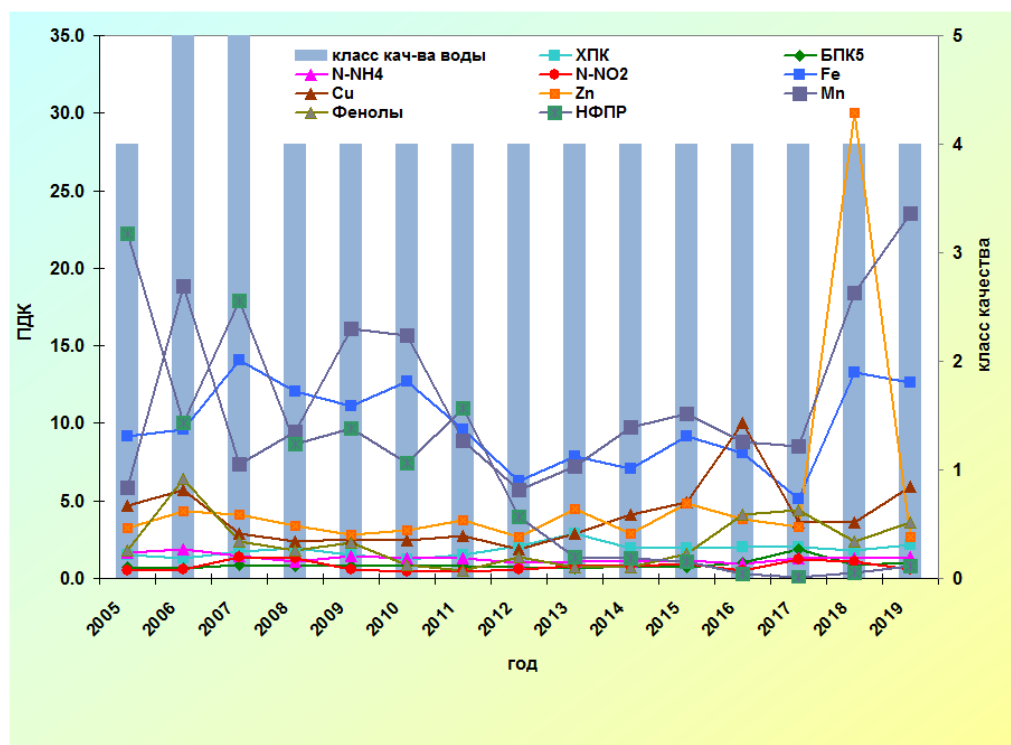
Рис. 3.46. Изменение среднегодовых концентраций отдельных ингредиентов и качества воды р. Обь ниже г. Салехард за многолетний период
