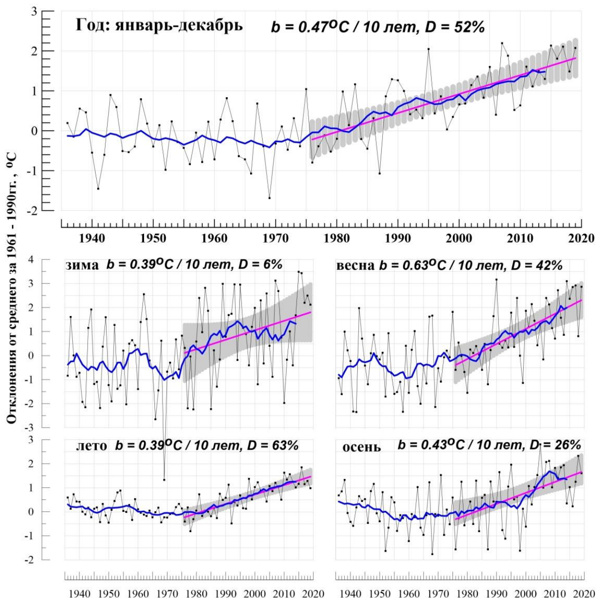
Рис. 1.7. Средние годовые (вверху) и сезонные аномалии температуры приземного воздуха ( ^{\circ}\text{C} ), осредненные по территории РФ, 1936-2019 гг. Аномалии рассчитаны как отклонения от среднего за 1961-1990 гг. Показаны также 11- летнее скользящее среднее, линейный тренд за 1976-2019 гг. с 95%-й доверительной полосой; b - коэффициент тренда ( ^{\circ}\text{C}/10 лет), D - вклад в суммарную дисперсию (%)
