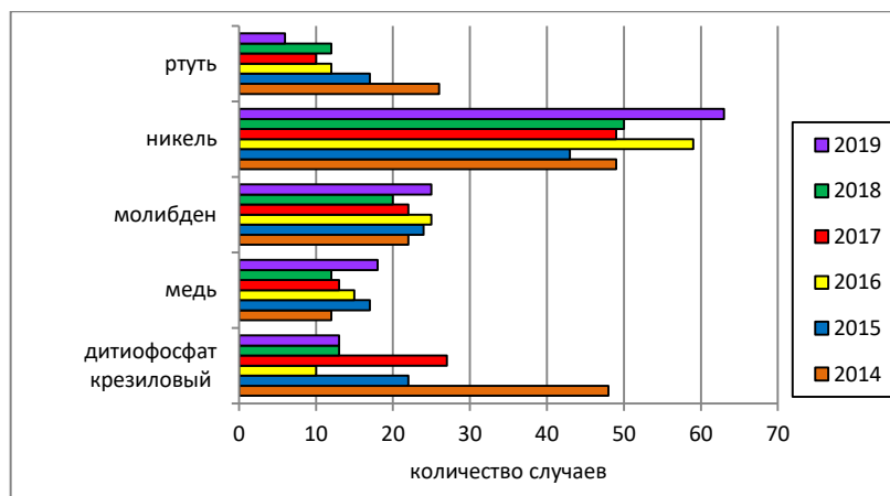
Рис. 4.48. Распределение случаев ВЗ и ЭВЗ по основным загрязняющим веществам в Мурманской обл. за период 2014-2019 гг.
