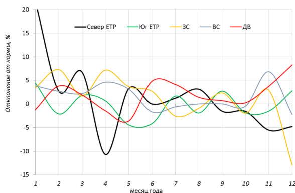
Рис. 2.12. Отклонения среднемесячных значений ОСО от норм по регионам РФ в 2019 г. (Север ЕТР — Север Европейской территории России, Юг ЕТР — Юг Европейской территории России, ЗС — Западная Сибирь, ВС — Восточная Сибирь, ДВ — Дальний восток)
