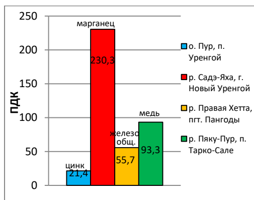
Рис. 4.53. Максимальные ПДК основных загрязняющих веществ в водных объектах Ямало-Ненецкого АО в 2019 г.
