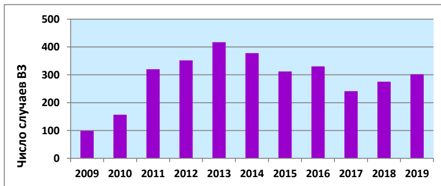
Рис. 4.10. Изменение количество случаев высокого загрязнения водотоков Московского региона
