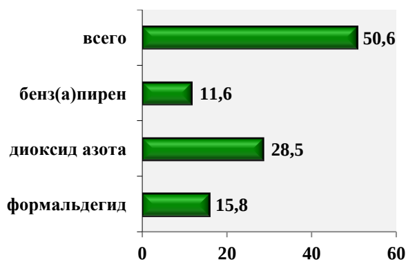
Рис. 3.19. Число жителей в городах (млн.), находящихся под воздействием средних концентраций примесей в воздухе выше 1 ПДК
