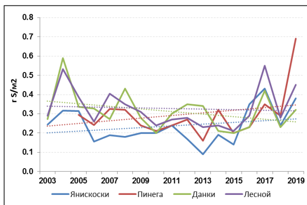
Рис. 2.29. Многолетние выпадения сульфатной серы из атмосферы с осадками на станциях ЕМЕП (г S/m²/год)
