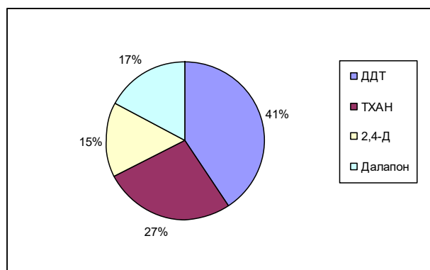
Рис. 3.31. Доля площади, загрязненной различными пестицидами по данным наблюдений в 2019 г.
