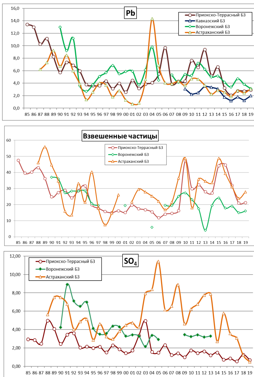
Рис. 2.14. Многолетнее изменение среднегодового содержания свинца (нг/м 3 ), взвешенных частиц и сульфатов
