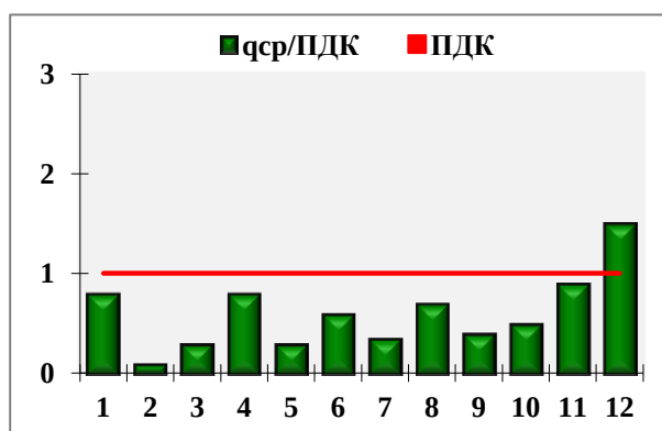
Рис. 3.17. Средние за год концентрации примесей в городах России 1 - взвешенные вещества (229), 2 - диоксид серы (241), 3 - оксид углерода (232), 4 - диоксид азота (244), 5 - оксид азота (177), 6 - сероуглерод (4), 7 - фенол (10), 8 - фторид водорода (30), 9 - хлорид водорода (39), 10 - аммиак (78), 11 - формальдегид (163), 12 - бенз(а)пирен (180). Цифры в скобках указывают количество городов, в которых проводились регулярные наблюдения за данной примесью.
