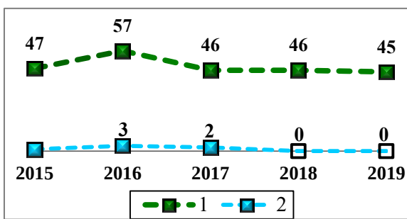
Рис. 3.8. Количество городов, в которых среднегодовые концентрации формальдегида превысили 1 ПДК (1), СИ формальдегида больше 10 (2)
