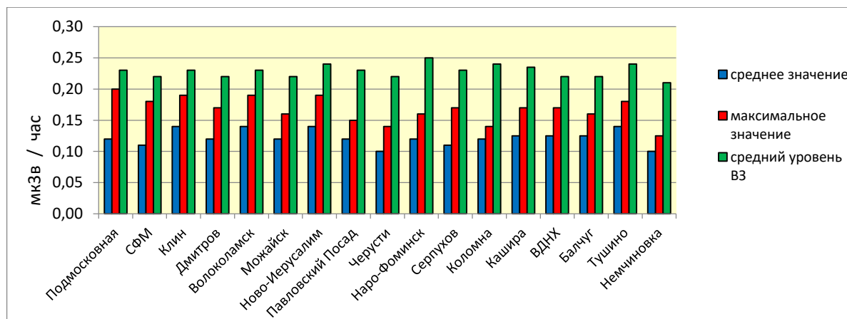
Рис. 4.14. Мощность амбиентного эквивалента дозы гамма-излучения (МАЗД) на станциях Московского региона в 2019 г.
