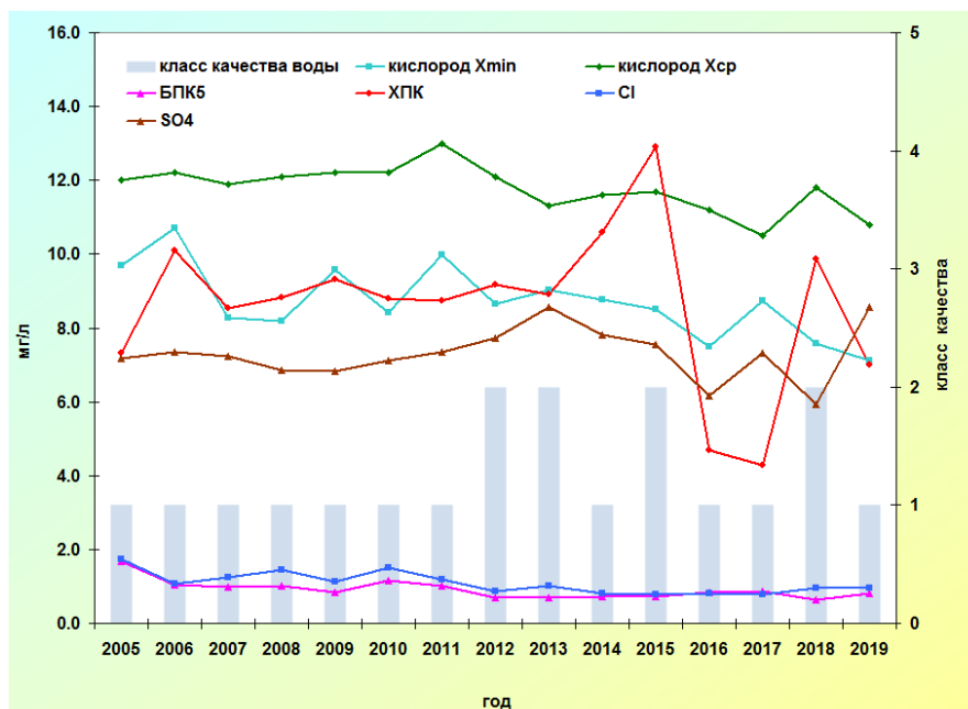
Рис. 2.40. Изменение среднегодовых концентраций отдельных ингредиентов и качества воды Иркутского водохранилища, ОГП-1 Исток Ангары за многолетний период
