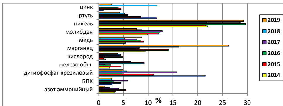
Рис. 4.46. Распределение числа случаев ВЗ и ЭВЗ по ингредиентам (в % от общего количества случаев ВЗ и ЭВЗ Арктической зоны РФ)
