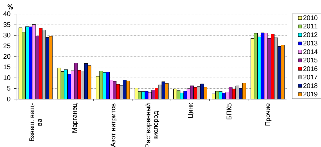
Рис. 3.57. Распределение случаев ВЗ и ЭВЗ поверхностных пресных вод по загрязняющим веществам и показателям качества воды (в % от общего количества случаев ВЗ и ЭВЗ на территории Российской Федерации)
