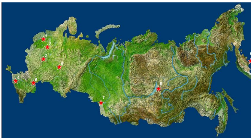
Рис. 2.34. Местоположение СКФМ: 1 - НП Смоленское Поозерье, 2 - Приокско-Террасный БЗ, 3 - Воронежский БЗ, 4 - Кавказский БЗ, 5 - Астраханский БЗ, 6 - Волжско-Камский БЗ, 7 - Алтайский БЗ (Яйлю), 8 - Баргузинский БЗ, 9 - Командорский БР
