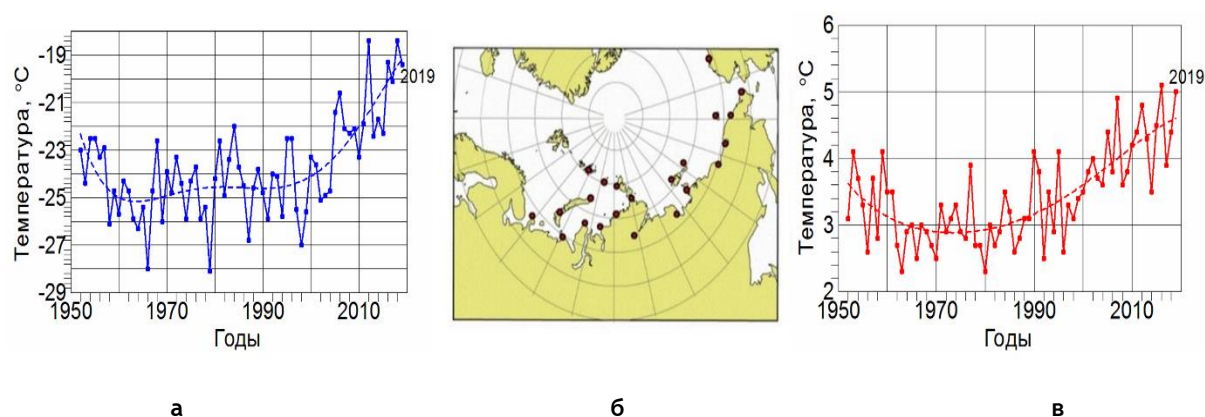
Рис. 4.32. Средняя температура воздуха зимой (а) и летом (в) на акватории арктических морей, по которым проходит трасса СМП по данным 22 метеорологических станций (б)
