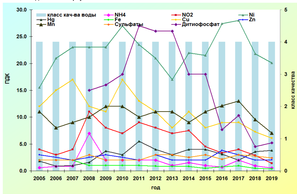
Рис. 3.34. Изменение среднегодовых концентраций отдельных ингредиентов и качества воды р. Хауки-лампи-йоки, г. Заполярный за многолетний период
