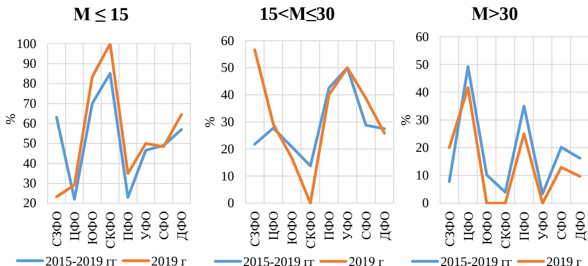
Рис. 2.22. Повторяемость (%) минерализации осадков (M, мг/л) по диапазонам в период с 2015 по 2019 гг.
