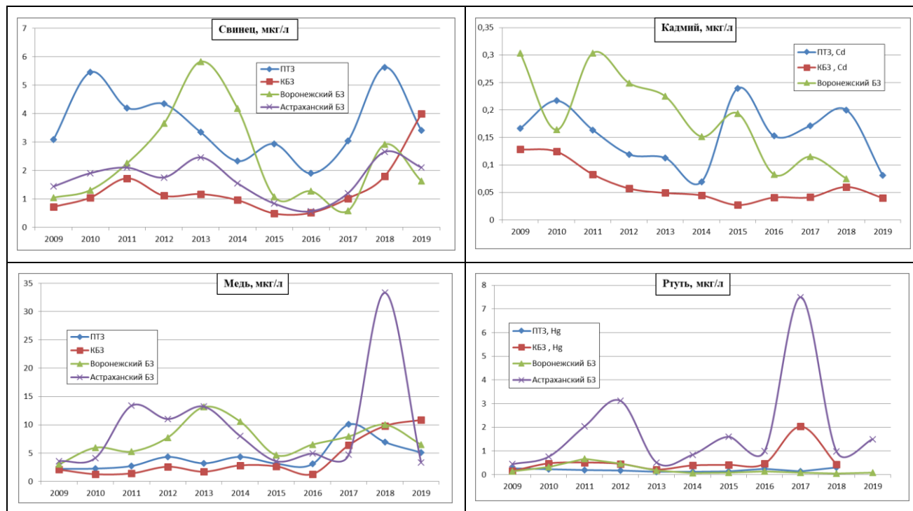
Рис. 2.28. Изменение среднегодового содержания тяжелых металлов в атмосферных осадках фоновых районов в 2009-2019 гг. (геофизические гг.)
