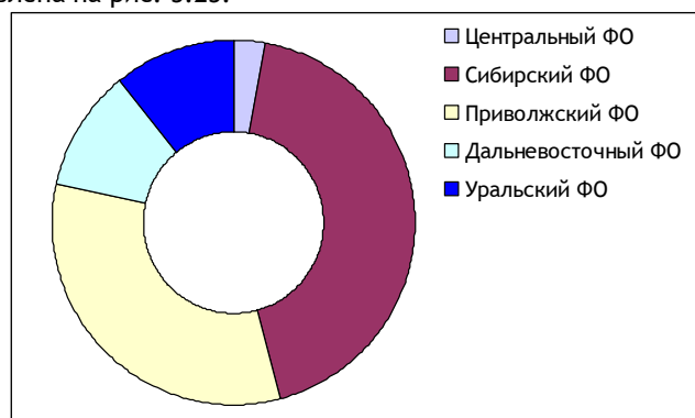
Рис. 3.23. Доля обследованных в 2019 г. населённых пунктов по Федеральным округам
