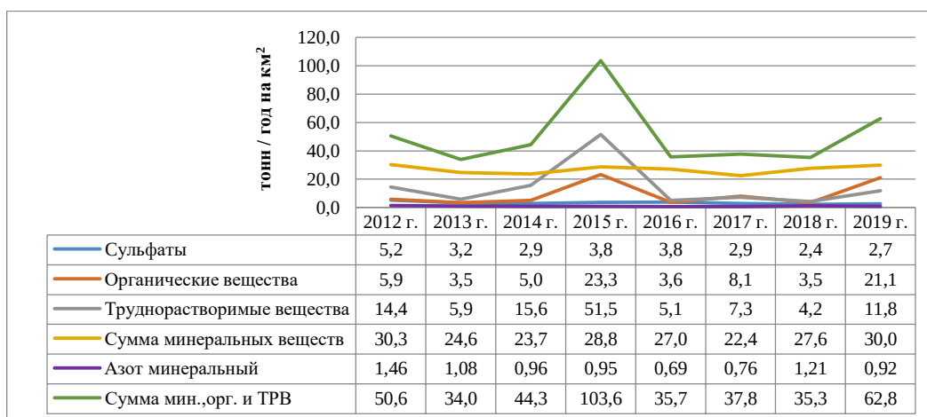
Рис. 4.15. Динамика поступления химических веществ из атмосферы на ст. Хамар-Дабан
