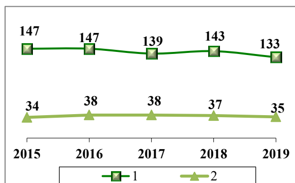
Рис. 3.3. Количество городов, в которых среднегодовые концентрации одного или нескольких веществ превысили 1 ПДК (1) и отмечались значения СИ больше 10 (2)
