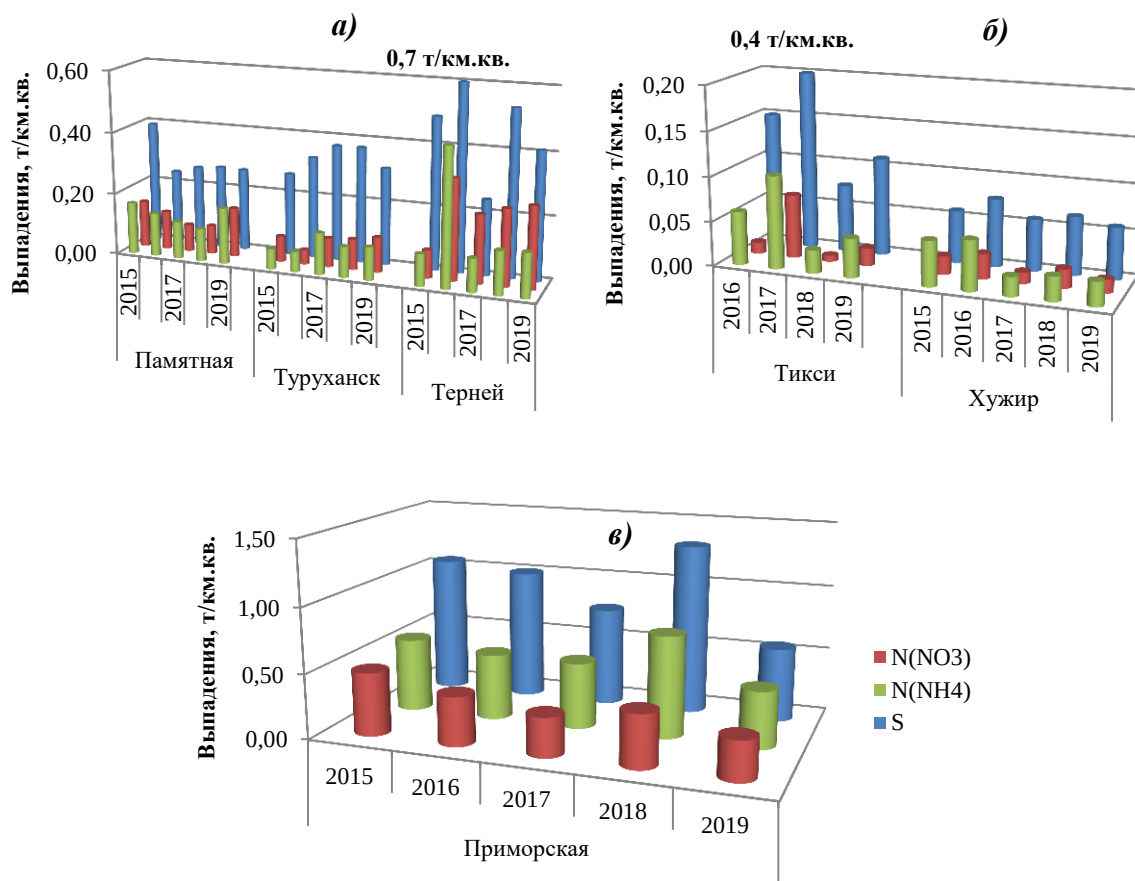
Рис. 2.20. Выпадения серы (S), азота нитратного ( N(NO_3) ) и азота аммонийного ( N(NH_4) ) с атмосферными осадками на АТР в период с 2015 по 2019 гг.
