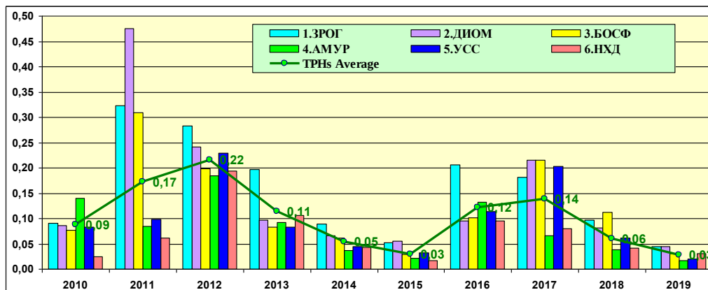
Рис. 3.70. Динамика среднегодовой концентрации нефтяных углеводородов (мг/дм 3 ) в водах различных районов залива Петра Великого Японского моря.
