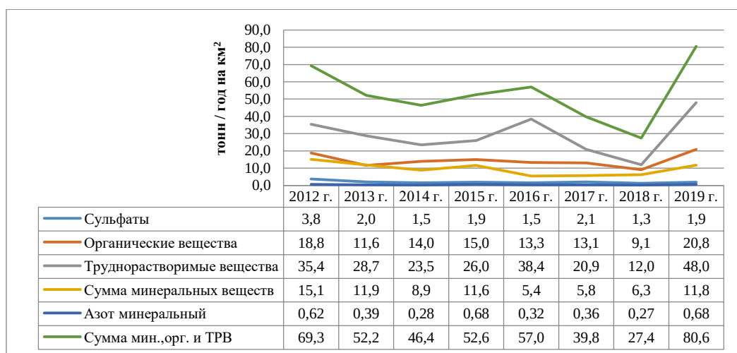
Рис. 4.16. Динамика поступления химических веществ из атмосферы на ст. Байкальск
