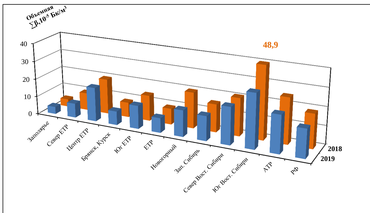
Рис. 2.44. Средние значения объемной \Sigma B в приземном слое атмосферы на территории РФ в 2018-2019 гг., 10^{-5} Бк/м 3
