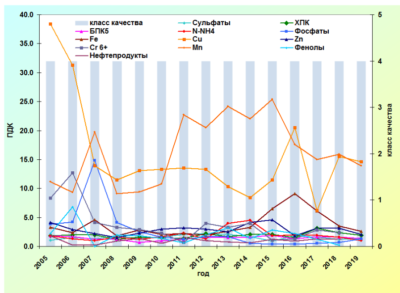
Рис. 3.42. Изменение среднегодовых концентраций отдельных ингредиентов и качества воды р. Чусовая, 1,7 км ниже г. Первоуральск за многолетний период
