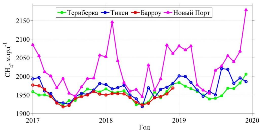
Рис. 4.37. Концентрация \text{CH}_4 для арктических станций РФ в сравнении со станцией Барроу
