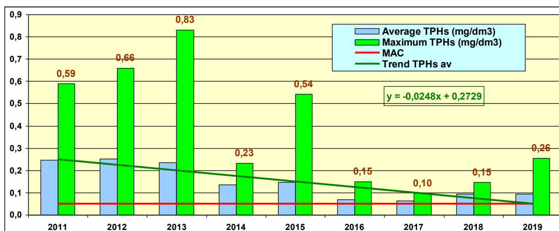
Рис. 3.68. Динамика среднегодового и максимального содержания нефтяных углеводородов (мг/дм³) в торговом порту Мурманска в 2011-2019 гг.
