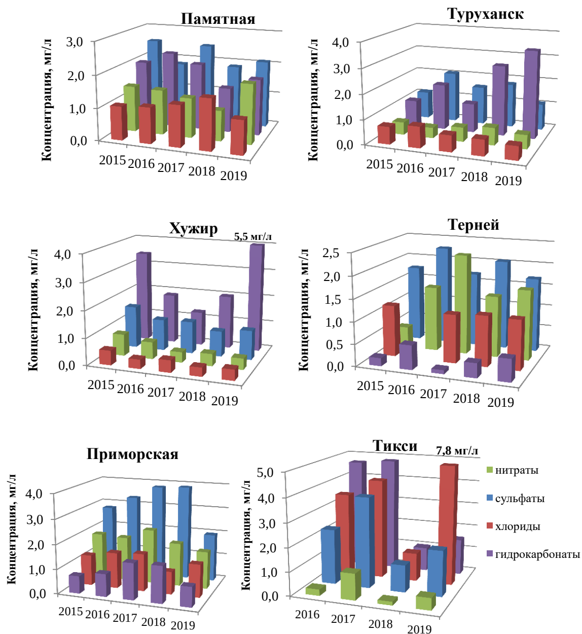
Рис. 2.17. Изменение содержания анионов в атмосферных осадках фоновых станций АТР в период с 2015 по 2019 гг.
