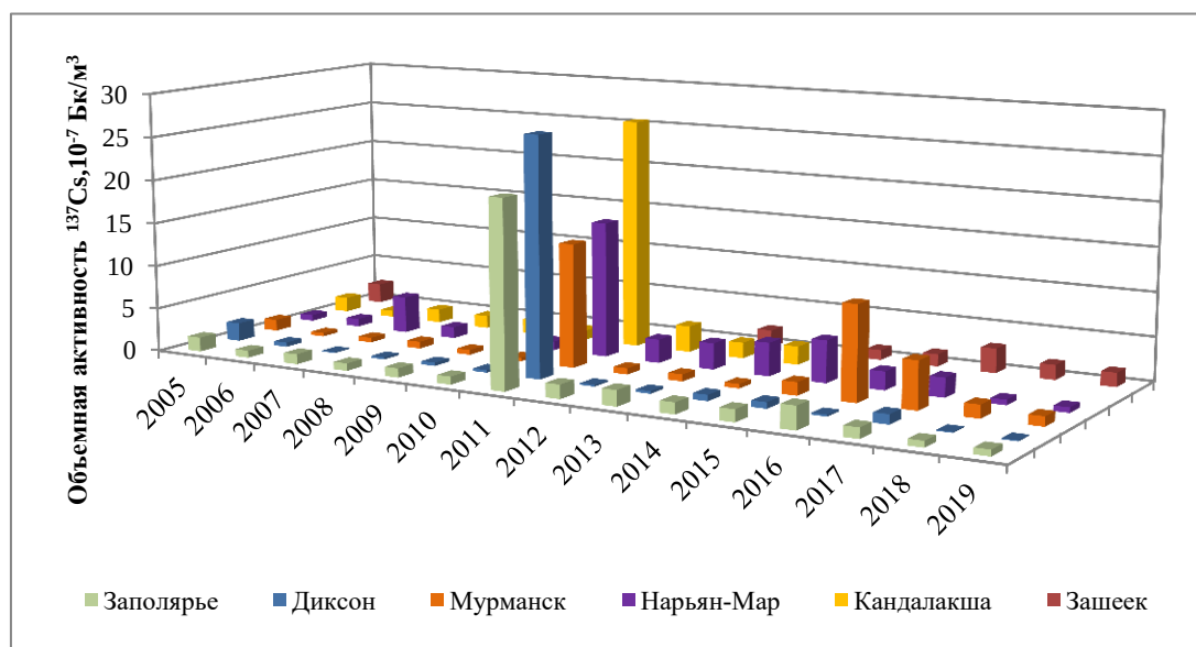
Рис. 4.56. Объемная активность ^{137}\text{Cs} в приземной атмосфере в пунктах наблюдения Сухопутных территорий Арктики и в среднем по Заполярье в 2005-2019 гг., 10^{-7} Бк/м 3
