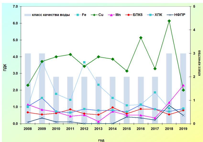
Рис. 2.42. Изменение среднегодовых концентраций отдельных ингредиентов и качества воды р. Правда в створе выше п. Правда за многолетний период
