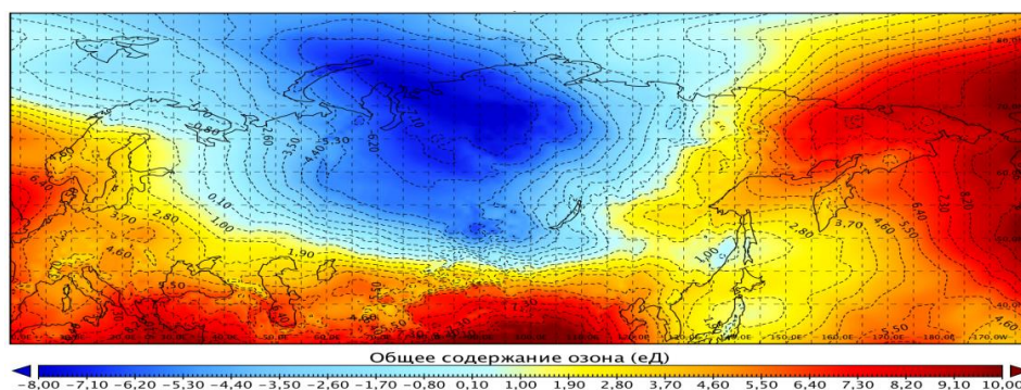
Рис. 2.10. Поле отклонений (%) общего содержания озона в декабре 2019 г. от среднемесячных многолетних значений (1979-1999 гг.)
