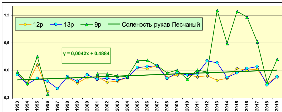
Рис. 3.61. Многолетняя динамика среднегодовой солености в устьевых протоках р. Дон в период 1993-2019 гг.
