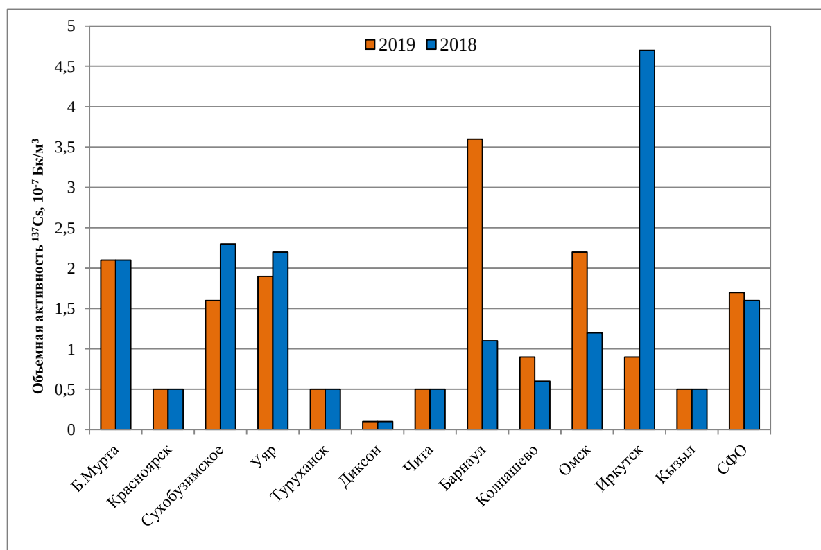
Рис. 2.46. Среднегодовая объемная активность ^{137}\text{Cs} в населенных пунктах СФО
