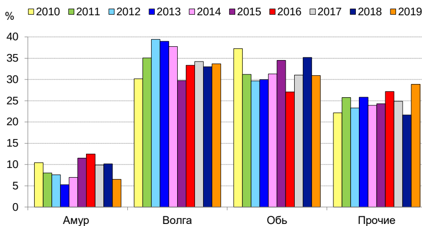
Рис. 3.55. Распределение случаев ВЗ и ЭВЗ по бассейнам рек (в % от общего количества случаев за год на территории Российской Федерации) за период 2010-2019 гг.
