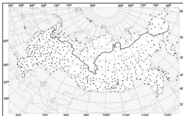
Рис. 4.25. Положение станций архива Т3288 (граница Российской Арктики показана жирной линией)
