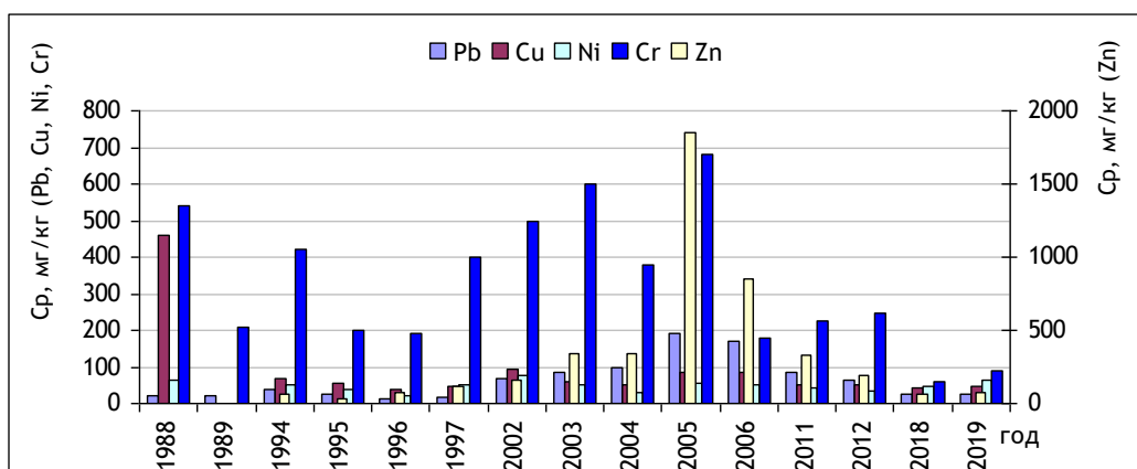
Рис. 3.27. Динамика изменений содержания некоторых ТМ в почвах г. Ижевска
