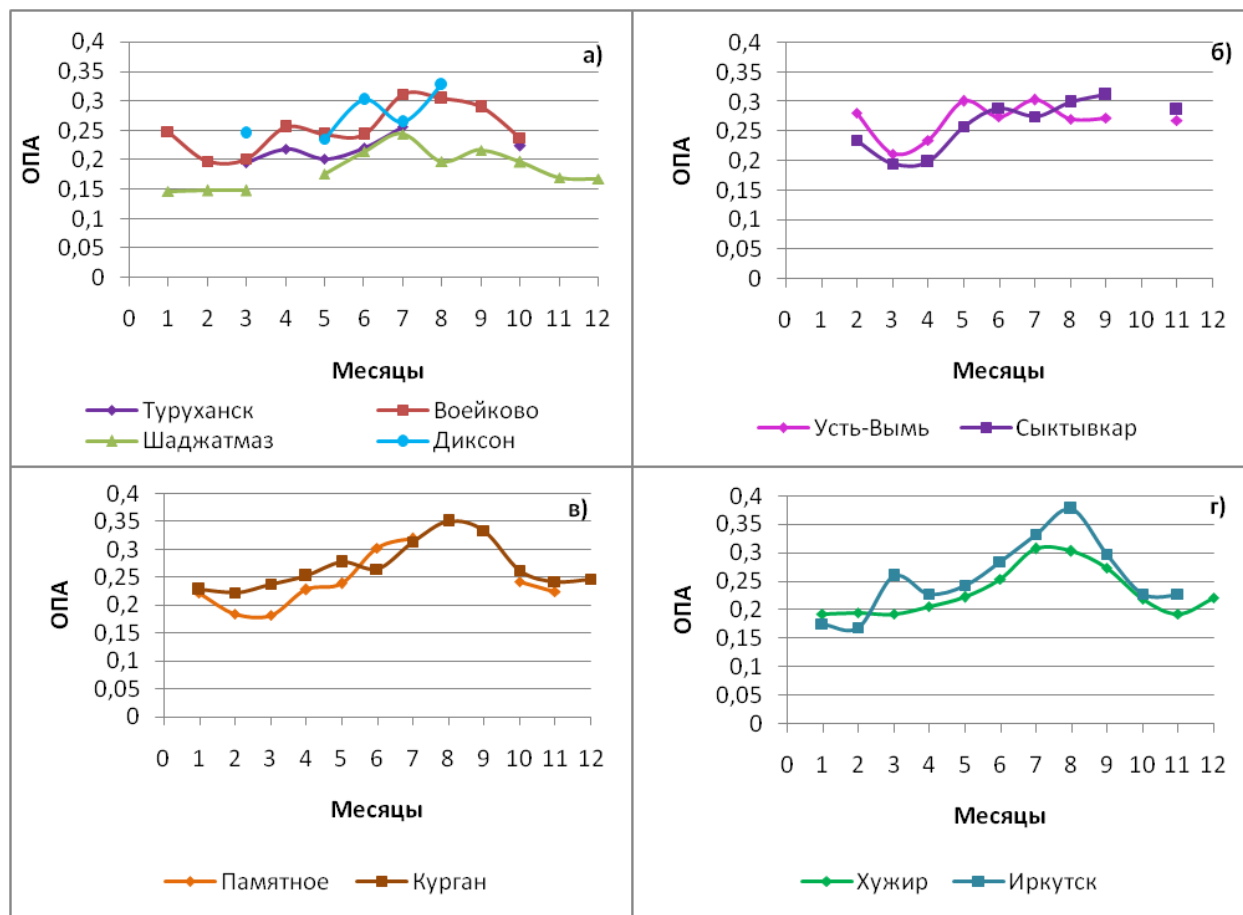
Рис. 2.5. Годовой ход ОПА на станциях фонового мониторинга атмосферы в 2019 г.
