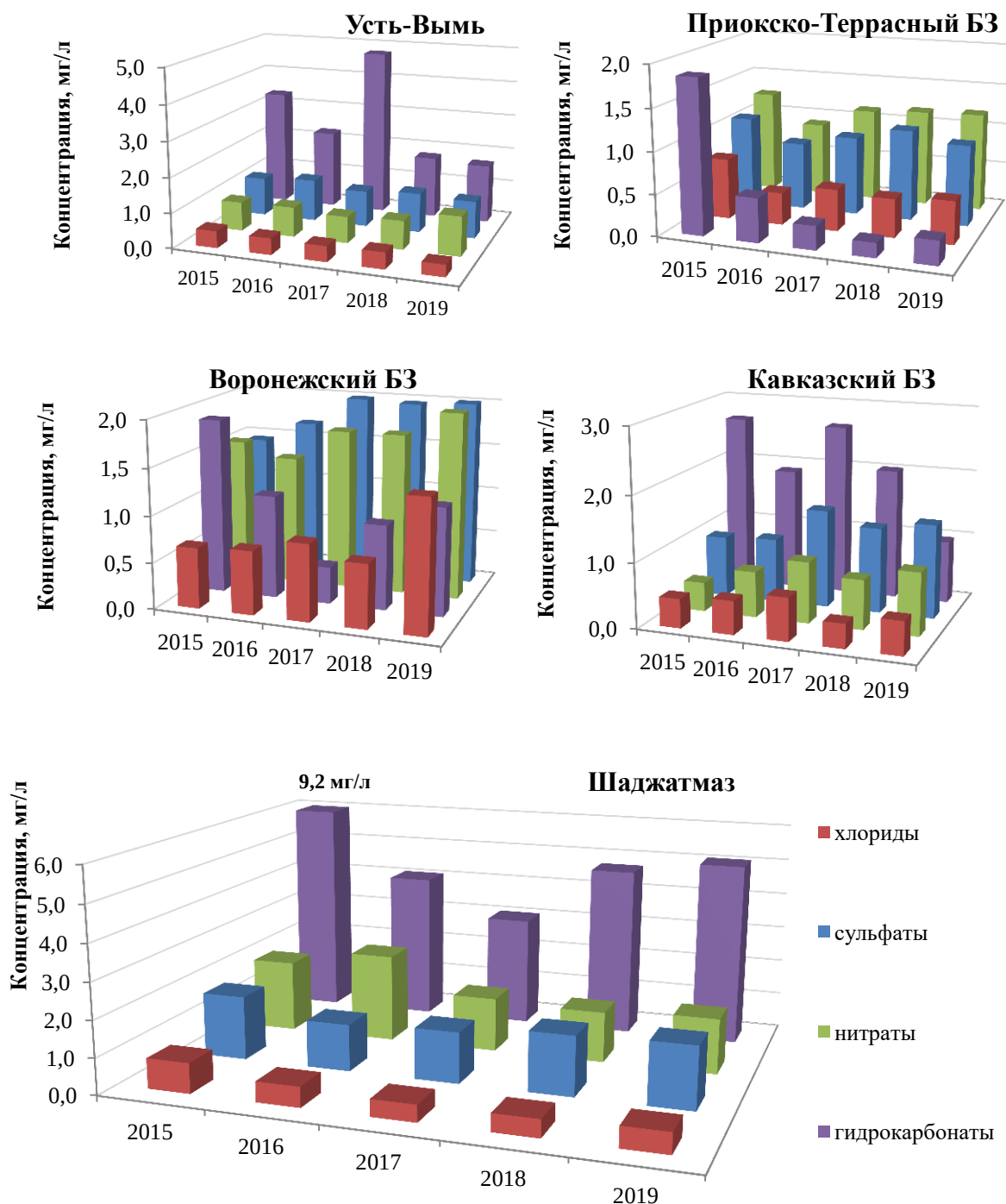
Рис. 2.16. Изменение содержания анионов в атмосферных осадках фоновых станций ЕТР в период с 2015 по 2019 гг.
