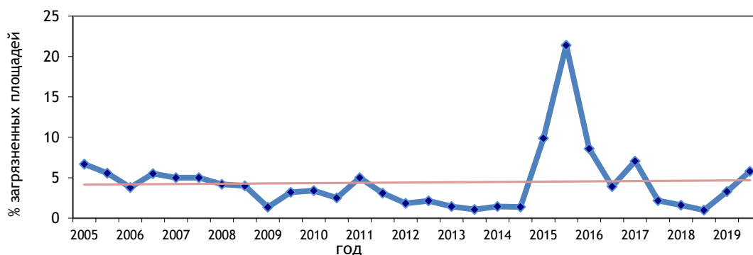
Рис. 3.32. Доля загрязненных почв, % от обследованной площади
