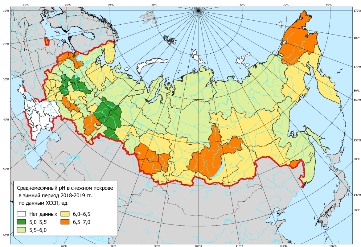
Рис. 2.27. pH снежного покрова в 2019 г.
