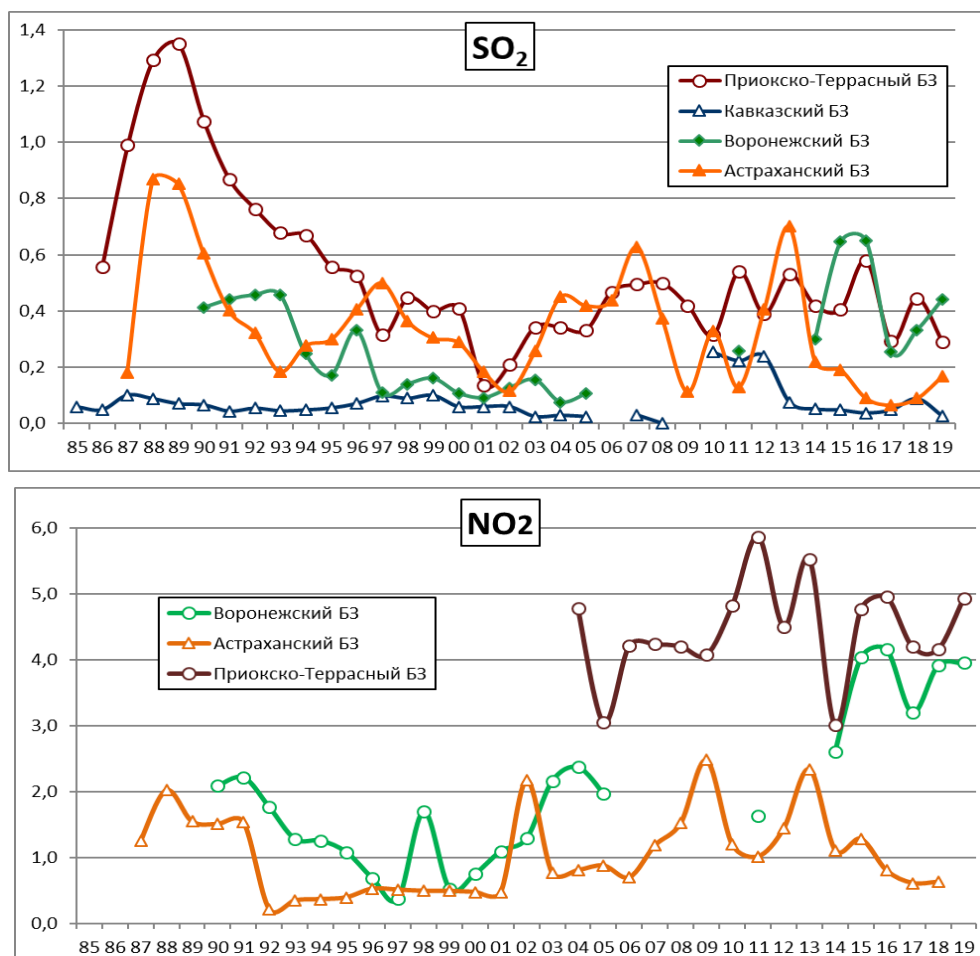
Рис. 2.15. Изменение фоновых концентраций диоксида серы и диоксида азота в атмосферном воздухе фоновых районов (мкг/м 3 ) за многолетний период (геофизические года)
