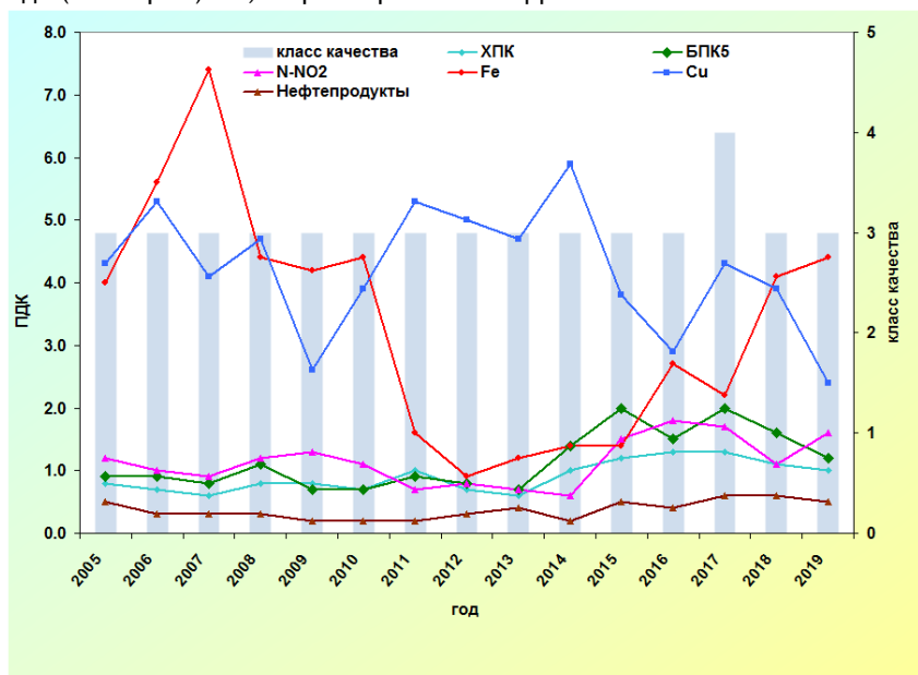
Рис. 3.45. Изменение среднегодовых концентраций отдельных ингредиентов и качества воды р. Кубань, 24,5 км ниже г. Краснодар за многолетний период
