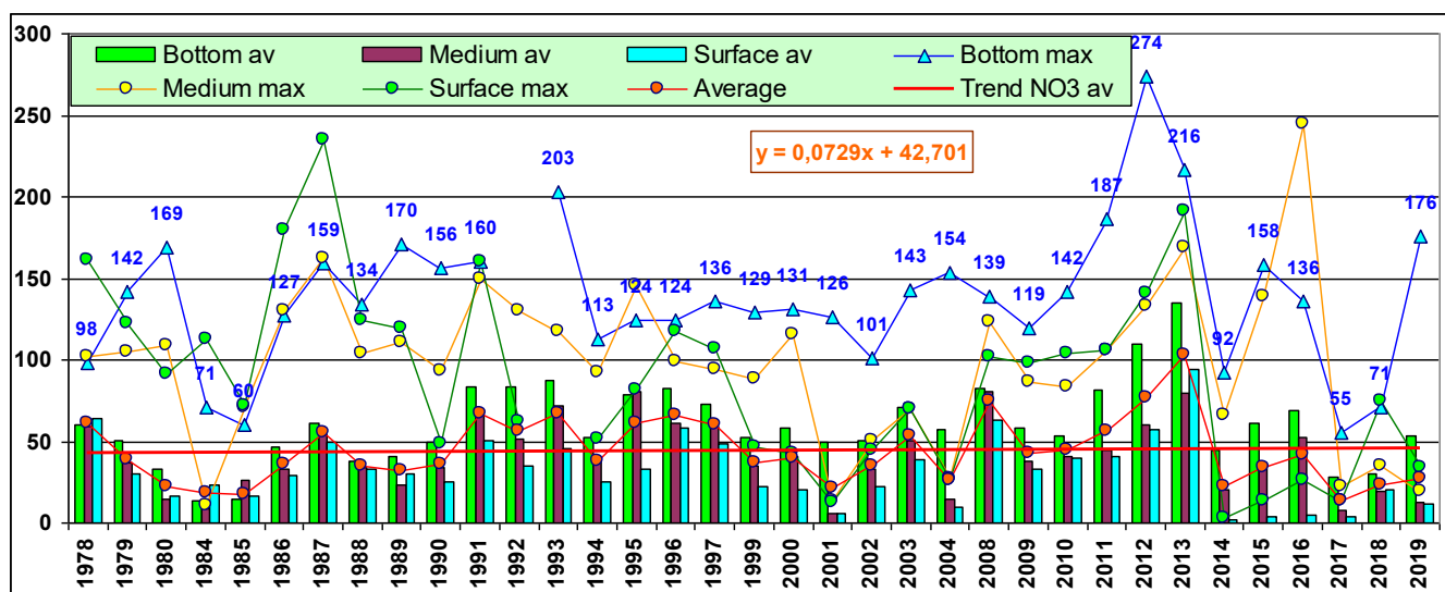
Рис. 3.67. Динамика средней и максимальной концентрации нитратов (мкг/дм³) в поверхностном, промежуточном и придонном слоях в водах Двинского залива Белого моря в 1978-2019 гг.
