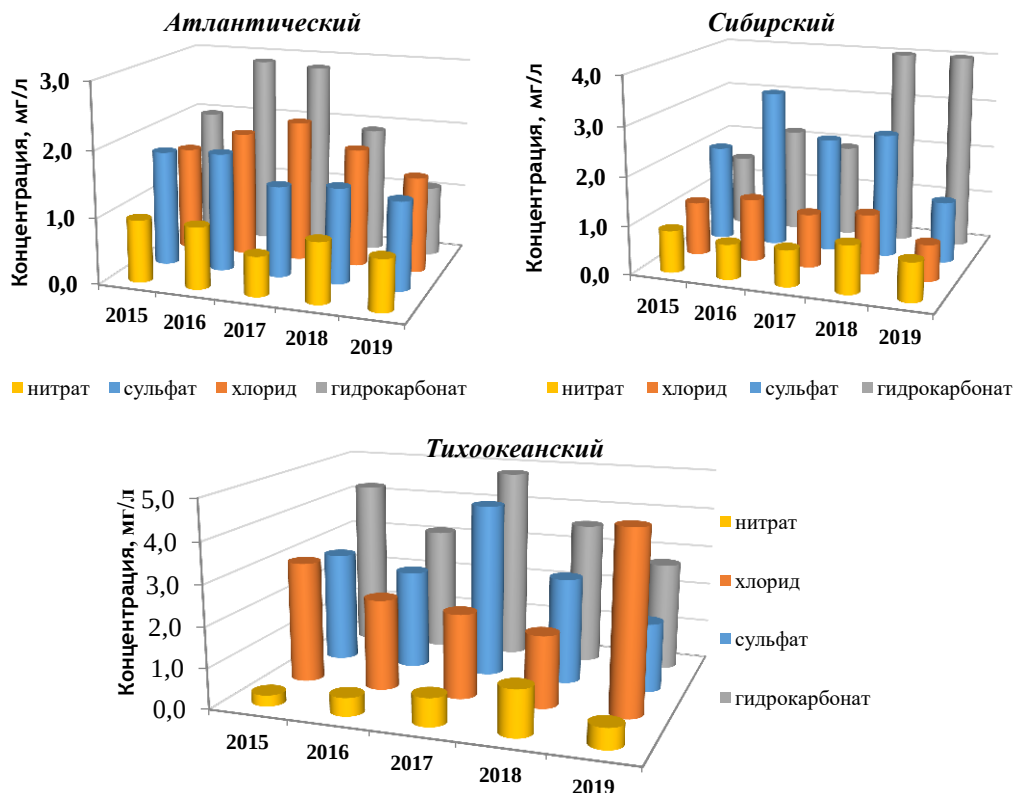
Рис. 4.41. Изменение по секторам концентраций основных ионов в осадках Арктического региона, 2015-2019 гг.
