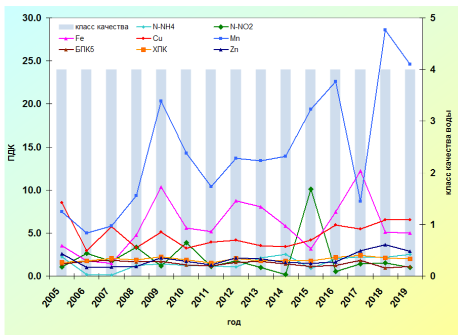
Рис. 3.33. Изменение среднегодовых концентраций отдельных ингредиентов и качества воды р. Охта, 0,05 км выше устья, в черте г. Санкт-Петербург
