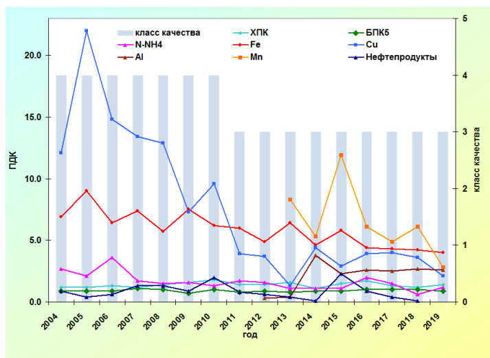
Рис. 3.51. Изменение среднегодовых концентраций отдельных ингредиентов и качества воды р. Амур, в пункте г. Амурск за многолетний период
