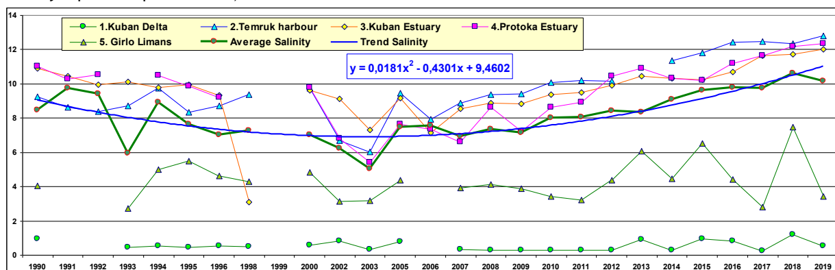
Рис. 3.63. Динамика среднегодовой солености (‰) в различных районах устьевой области р. Кубань и Темрюкском заливе в 1990-2019 гг.
