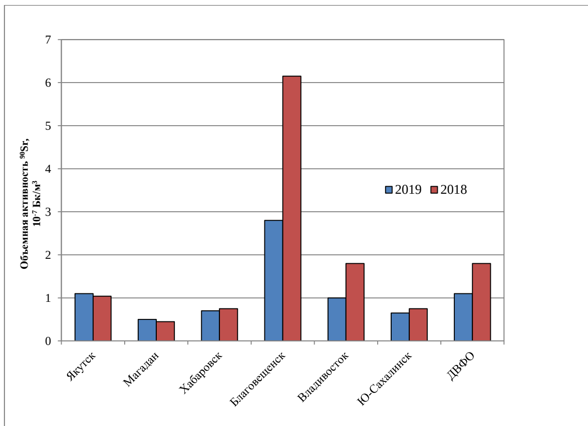
Рис. 2.47. Среднегодовая объемная активность ^{90}\text{Sr} в населенных пунктах ДВФО
