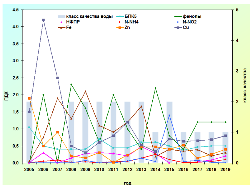
Рис. 2.39 (окончание). Изменение среднегодовых концентраций отдельных ингредиентов и качества воды а) р. Голоустная, б) р. Бугульдейка, в) р. Сарма, г) р. Мантуриха, д) р. Мысовка за многолетний период
