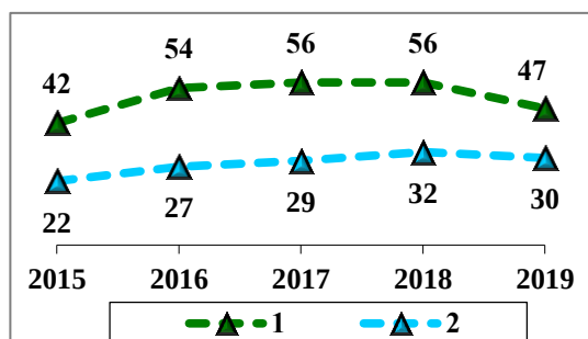
Рис. 3.7. Количество городов, в которых среднегодовые концентрации бенз(а)пирена превысили 1 ПДК (1), СИ бенз(а)пирена больше 10 (2)
