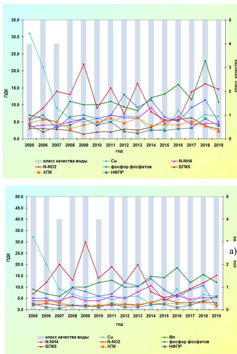
Рис. 3.48. Изменение среднегодовых концентраций отдельных ингредиентов и качества воды р. Исеть а) 7 км ниже г. Екатеринбург, б) 19,1 км ниже г. Екатеринбург за многолетний период
