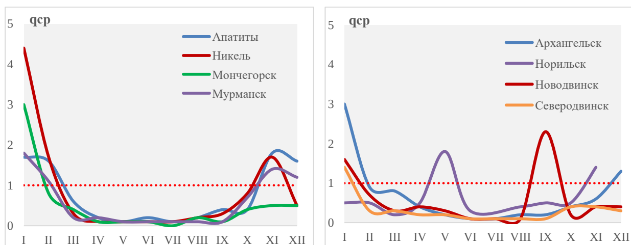
Рис. 4.44. Годовой ход бенз(а)пирена в городах АЗРФ в 2019 г., q_{ср}, нг/м³
