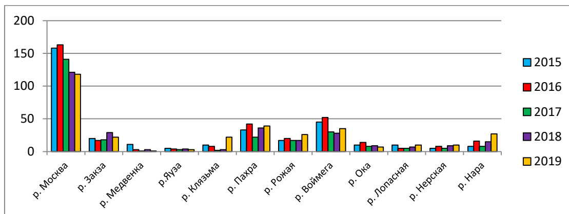
Рис. 4.11. Распределение случаев высокого загрязнения по водотокам Московского региона
