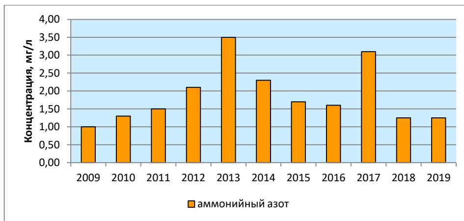
Рис. 4.9. Изменение среднегодовых концентраций аммонийного азота в целом по водным объектам Московского региона
