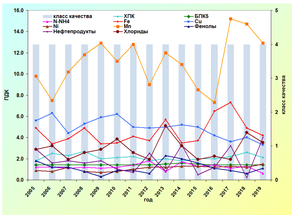
Рис 3.43. Изменение среднегодовых концентраций отдельных ингредиентов и качества воды р. Белая, 10,5 км ниже г. Стерлитамак за многолетний период
