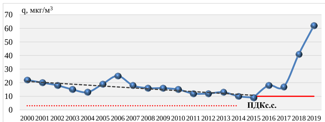
Рис. 3.21. Средние за год концентрации (q, мкг/м 3 ) формальдегида в Южно-Сахалинске за период 2000-2019 гг.
