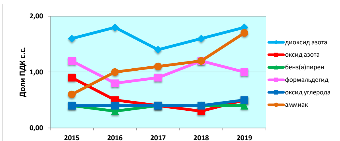
Рис. 4.4. Изменение среднегодовых концентрации примесей в атмосферном воздухе г. Москвы
