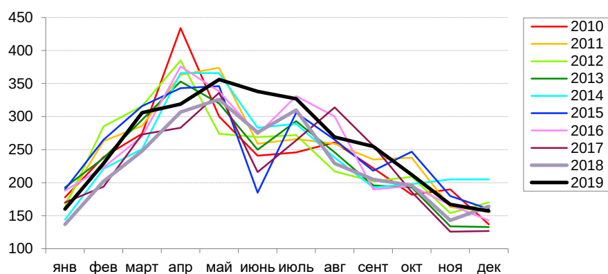
Рис. 3.54. Динамика внутригодового распределения количества случаев ВЗ и ЭВЗ поверхностных вод суши на территории Российской Федерации за период 2010-2019 гг.
