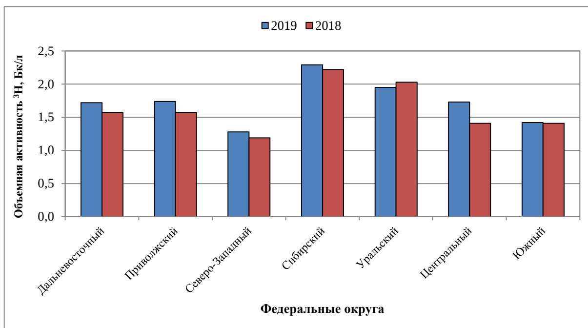
Рис. 2.48. Среднегодовая объемная активность ^3\text{H} в атмосферных осадках
