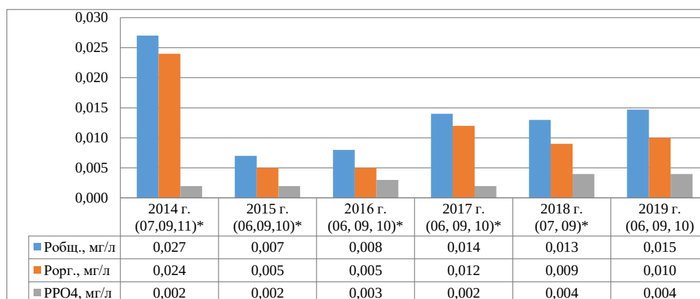
Рис. 4.21. Содержание форм фосфора в воде озера в районе продольного разреза (*-месяц отбора проб)
