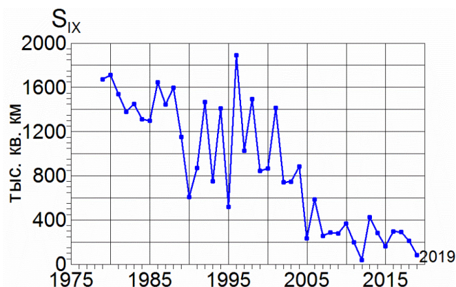
Рис. 4.33. Площадь, занятая морским льдом в сентябре в Сибирских арктических морях (моря Карское, Лаптевых, Восточно-Сибирское, Чукотское) по данным отдела ледовых прогнозов ААНИИ
