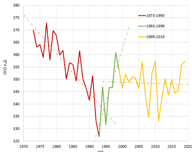
Рис. 2.11. Среднегодовые значения ОСО над территорией РФ в период 1973-2019 гг. Вариации поля ОСО над регионами РФ в 2019 г.
