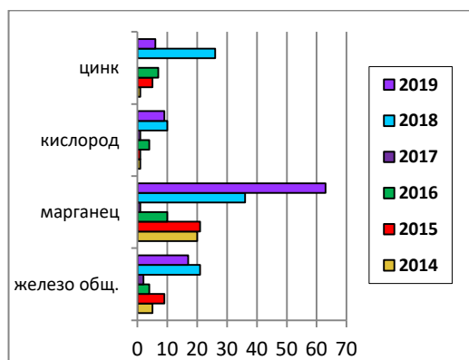
Рис. 4.52. Распределение случаев ВЗ и ЭВЗ по основным загрязняющим веществам в Ямало-Ненецком АО за период 2014-2019 гг.
