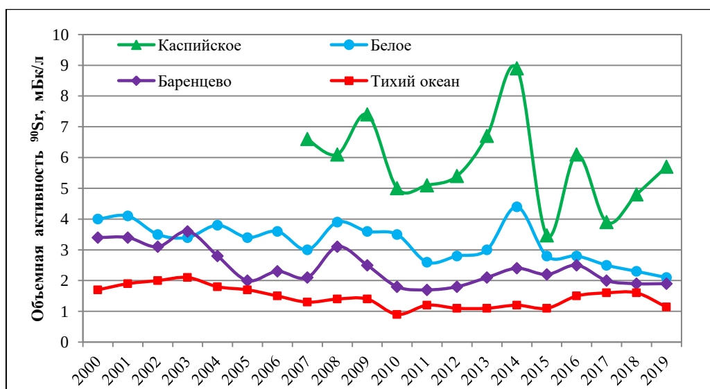
Рис. 4.59. Динамика объемной активности ^{90}\text{Sr} в прибрежных водах Белого и Баренцева морей в сравнении с водами Каспийского моря и Тихого океана вблизи восточного побережья Камчатки в 2000-2019 гг., мБк/л
