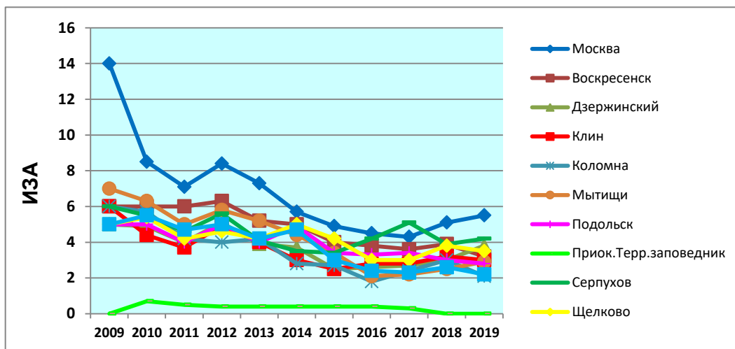
Рис. 4.2. Уровни загрязнения атмосферного воздуха в Московском регионе
