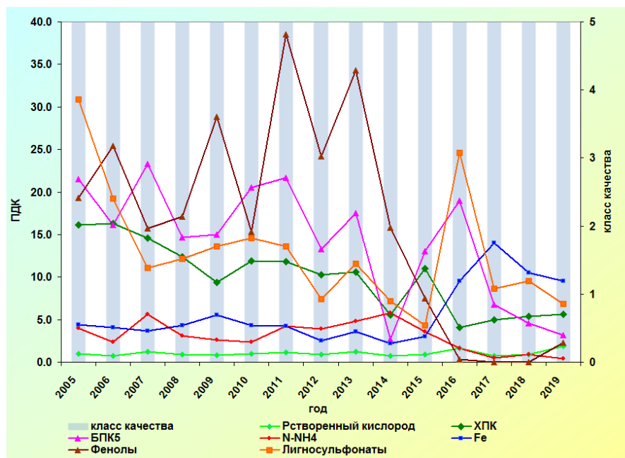
Рис. 3.36. Изменение среднегодовых концентраций отдельных ингредиентов и качества воды р. Пельшма, г. Сокол за многолетний период
