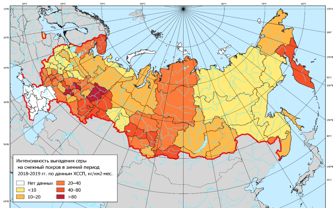
Рис. 2.25. Интенсивность выпадения серы на снежный покров в 2019 г.
