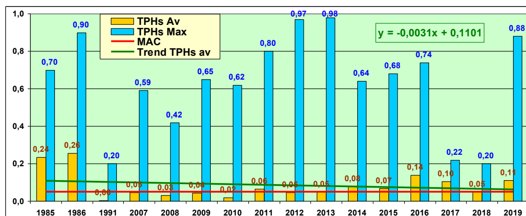
Рис. 3.69. Средняя и минимальная концентрация нефтяных углеводородов (мг/дм³) в водах Авачинской губы на Камчатке в 1985-2019 гг.
