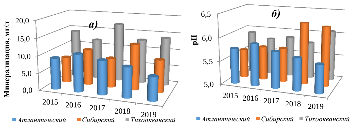
Рис. 4.40. Изменение средневзвешенной минерализации (а) и pH (б) осадков Арктического региона, 2015-2019 гг. Примечание: данные по Атлантическому региону рассчитаны без ст. Мурманск и Никель, по Сибирскому без ст. Норильск и Диксон, а по Тихоокеанскому без ст. Кюсю
