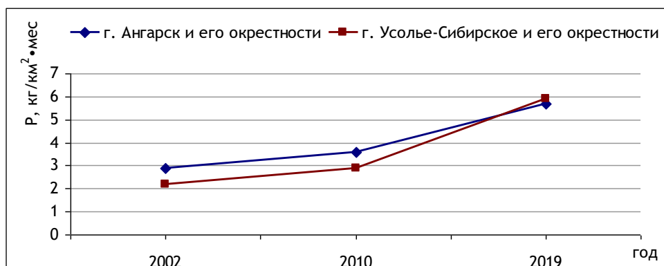
Рис. 3.29. Плотность атмосферных выпадений соединений фтора (Р, кг/км 2 ·мес) по данным обследования снежного покрова в городах Ангарск и Усолье-Сибирское Иркутской области
