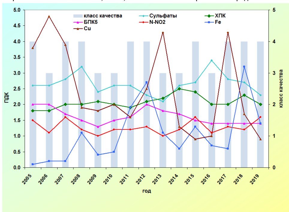
Рис. 3.44. Изменение среднегодовых концентраций отдельных ингредиентов и качества воды р. Дон, ниже г. Ростов-на-Дону за многолетний период
