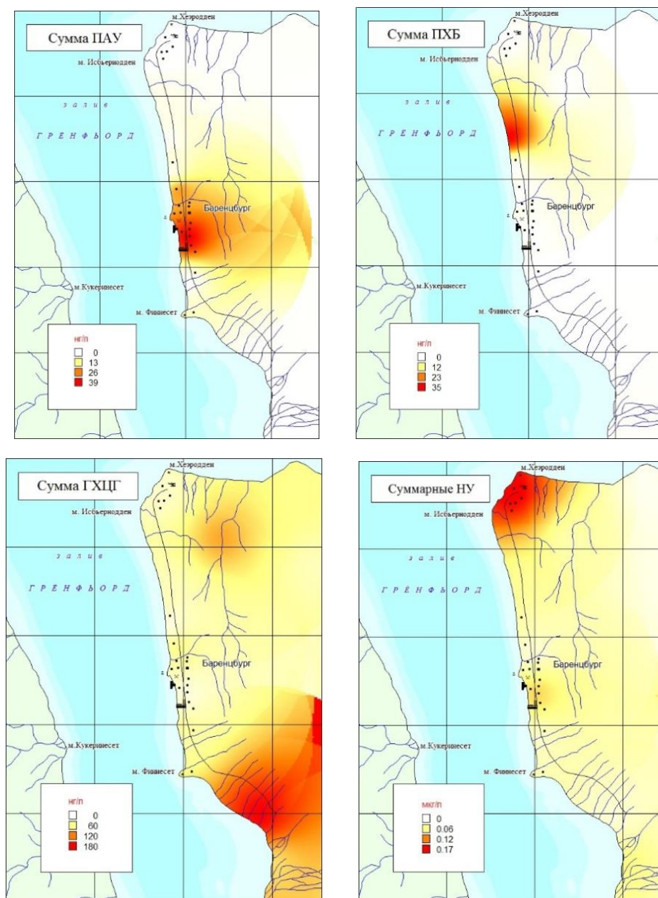
Рис. 4.61. Распределение содержания суммы ПАУ, суммы ПХБ, суммы ГХЦГ и суммарных нефтепродуктов в пробах талого снега в 2019 г.
