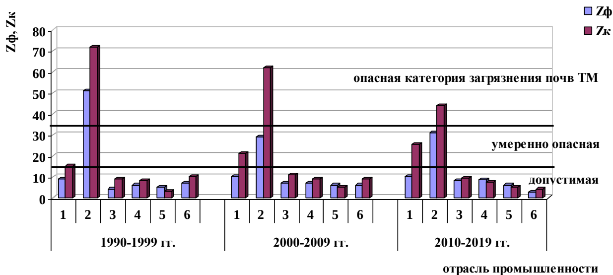
Рис. 3.24. Динамика усреднённых за несколько лет показателей загрязнения почв комплексом ТМ Z_f и Z_k вокруг предприятий черной металлургии (1), цветной металлургии (2), машиностроения и металлообработки (3), топливной и энергетической промышленности (4), химической и нефтехимической промышленности (5), строительной промышленности и производства стройматериалов (6)
