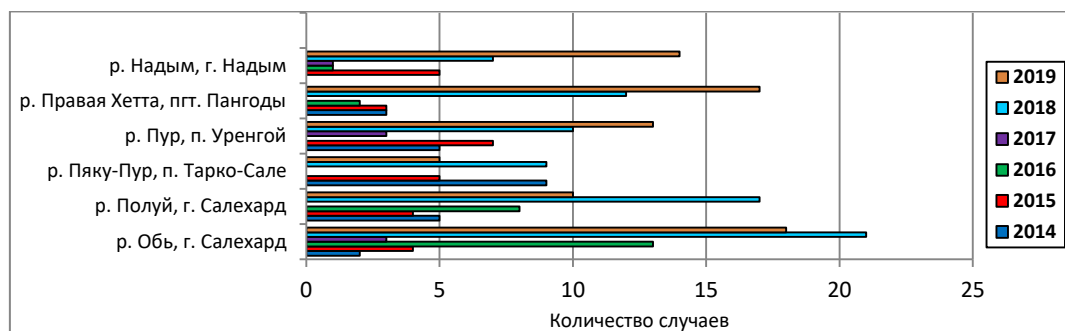
Рис. 4.51. Водные объекты Ямало-Ненецкого АО, в которых регистрировалось максимальное число повторений случаев ВЗ и ЭВЗ за период 2014-2019 гг.
