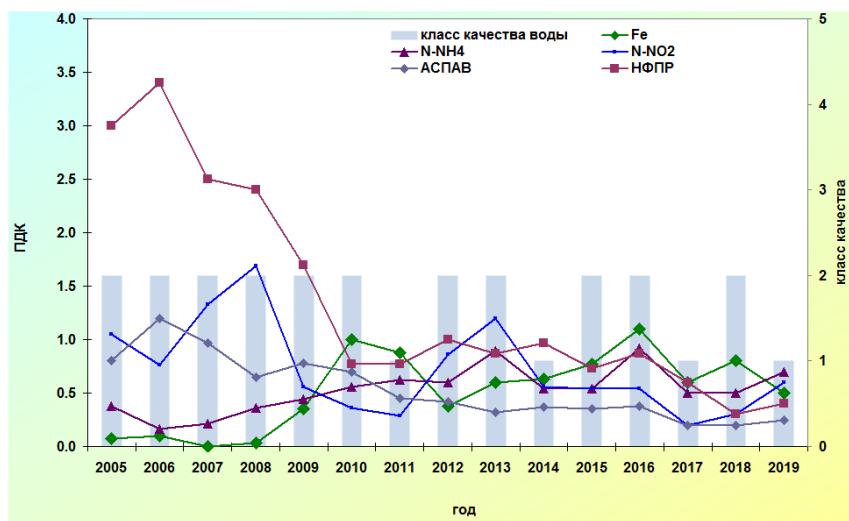
Рис. 2.38 (окончание). Изменение среднегодовых концентраций отдельных ингредиентов и качества воды р. Лесной Воронеж выше г. Мичуринск за многолетний период
