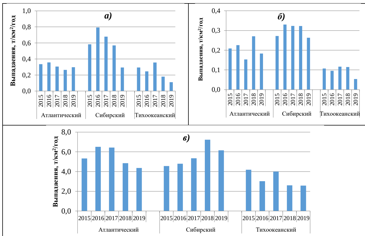
Рис. 4.42. Межгодовой ход влажных выпадений серы (а), суммарного азота (б) и суммы ионов (в) на территории Арктики Примечание: данные по Атлантическому региону рассчитаны без ст. Мурманск и Никель, по Сибирскому без ст. Норильск и Диксон, а по Тихоокеанскому без ст. Кюсюр
