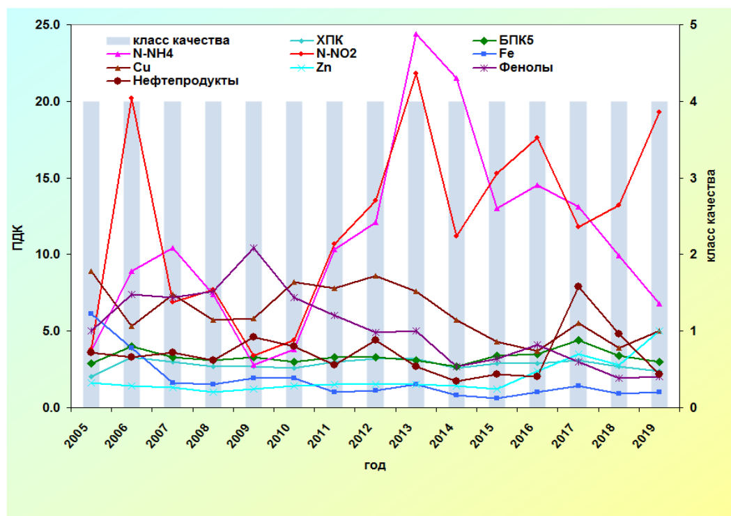
Рис. 3.40. Изменение среднегодовых концентраций отдельных ингредиентов и качества воды р. Москва, г. Москва выше Бесединского моста МКАД за многолетний период
