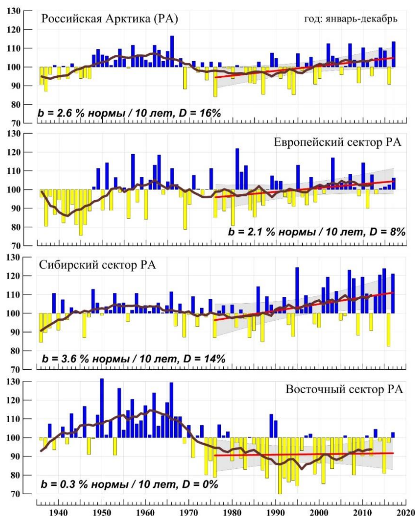
Рис. 4.31. Годовые (январь-декабрь) суммы осадков (% нормы) в Российской Арктике и ее секторах в 1936-2019 гг. Жирная черная кривая - 11летнее скользящее среднее. Показан линейный тренд за 1976-2019 гг.
