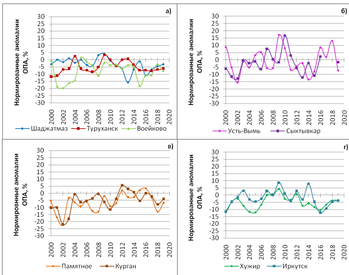
Рис. 2.6. Межгодовая изменчивость нормированных аномалий ОПА (%) на станциях фонового мониторинга
