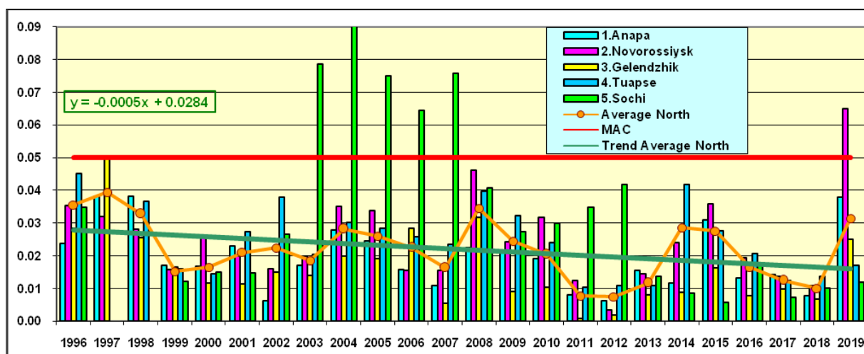
Рис. 3.64. Динамика средней концентрации нефтяных углеводородов ( \text{мг/дм}^3 ) в прибрежных водах Кавказа в 1996-2019 гг. Сокращения: Average North - средняя величина в северной части Кавказского побережья; МАС - предельно допустимая концентрация; Trend Average North - тренд концентрации НУ в северной части побережья.
