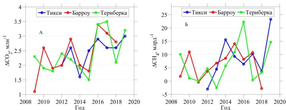
Рис. 2.1. Межгодовые изменения концентрации \text{CO}_2 (А) и \text{CH}_4 (Б)
