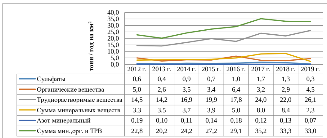
Рис. 4.19. Поступление веществ из атмосферы на ст. Хужир
