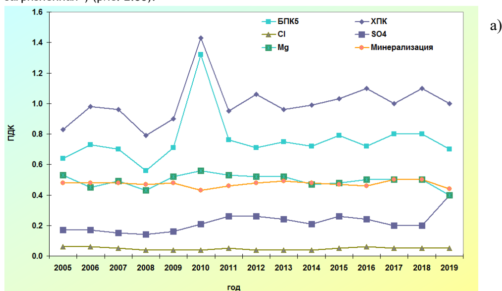
Рис. 2.38 (начало). Изменение среднегодовых концентраций отдельных ингредиентов и качества воды р. Лесной Воронеж выше г. Мичуринск за многолетний период
