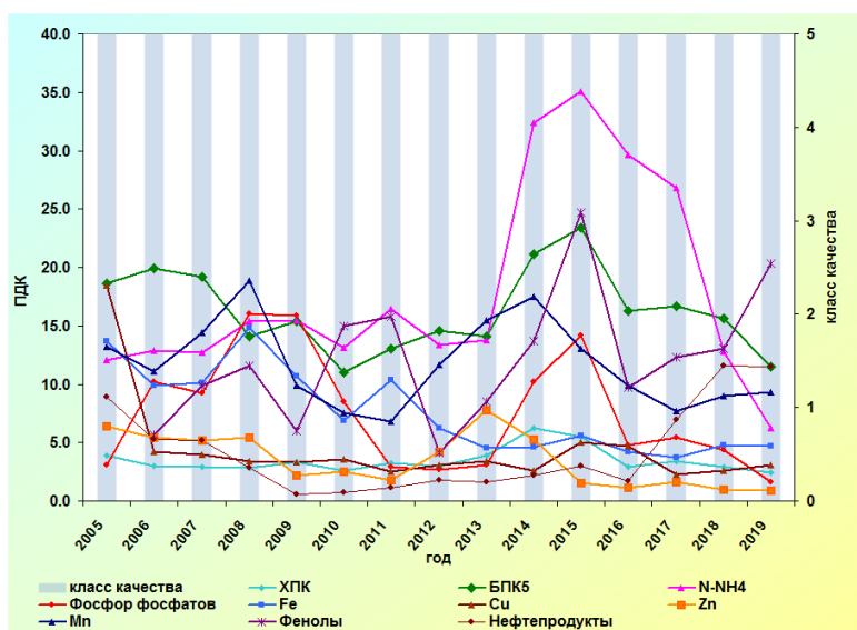
Рис. 3.52. Изменение среднегодовых концентраций отдельных ингредиентов и качества воды р. Дачная, в черте г. Арсеньев за многолетний период
