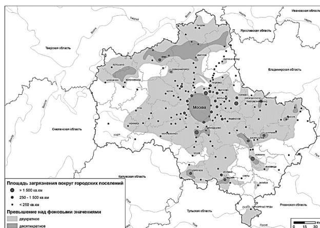
Рис. 4.5. Загрязненность почв Московского региона
