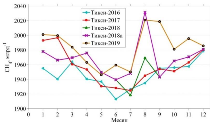
Рис. 2.2. Сезонный ход концентрации \text{CH}_4 на станции Тикси
