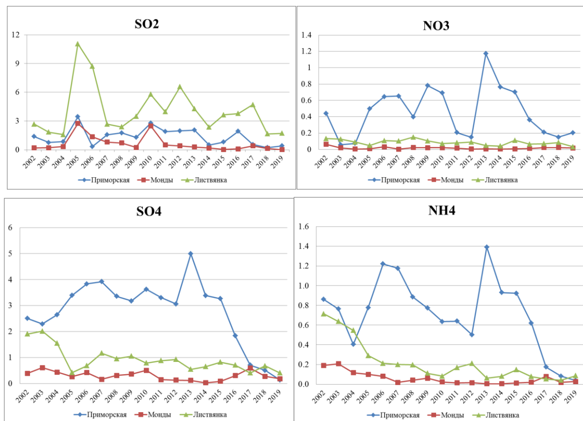
Рис. 2.32. Изменения средних годовых концентрации соединений серы (слева) и азота (справа) в воздухе на станциях ЕАНЕТ ( \text{мкг/м}^3 )
