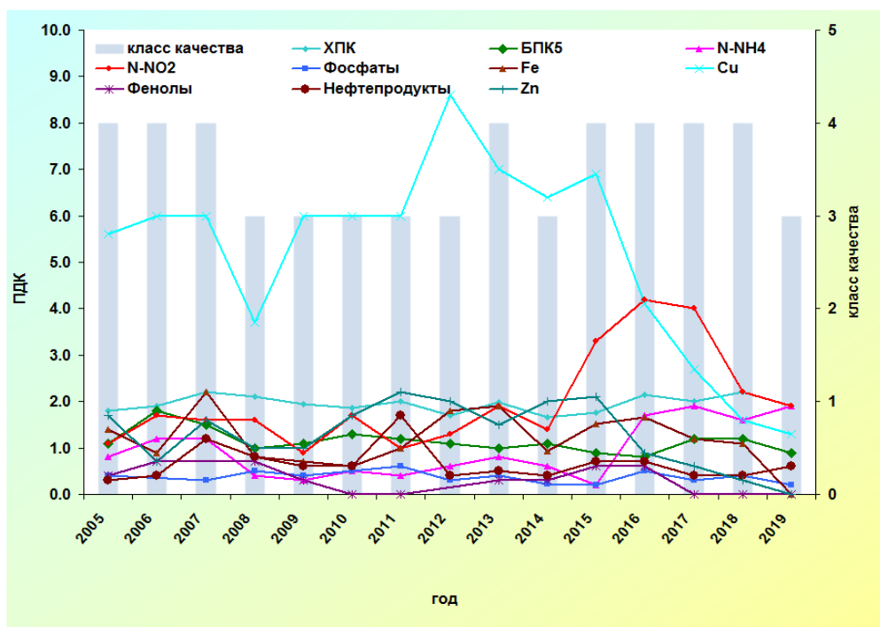
Рис. 3.37. Изменение среднегодовых концентраций отдельных ингредиентов и качества воды Чебоксарского водохранилища, 4,2 км ниже г. Нижний Новгород за многолетний период
