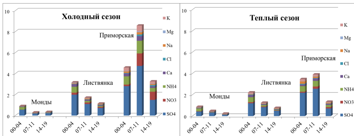
Рис. 2.31. Изменения среднего химического состава аэрозолей ( \text{мкг/м}^3 ) на станциях ЕАНЕТ в холодный (слева) и теплый (справа) сезоны по наблюдениям в 2000-2019 гг.
