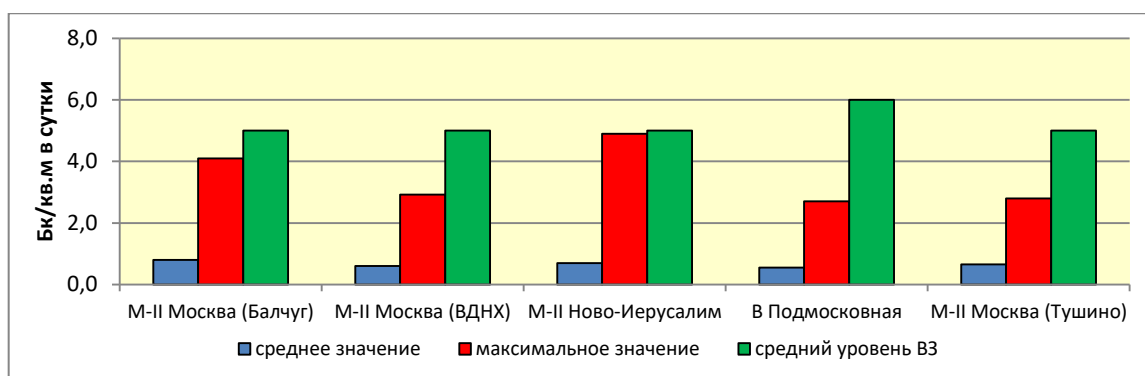
Рис. 4.13. Среднемесячные и максимальные суточные выпадения на станциях Московского региона в 2019 г.
