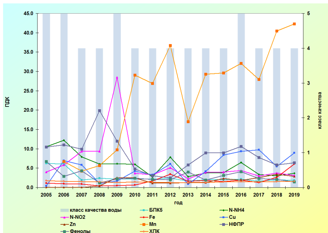
Рис. 3.47. Изменение среднегодовых концентраций отдельных ингредиентов и качества воды р. Каменка за многолетний период
