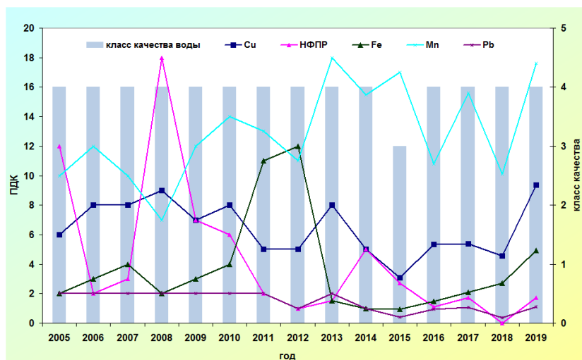
Рис. 3.50. Изменение среднегодовых концентраций отдельных ингредиентов и качества воды р. Колыма, п. Усть-Среднекан за многолетний период
