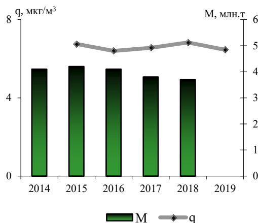
Рис. 3.10. Среднегодовые концентрации (q, мкг/м³) и суммарные выбросы (M, млн. т) диоксида серы
