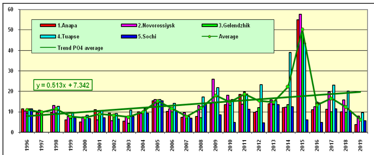
Рис. 3.65. Динамика средней концентрации фосфатов P-PO 4 ( \text{мг/дм}^3 ) в прибрежных водах Кавказа в 1996-2019 гг. Сокращения: Average - средняя концентрация фосфатов; Trend PO 4 average - тренд средней концентрации фосфатов.
