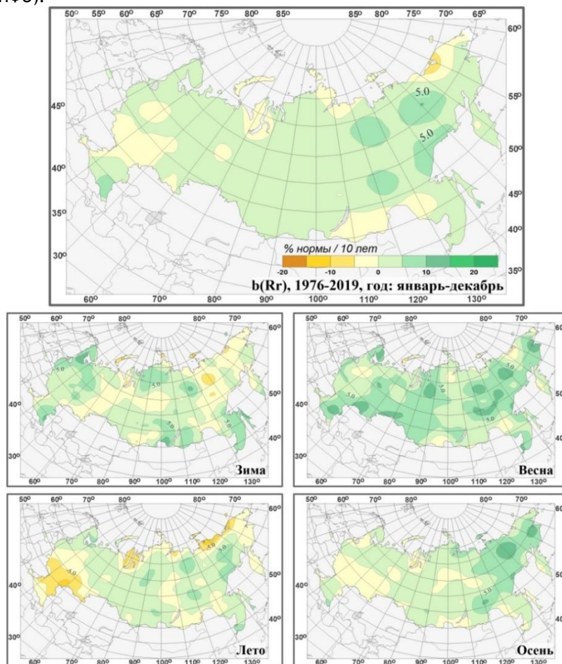
Рис. 1.13. Пространственные распределения локальных коэффициентов линейного тренда годовых и сезонных сумм атмосферных осадков за 1976-2019 гг. на территории России (% от нормы за 10 лет)
