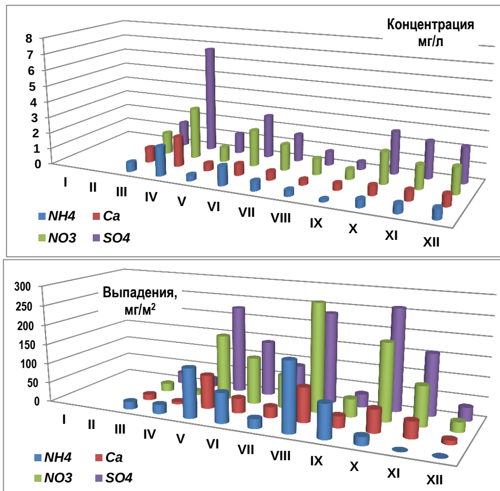
Рис. 2.33. Годовой ход концентраций (верхний) и выпадений (нижний) основных кислотообразующих ионов с осадками в районе станции Приморская (юг Дальнего Востока) в 2019 г.
