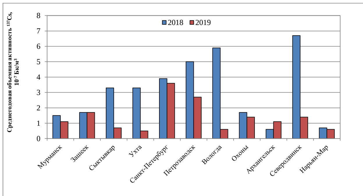
Рис. 2.45. Среднегодовая объемная активность ^{137}\text{Cs} в населенных пунктах СЗФО
