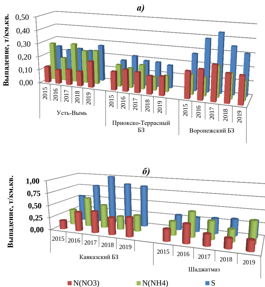
Рис. 2.19. Выпадения серы (S), азота нитратного (N(NO 3 )) и азота аммонийного (N(NH 4 )) с атмосферными осадками на ЕТР в период с 2015 по 2019 гг.
