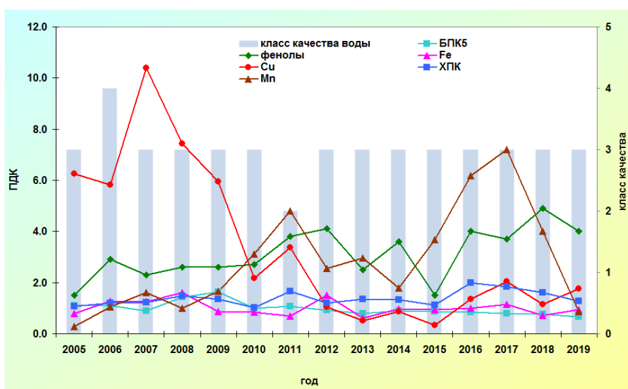
Рис. 3.49. Изменение среднегодовых концентраций отдельных ингредиентов и качества воды р. Лена, г. Якутск за многолетний период
