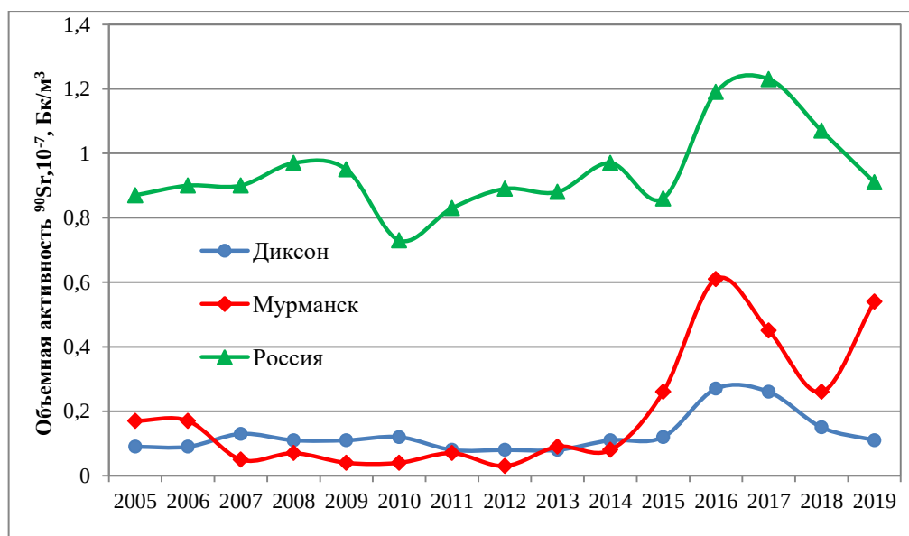
Рис. 4.58. Динамика объемной активности ^{90}\text{Sr} в воздухе на о. Диксоне, в Мурманске и средневзвешенной по России в 2005-2019 гг.
