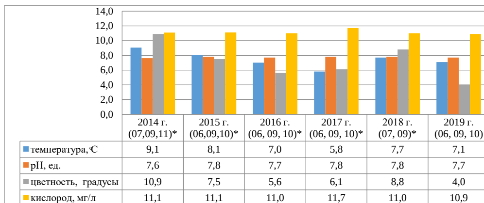
Рис. 4.20. Общая гидрохимическая характеристика воды в районе продольного разреза оз. Байкал (*-месяц отбора проб)
