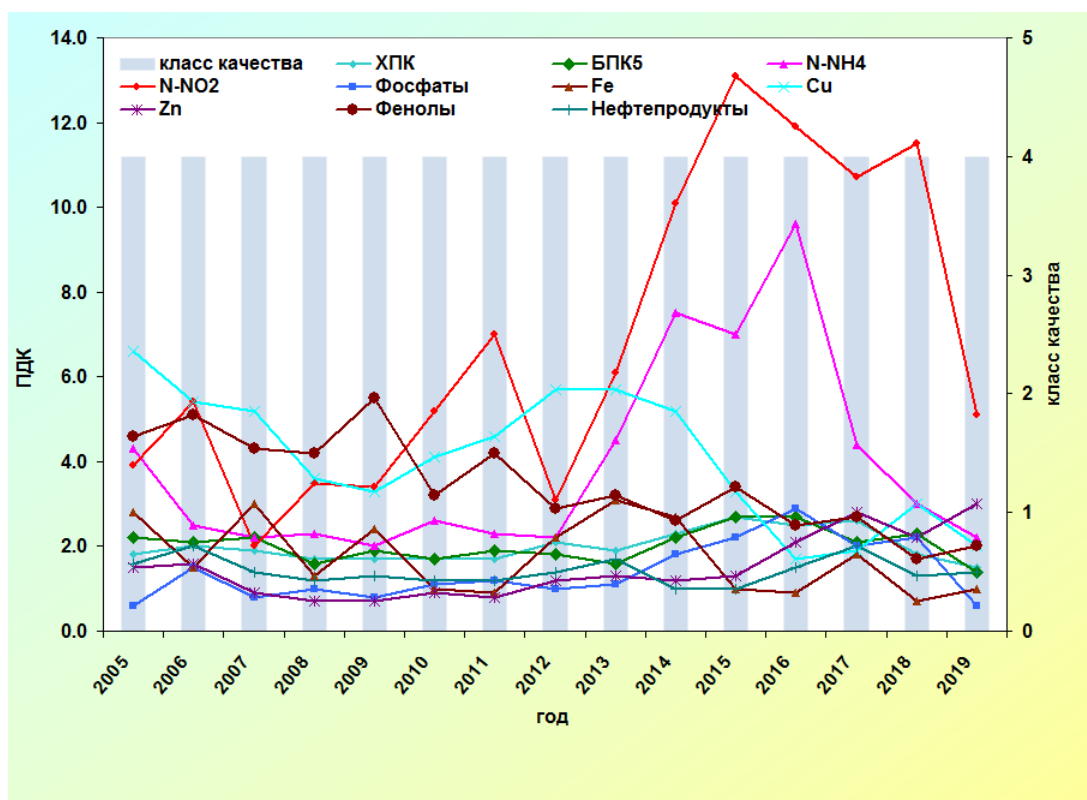
Рис. 3.39. Изменение среднегодовых концентраций отдельных ингредиентов и качества воды р. Ока ниже г. Коломна за многолетний период
