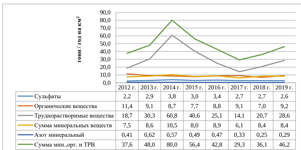
Рис. 4.17. Динамика поступления химических веществ из атмосферы на ст. Исток Ангары
