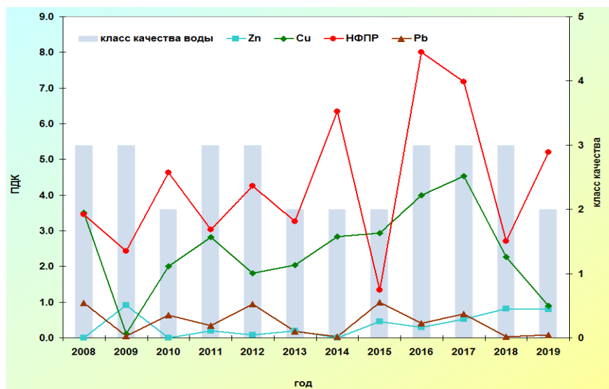
Рис. 2.43. Изменение среднегодовых концентраций отдельных ингредиентов и качества воды р. Берш в пункте с. Пушино за многолетний период
