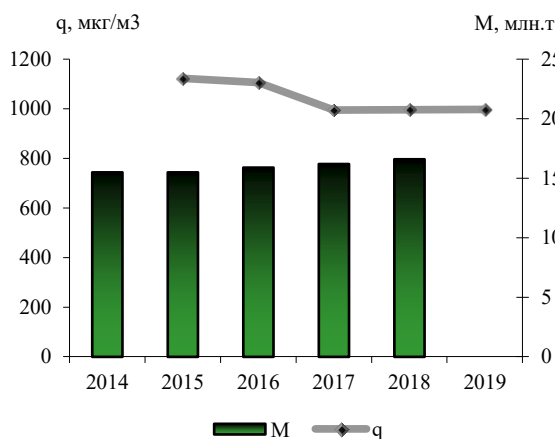
Рис. 3.11. Среднегодовые концентрации ( q , мкг/м 3 ) и суммарные выбросы ( M , млн. т) оксида углерода
