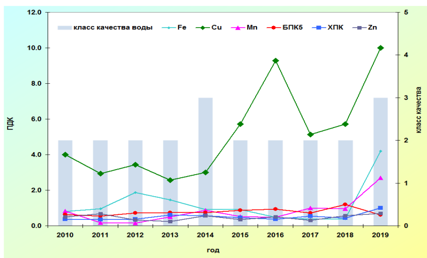
Рис. 2.41. Изменение среднегодовых концентраций отдельных ингредиентов и качества воды р. Рогатка в створе выше г. Южно-Сахалинск за многолетний период
