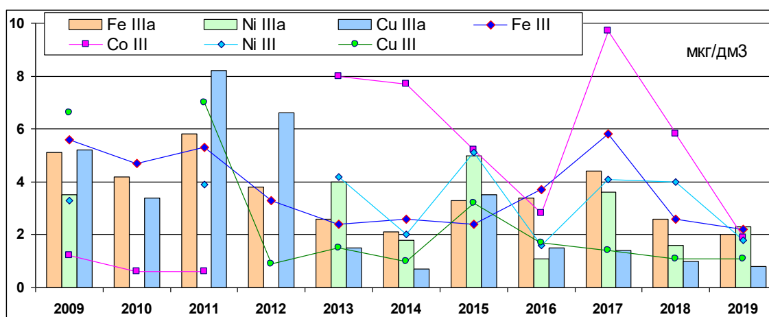
Рис. 3.59. Многолетняя динамика средней годовой концентрации железа (Fe), никеля (Ni) и меди (Cu) на разрезах III (Sec III) и IIIa (Sec IIIa).
