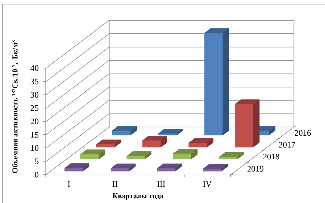
Рис. 4.57. Динамика средней за квартал величины объемной активности ^{137}\text{Cs} в воздухе в Мурманске в 2016-2019 гг.
