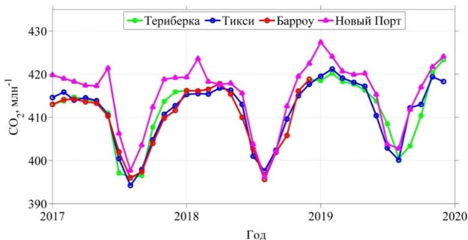
Рис. 4.36. Концентрация \text{CO}_2 для арктических станций РФ в сравнении со станцией Барроу
