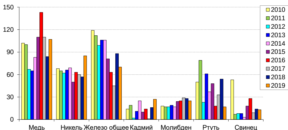
Рис. 3.58. Динамика количества случаев ВЗ и ЭВЗ поверхностных пресных вод некоторыми тяжелыми металлами на территории Российской Федерации
