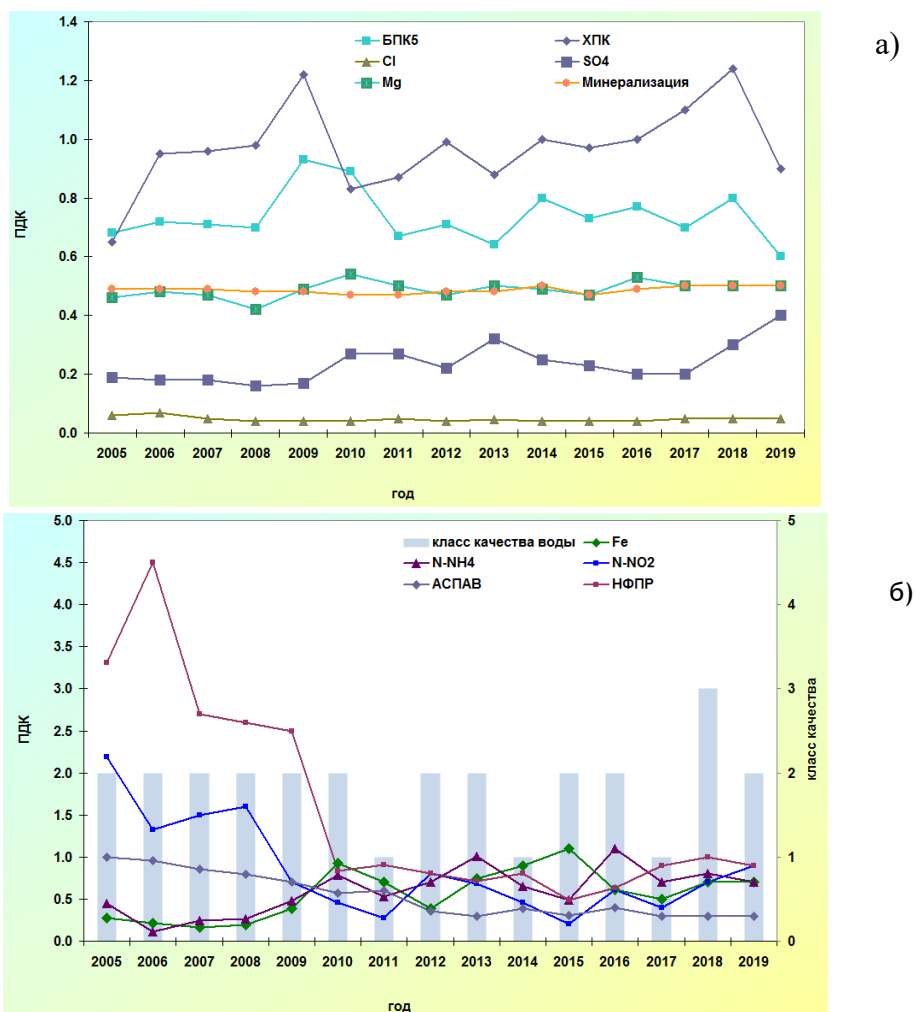
Рис. 2.37. Изменение среднегодовых концентраций отдельных ингредиентов и качества воды р. Ворона в черте г. Уварово за многолетний период
