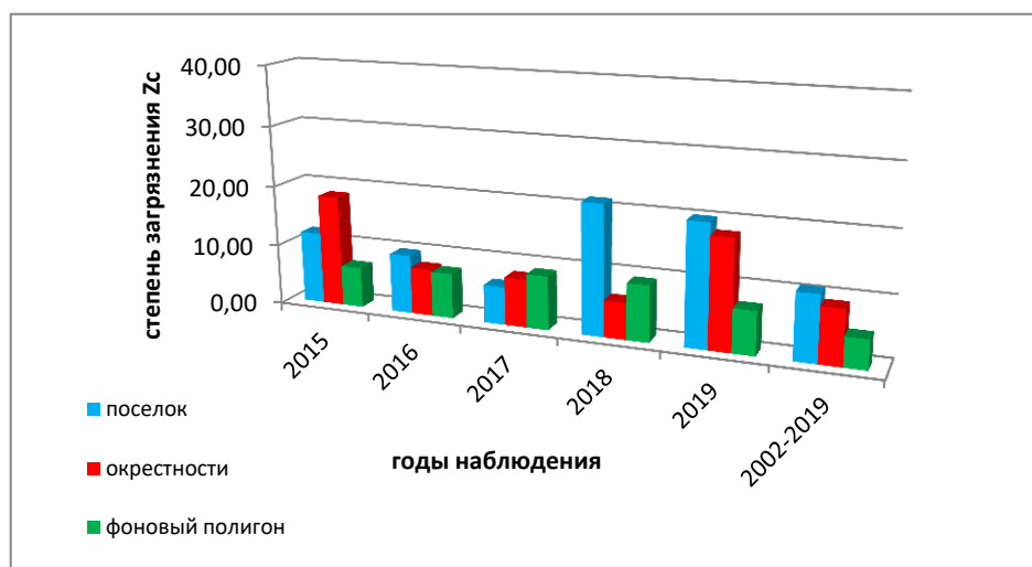
Рис. 4.63. Межгодовая изменчивость суммарного показателя химического загрязнения Z_c в районе пос. Баренцбург, его окрестностях и фоновых территориях в период 2015-2019 гг. и осредненные значения за 2002-2019 гг.
