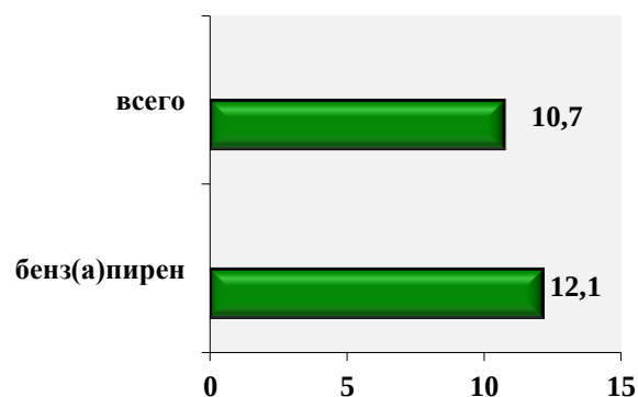
Рис. 3.20. Число жителей в городах (млн.), находящихся под воздействием максимальных концентраций примесей в воздухе выше 10 ПДК (всего) и 5 ПДК бенз(а)пирена
