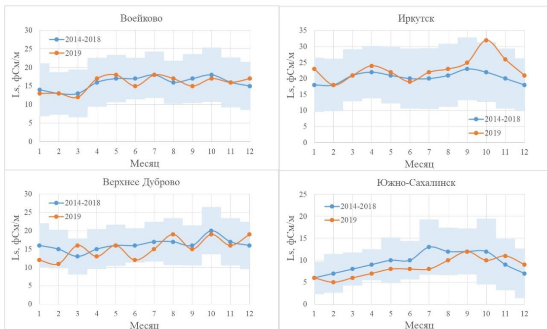
Рис. 2.9. Годовой ход L_5 на станциях Воейково, Иркутск, Верхнее Дуброво и Южно-Сахалинск в 2019 г. на фоне осредненного годового хода L_5 за период 2014-2018 гг. Цветным фоном обозначены границы стандартного отклонения \pm\sigma от среднего значения за 2014-2018 гг.
