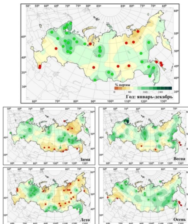
Рис. 1.11. Аномалии годовых и сезонных сумм осадков на территории России в 2019 г. (% от нормы 1961-1990 гг.)
