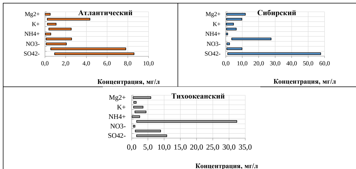
Рис. 4.39. Диапазон изменения средневзвешенных концентраций основных ионов атмосферных осадков Арктической зоны РФ, 2019 г.
