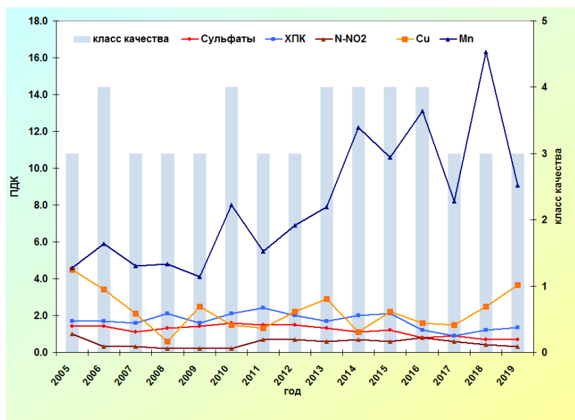
Рис. 3.41. Изменение среднегодовых концентраций отдельных ингредиентов и качества воды Нижнекамского водохранилища в пункте д. Андреевка за многолетний период
