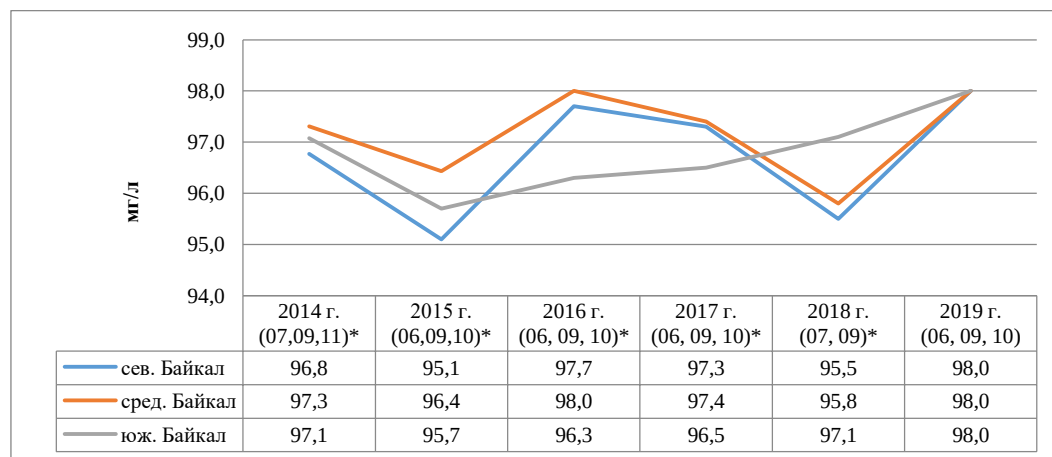
Рис. 4.22. Минерализация воды озера по котловинам продольного разреза (*-месяц отбора проб)
