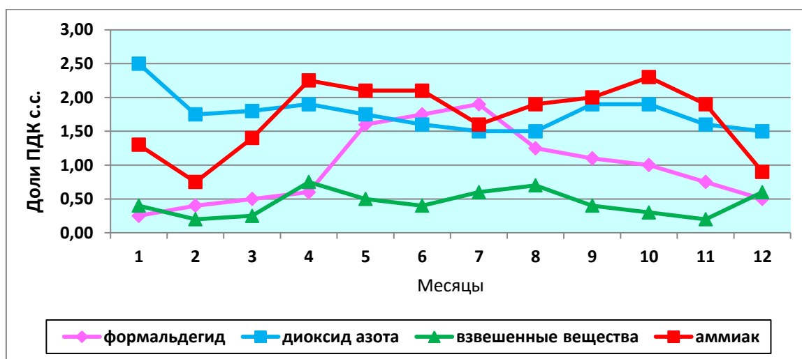
Рис. 4.3. Годовой ход концентраций взвешенных веществ, формальдегида и диоксида азота в атмосферном воздухе г. Москвы в 2019 г.
