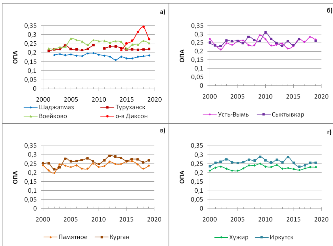
Рис. 2.7. Изменчивость среднегодовых значений ОПА в 2000-2019 гг.
