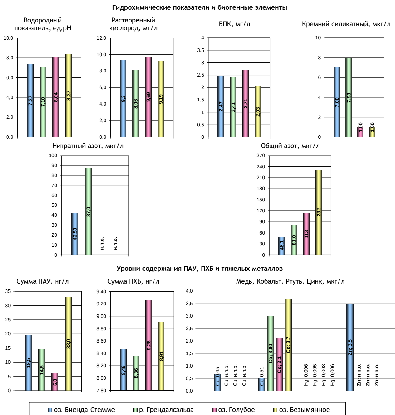
Рис. 4.62. Средние значения основных гидрохимических показателей и загрязняющих веществ поверхностных вод суши в летний период
