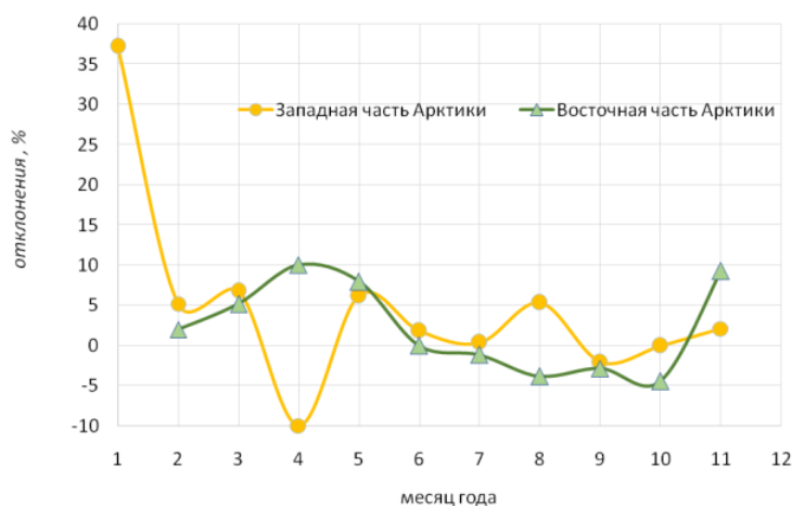
Рис. 4.34. Отклонения среднемесячных значений ОСО от нормы в восточной и западной частях Арктического региона в 2019 г.
