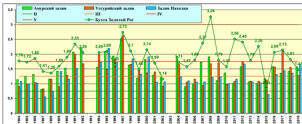
Рис. 3.71. Многолетняя динамика индекса загрязненности вод (ИЗВ) в различных районах залива Петра Великого Японского моря
