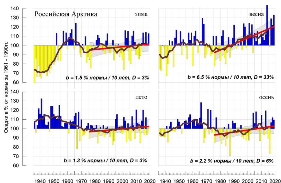
Рис. 4.30. Сезонные суммы осадков (% нормы) в Российской Арктике в 1936-2019 гг. Жирная черная кривая - 11летнее скользящее среднее. Показан линейный тренд за 1976-2019 гг.
