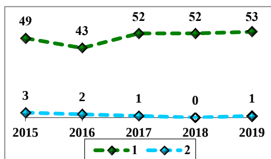
Рис. 3.5. Количество городов, в которых среднегодовые концентрации взвешенных веществ превысили 1 ПДК (1), СИ взвешенных веществ больше 10 (2)
