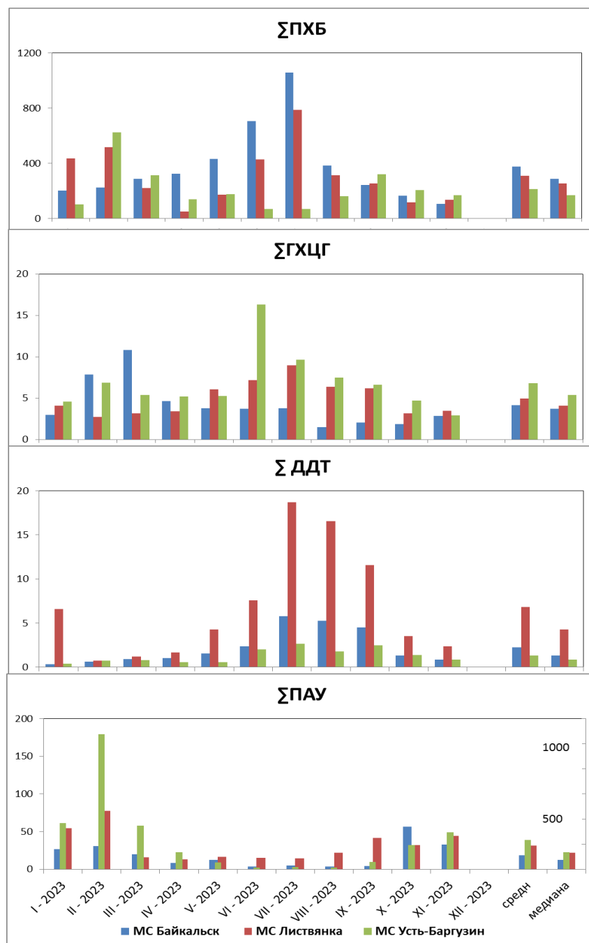
Рис. 4.15. Ход приземных концентраций ΣПХБ, ΣГХЦГ, ΣДДТ (нг/м 3 ) и ΣПАУ (нг/м 3 ) в атмосферном воздухе в 2023 г.
