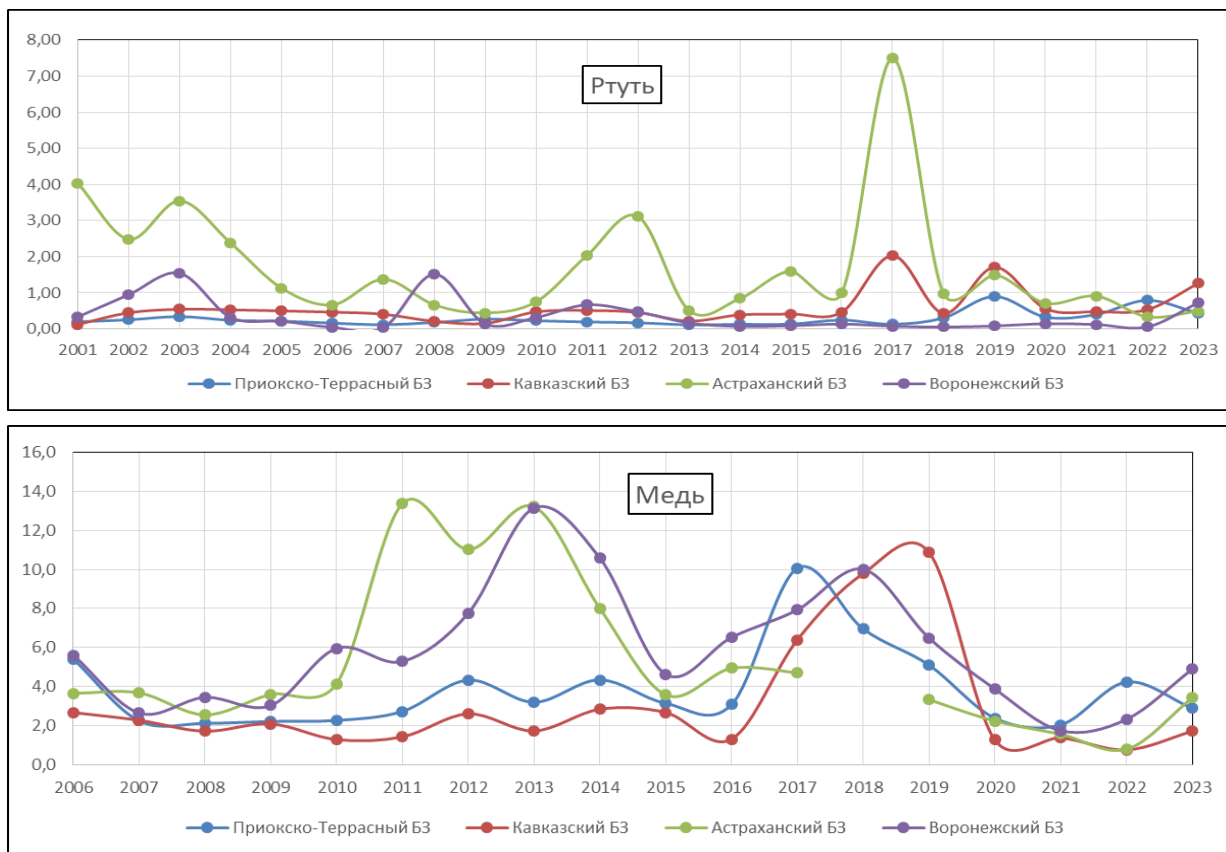
Рис. 2.34 (окончание). Изменение среднего содержания тяжелых металлов (мкг/л) в атмосферных осадках на станциях комплексного фонового мониторинга в 2001-2023 гг.
