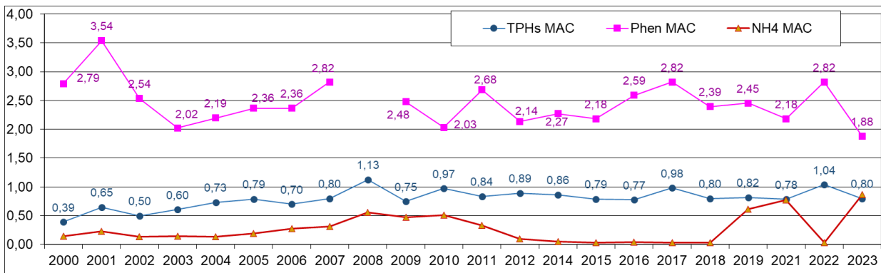
Рис. 3.51. Динамика содержания фенолов (Phen MAC), НУ (TPHs MAC) и аммонийного азота (NH 4 MAC) в ПДК в 2000-2023 гг. на южной границе Северного Каспия (разрез IV) в 2000-2023 гг. MAC - предельно допустимая концентрация (ПДК).
