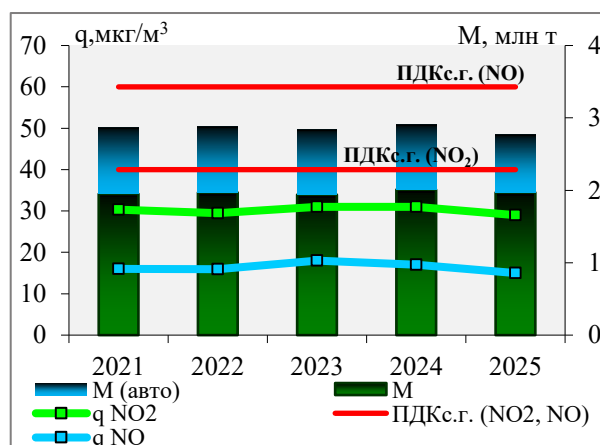
Рис. 3.12. Среднегодовые концентрации диоксида азота (qNO 2 , мкг/м³) и оксида азота (qNO, мкг/м³) и выбросы от стационарных источников (M, млн т) и автотранспорта (M, млн т) NO x (в пересчете на NO 2 )
