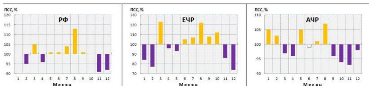
Рисунок 12.4 – Относительные аномалии суммарной за месяц продолжительности солнечного сияния, усредненной по территории РФ, ЕЧР и АЧР; 2024 год
