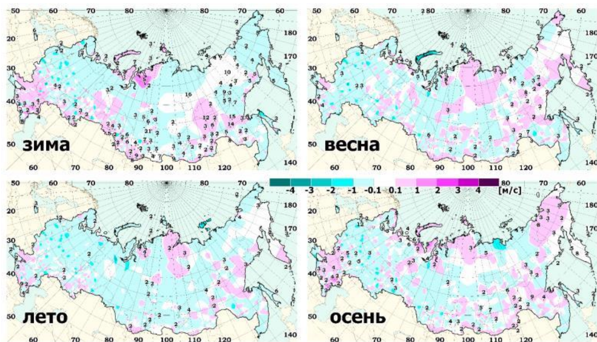
Рисунок 14.2 – Аномалии средней скорости ветра по календарным сезонам 2024 года. Точки и цифрами обозначены станции, на которых скорость ветра превышала 95-й процентиль и число дней с такой экстремальной скоростью ветра
