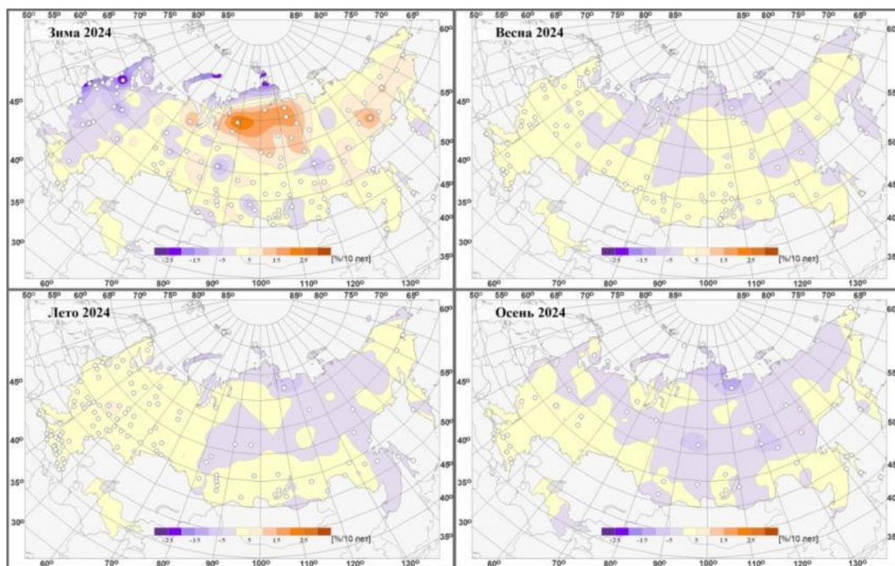
Рисунок 12.6 – Сммотри рисунок 12.5, но для коэффициентов линейного тренда относительных аномалий сезонной продолжительности солнечного сияния
