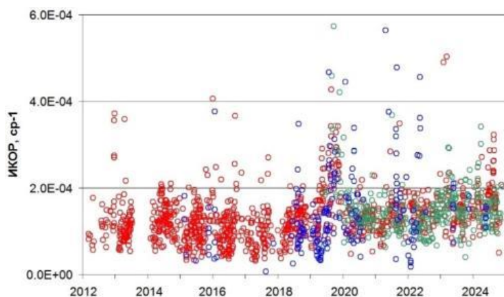
Рисунок 19.1 – ИККОР в слое от 15 до 30 км на лидарных станциях Обнинска, Новосибирска и Знаменска (красные, синие и зеленые кружки)
