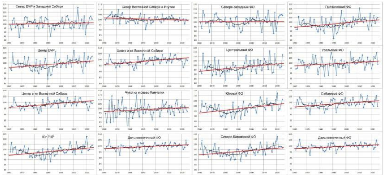
Рисунок 12.8 – Относительные аномалии (%) суммарной за год продолжительности солнечного сияния, осредненной по квази-однородным физико-географическим регионам и федеральным округам РФ
