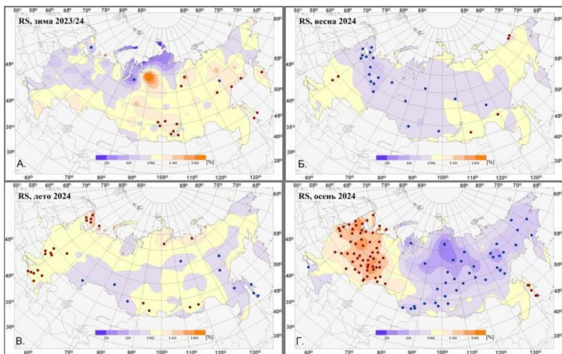
Рисунок 12.2 – Пространственное распределение относительных аномалий сезонной продолжительности солнечного сияния ( RS , %) на территории РФ в 2024 году. Кружками синего цвета показано местоположение станций с экстремумами ниже 5-го перцентиля, коричневого цвета – выше 95-го перцентиля
