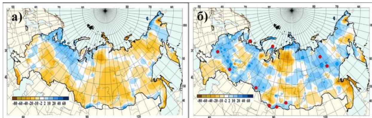
Рисунок 3.2 – а) Аномалии числа дней с покрытием снегом более 50 % территории вокруг метеостанции зимой 2023-2024гг. (от среднемноголетних значений за период 1991-2020 гг.); б) Аномалии максимальной высоты снежного покрова зимой 2023-2024 гг. (от средних многолетних значений за период 1991-2020 гг.). Кружками красного цвета показаны станции, на которых зарегистрирован абсолютный максимум высоты снежного покрова
