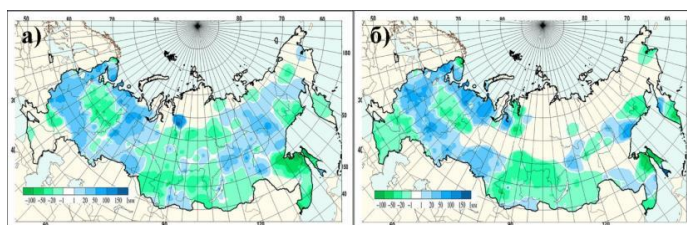
Рисунок 3.3 – Аномалии максимального запаса воды в снеге (мм) зимой 2020-2024 гг. (от среднееголетних значений за период 1971-2000 гг.) в поле (а) и в лесу (б)
