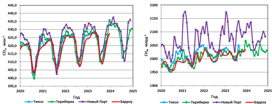
Рисунок 16.1 – Временной ход концентрации \text{CO}_2 и \text{CH}_4 на российских арктических станциях в сравнении с данными станции Барроу (НУОА, США)
