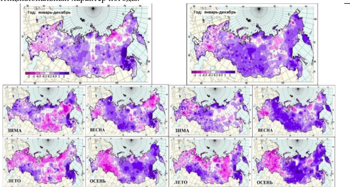
Рисунок 20.1 - Аномалии среднегодового и сезонного балла общей (слева) и нижней (справа) облачности на территории России в 2024 году
