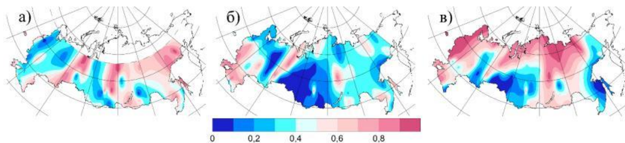
Рисунок 10.4 – Вероятности непревышения сезонных сумм суммарной солнечной радиации зимой 2023-2024 гг. (а), весной 2024 года (б) и летом 2024 года (в)
