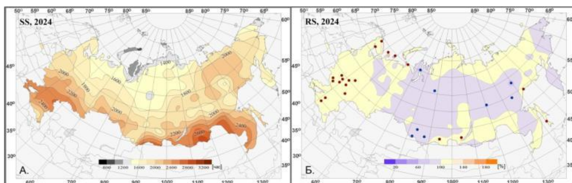
Рисунок 12.1 – Пространственное распределение суммарной за год продолжительности солнечного сияния ( SS , часы) и ее относительных аномалий ( RS , %) на территории РФ в 2024 году. Кружками синего цвета показано местоположение станций с экстремумами ниже 5-го перцентиля, коричневого цвета – выше 95-го перцентиля
