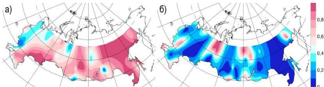
Рисунок 10.3 — Вероятности непревышения сезонных сумм прямой солнечной (а) и рассеянной (б) радиации. Зима 2023-2024 гг.
