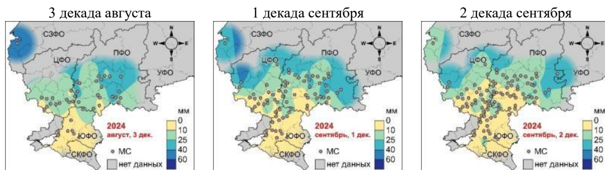
Рисунок 8.5 – Запасы продуктивной влаги в пахотном слое почвы под озимой пшеницей на третью декаду августа, первую и вторую декады сентября 2024 года (по данным наблюдений)
