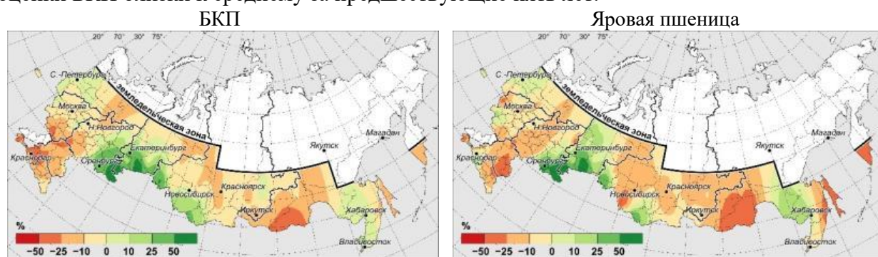
Рисунок 8.4 – Отклонения (%) значений биоклиматического потенциала и климатически обусловленной урожайности яровой пшеницы за 2024 год относительно средних за 2019-2023 гг. Расчёты выполнены в имитационной системе Климат-Почва-Урожай
