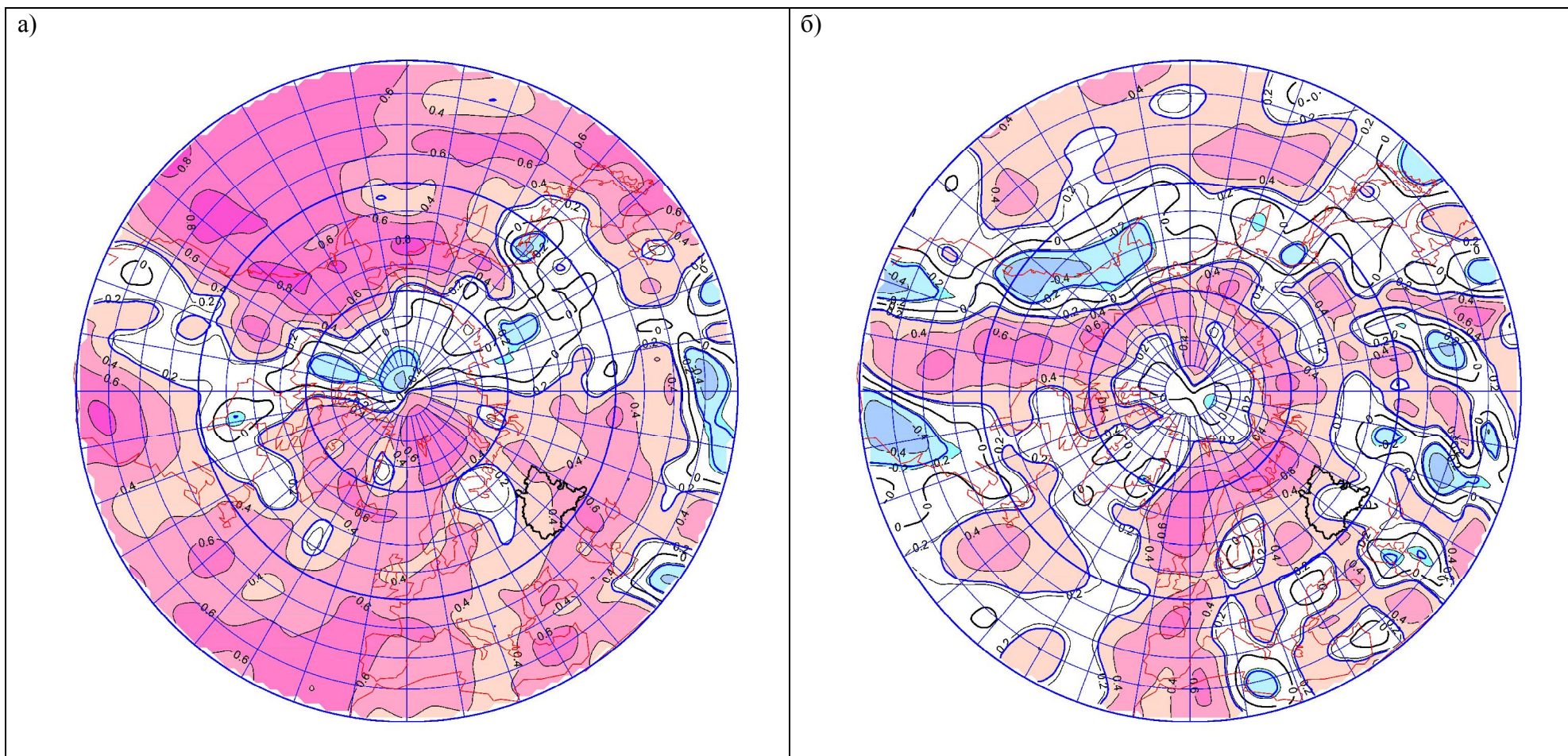
Рис.16. Коэффициенты частной корреляции приземной температуры воздуха и меридиональной компоненты скорости ветра на изобарической поверхности 850 гПа зимой (слева) и летом (справа).
