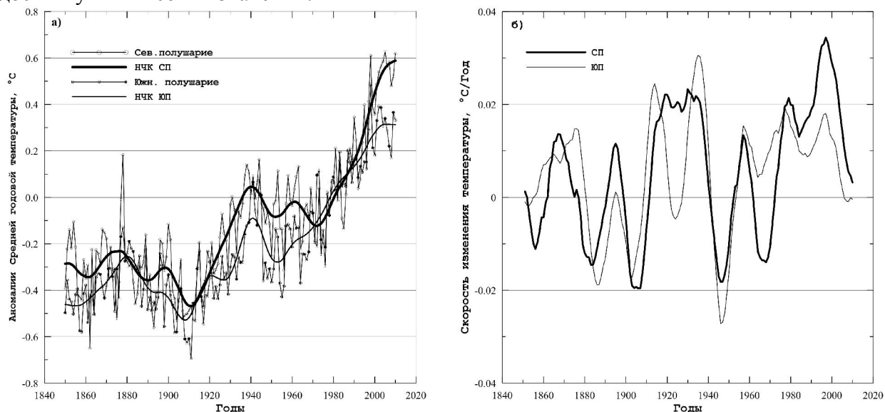
Рис. 1.2. (а) Многолетний ход средней годовой приземной температуры воздуха ( ^{\circ}\text{C} ) северного (вверху) и южного (внизу) полушария ( ^{\circ}\text{C} ), сглаженный НЧ фильтром Поттера (полоса пропускания 10 лет и более). (б) Многолетний ход интенсивности изменения ( ^{\circ}\text{C}/\text{год} ) средней годовой приземной температуры воздуха северного и южного полушария, сглаженный НЧ фильтром Поттера (полоса пропускания 10 лет и более).
