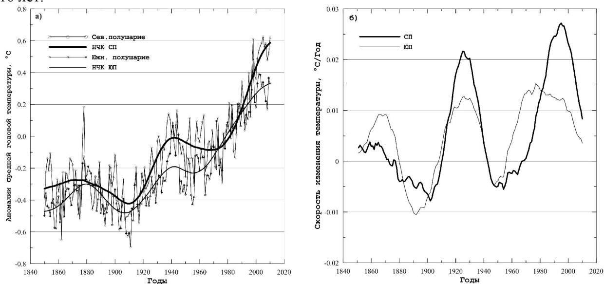
Рис.1.1. (а) Многолетний ход средней годовой приземной температуры воздуха ( ^{\circ}\text{C} ) северного (вверху) и южного (внизу) полушарий и ее долгопериодной компоненты (30 лет и более); (б) Многолетний ход интенсивности изменения ( ^{\circ}\text{C}/\text{год} ) долгопериодной компоненты (30 лет и более) температуры северного и южного полушарий.
