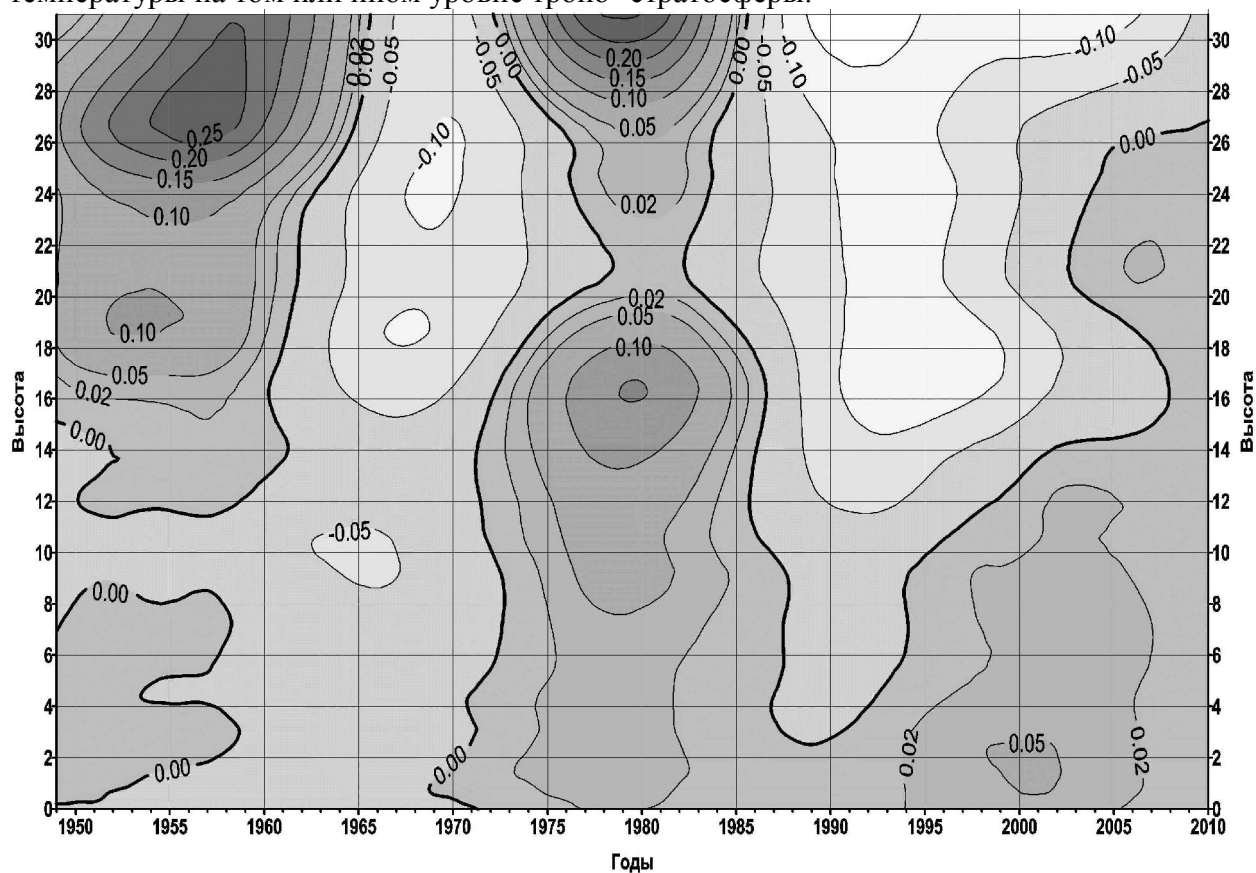
Рис. 1.4. Временной вертикальный разрез осредненных по территории Северного полушария изменений долгопериодной (10 и более лет) компоненты температуры воздуха ( ^{\circ}\text{C}/\text{год} ) по данным реанализа.
