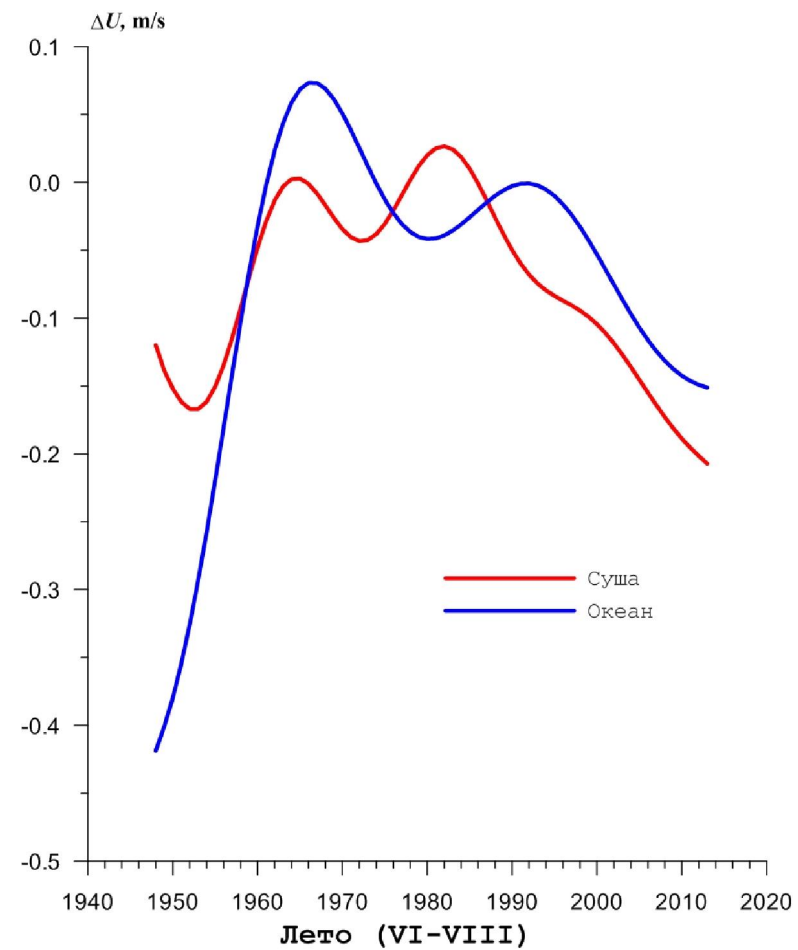
Рис.2.6. НЧК (более 10 лет) аномалий зональной компоненты скорости ветра в умеренной зоне СП над сушей и океаном на изобарической поверхности 500 гПа зимой и летом.
