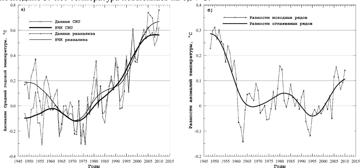
Рис. 1.3. Многолетний ход аномалий средней годовой приземной температуры Северного полушария (а) и разностей аномалий ( ^{\circ}\text{C} ) по данным реанализа и университета Восточной Англии. Сглаженная линия – низкочастотная (10 и более лет) компонента аномалий среднегодовой температуры Северного полушария.
