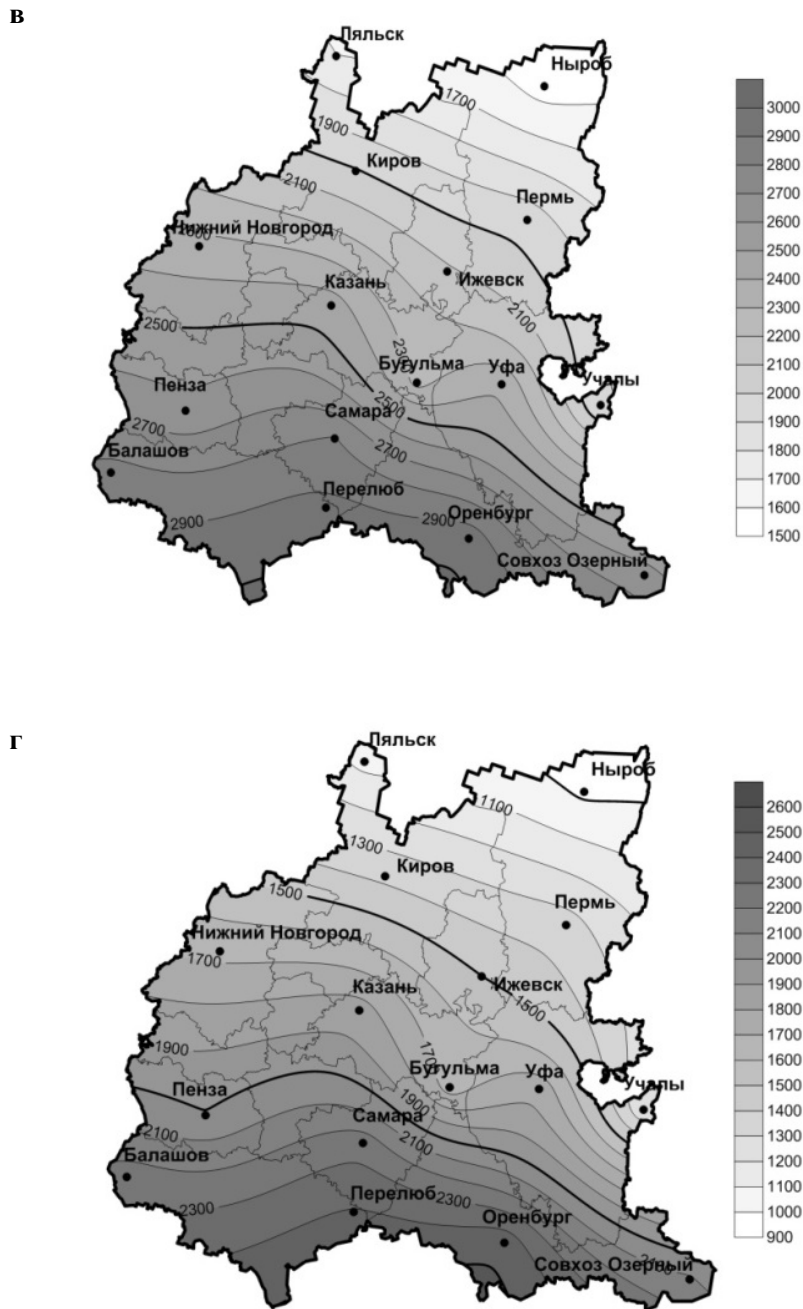
Рисунок 5. Распределение сумм положительных температур для периодов превышения средней суточной температуры пределов 0 (а), 5 (б), 10 (в) и 15 (г) °С
