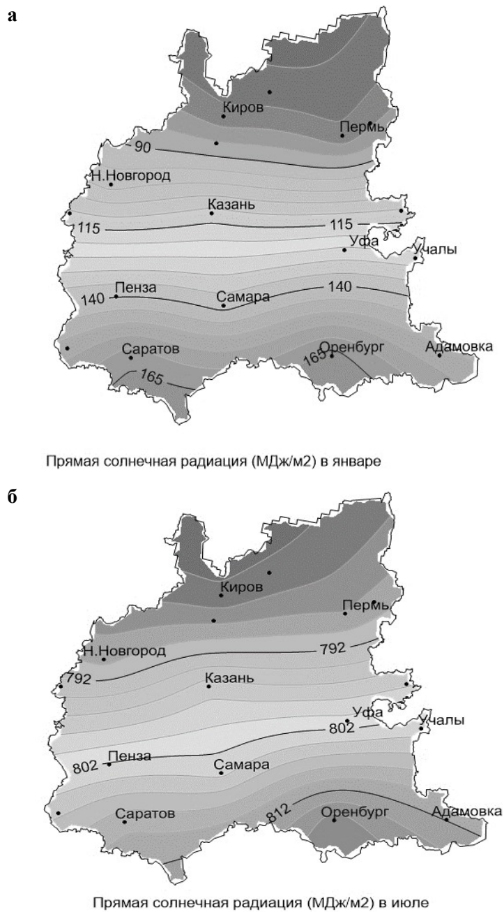
Рисунок 1. Суммы прямой солнечной радиации при ясном небе в январе (а) и июле (б), МДж/м 2
