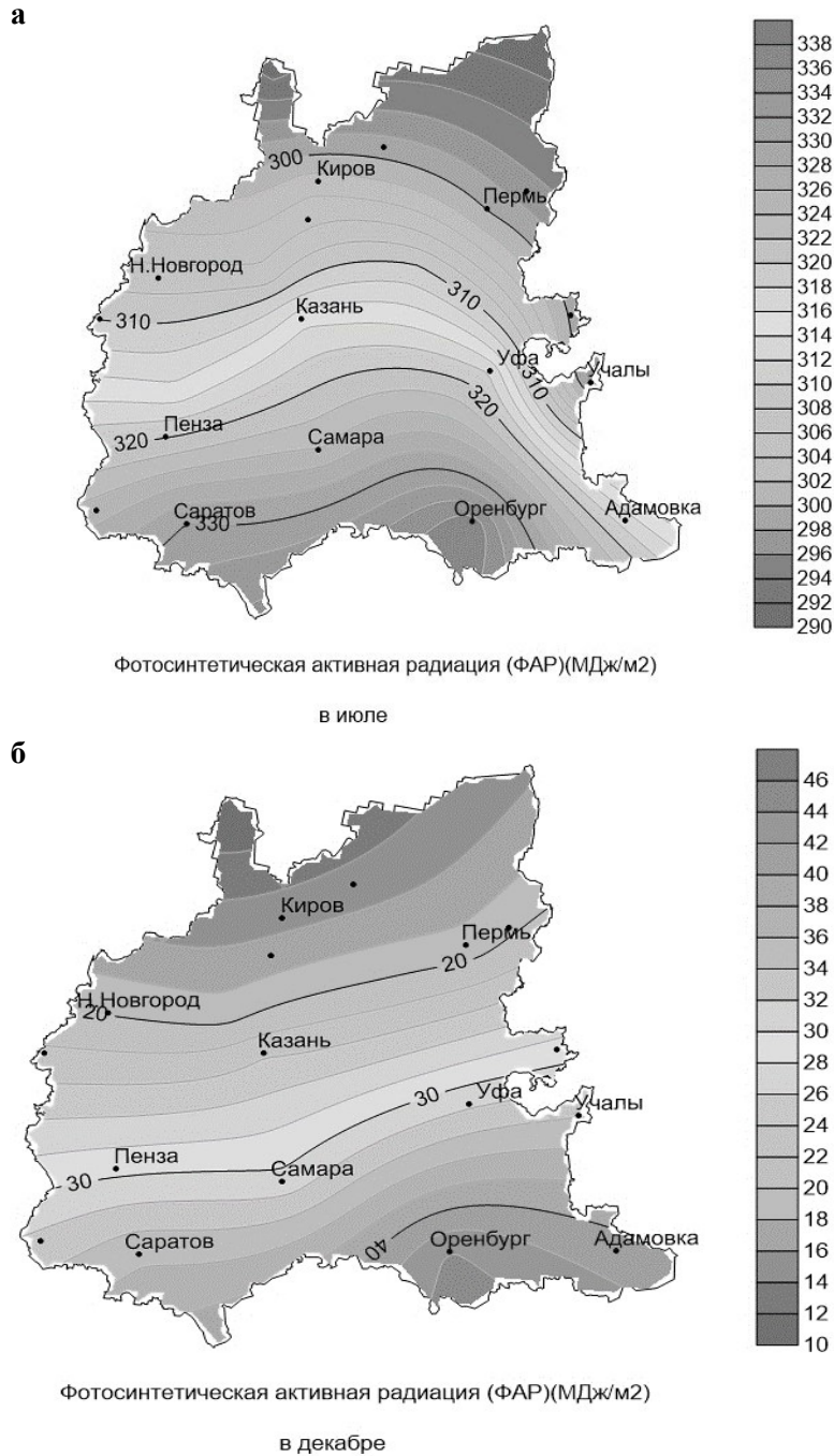
Рисунок 3. Фотосинтетически активная радиация в апреле (а) и в июле (б), МДж/м 2 Figure 3. Photosynthetically active radiation in April (a) and July (b), MJ/m 2
