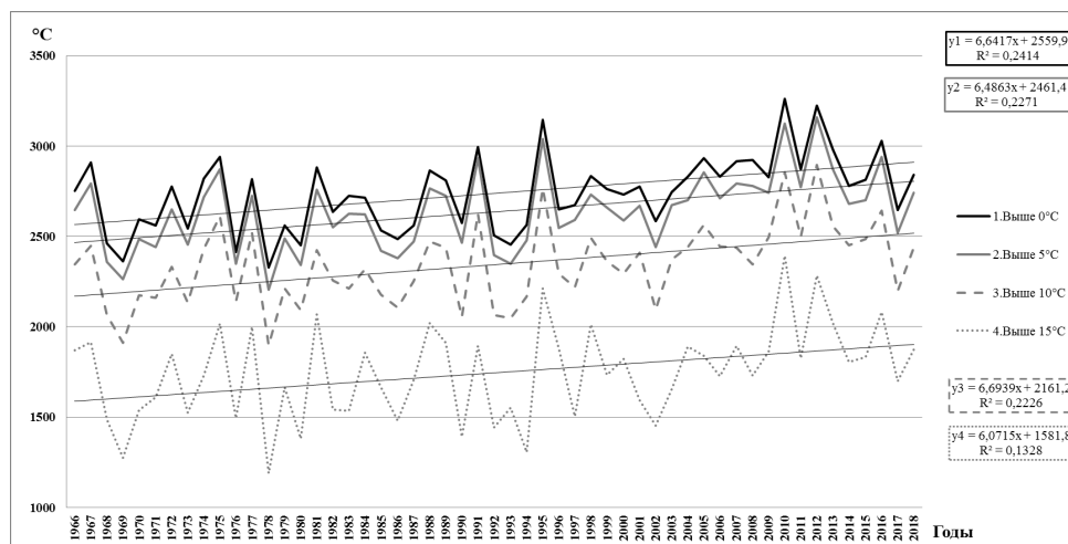
Рисунок 6. Многолетний ход сумм температур выше 0, 5, 10, 15 ^{\circ}\text{C} , осредненных для ПФО (1966-2018 гг.)
