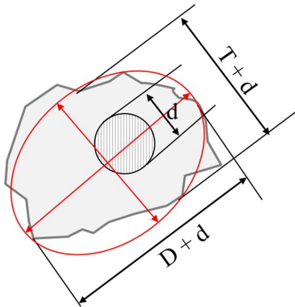
Рисунок 1. Схема гололедно-изморозевого отложения на проводе гололедного станка (Наставление, 1985)
