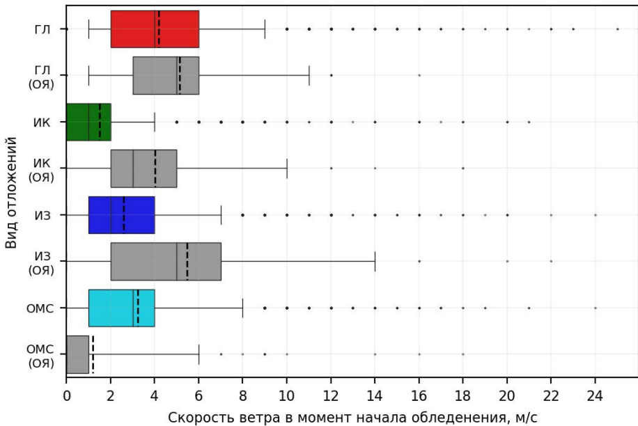
Рисунок 3. Различия наблюдаемой скорости ветра в момент начала обледенения для каждого из видов гололедно-изморозевых отложений
